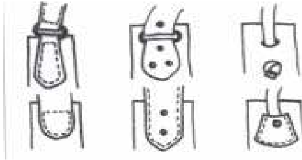
Şekil No:15 Sapı Çantaya Takma Teknikleri
