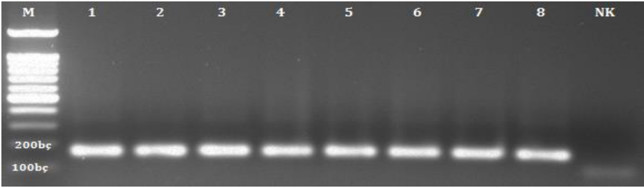
Şekil 4.5. BARII hattında MCW020 lokusu için PCR ürünlerine ait agaroz jel görüntüsü
