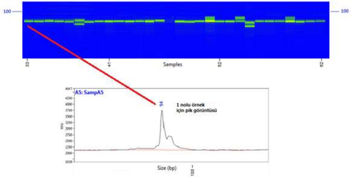
Şekil 4.9. RIRII hattında MCW0123 lokusu için fragment analiz cihazındaki gel ve pik görüntüsü
