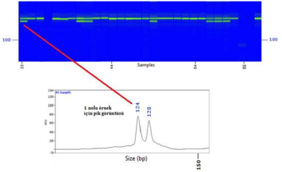
Şekil 4.12. L-54 hattında ADL0112 lokusu için fragment analiz cihazındaki jel ve pik görüntüsü
