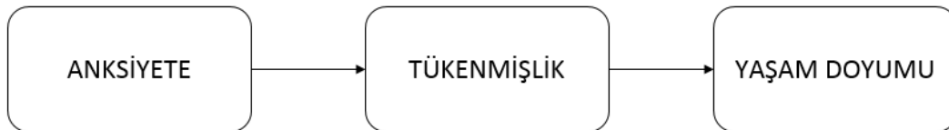
Şekil 2. Sonuç Modeli
