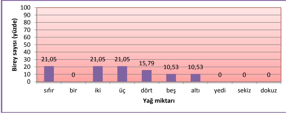
řekil 4.14. Saz kamyřınıının 2011 yılı sonbahar g dnemi yağ miktarı
