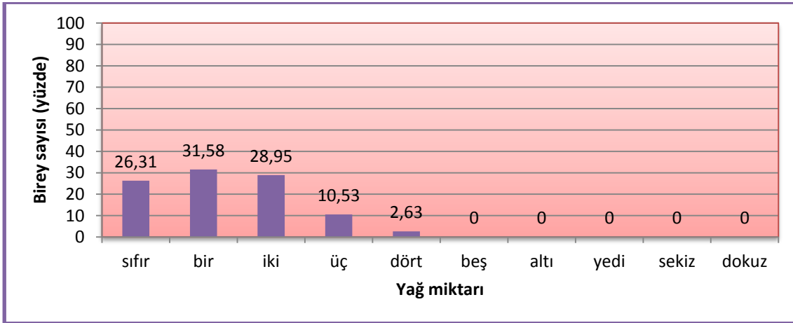
řekil 4.15. Saz kamyřınıının 2012 yılı ilkbahar g dnemi yağ miktarı
