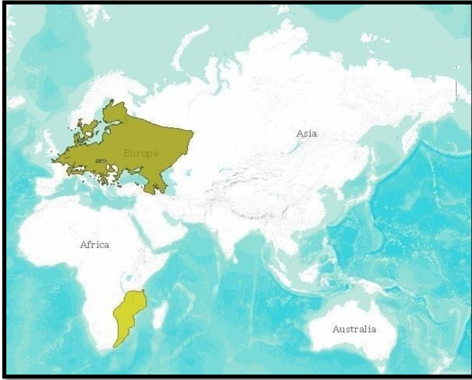
Şekil 2.4. Çalı kamışçınının yayılış haritası (IUCN 2013'den)
