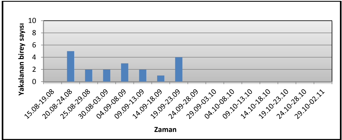
Şekil 4.8. Saz kamyışınının 2011 yılı sonbahar dönemi göç takvimi
