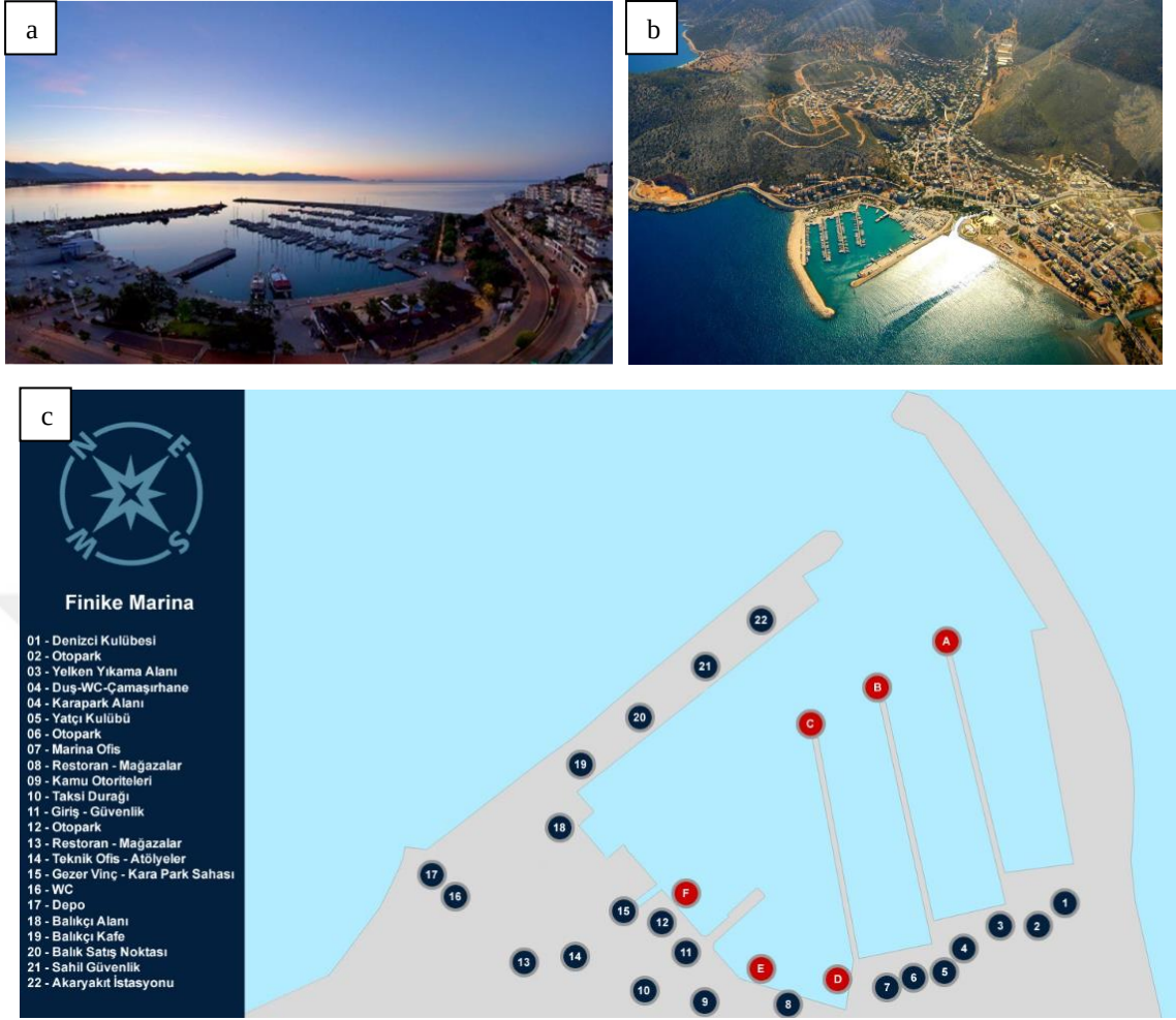
Şekil 4.24. Finike Marina; a) Phonikos tepesinden akşamüstü görüntüsü; b) Hava fotoğrafı (Finike Belediyesi 2022b); c) Yerleşim Planı (Setur Marina 2022)
