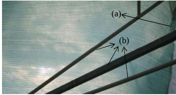
Şekil 4.12. Seraların Soğutulması Amacıyla Çatı İç Yüzeyinde Gölgeleme Perdesinin Kullanıldığı Bir Sera İşletmesi (a) Gölgelemede kullanılan malzeme, (b) çatı kısmındaki yapı elemanları
