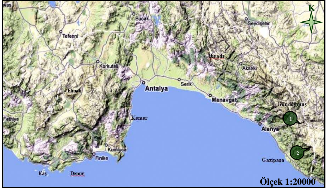
Şekil 3.15. S. erythrantha var. cedretorum 'un örneklendiği lokasyonların haritadaki yeri
