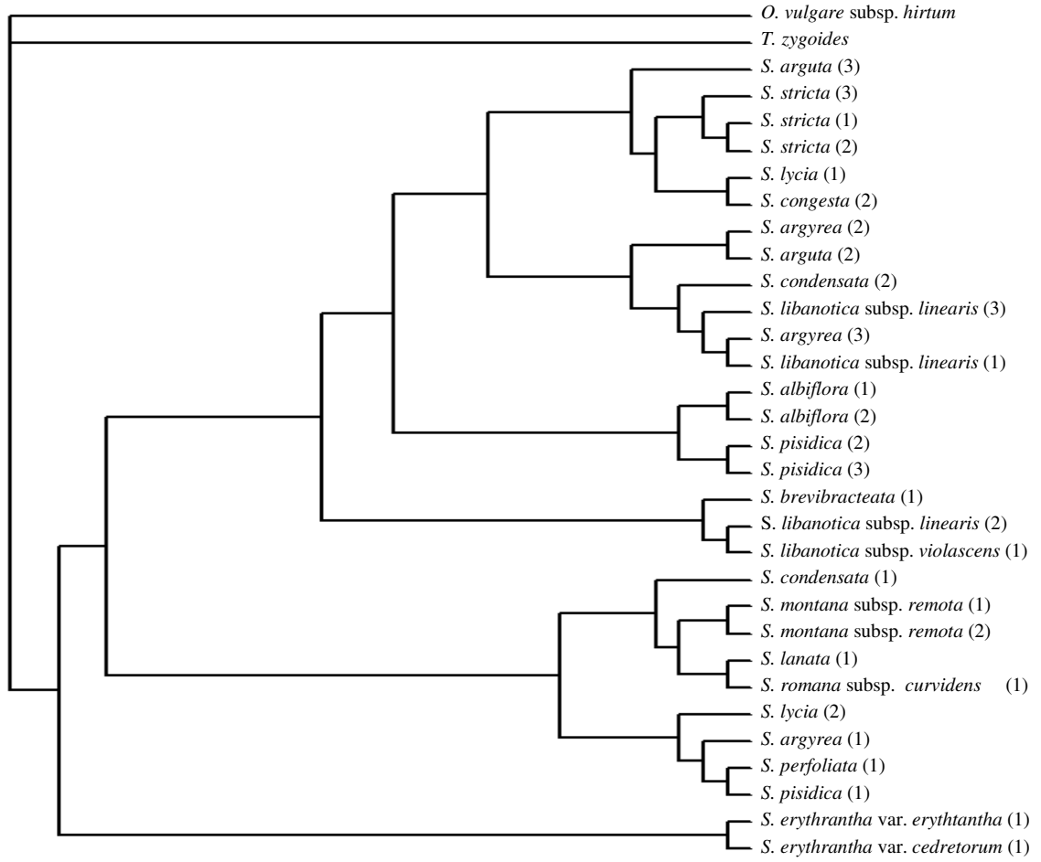
Şekil 4.28. 5.8 S gen bölgesinde neighbor joining analizi sonucu elde edilen dendrogram
