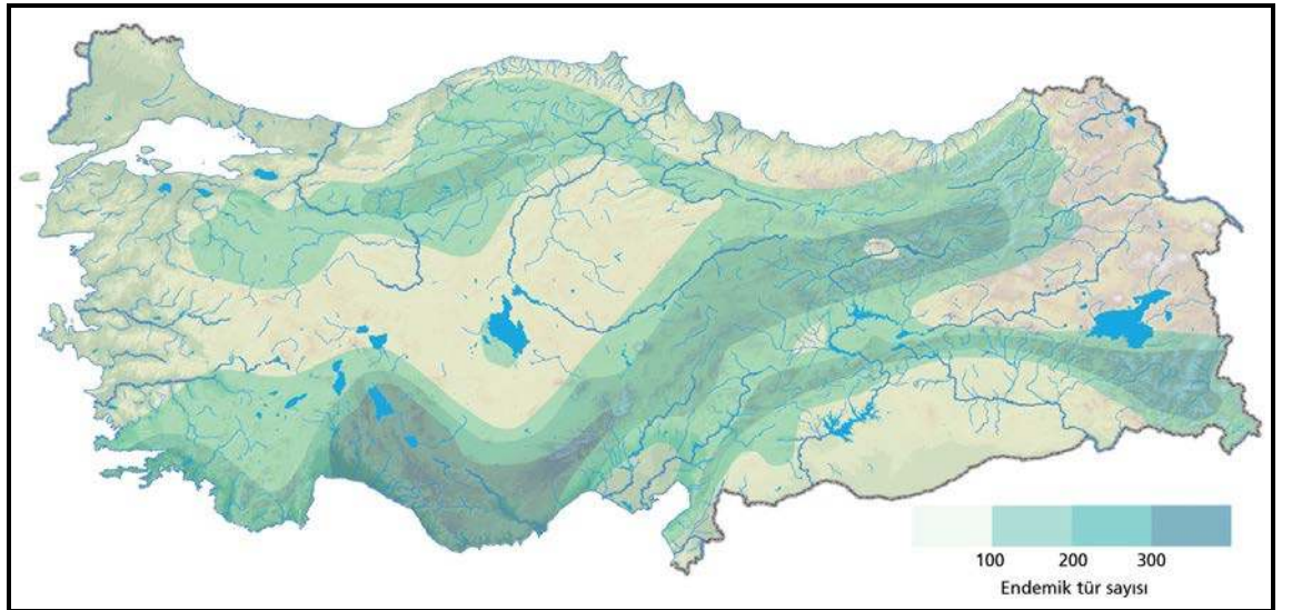
Şekil 1.2. Türkiye endemik tür sayısı haritası, (Eken vd 2006).
