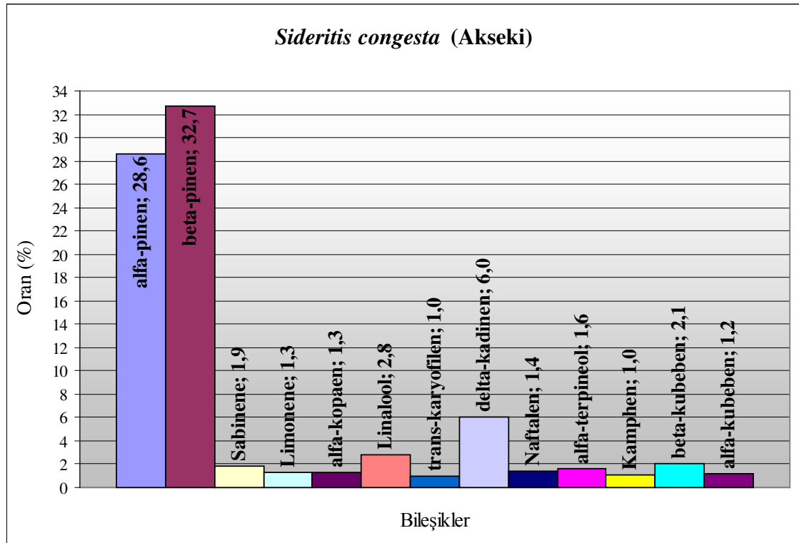
Şekil 4.11. S. congesta türünün uçucu yağ bileşenlerine ait grafik (Akseki)
