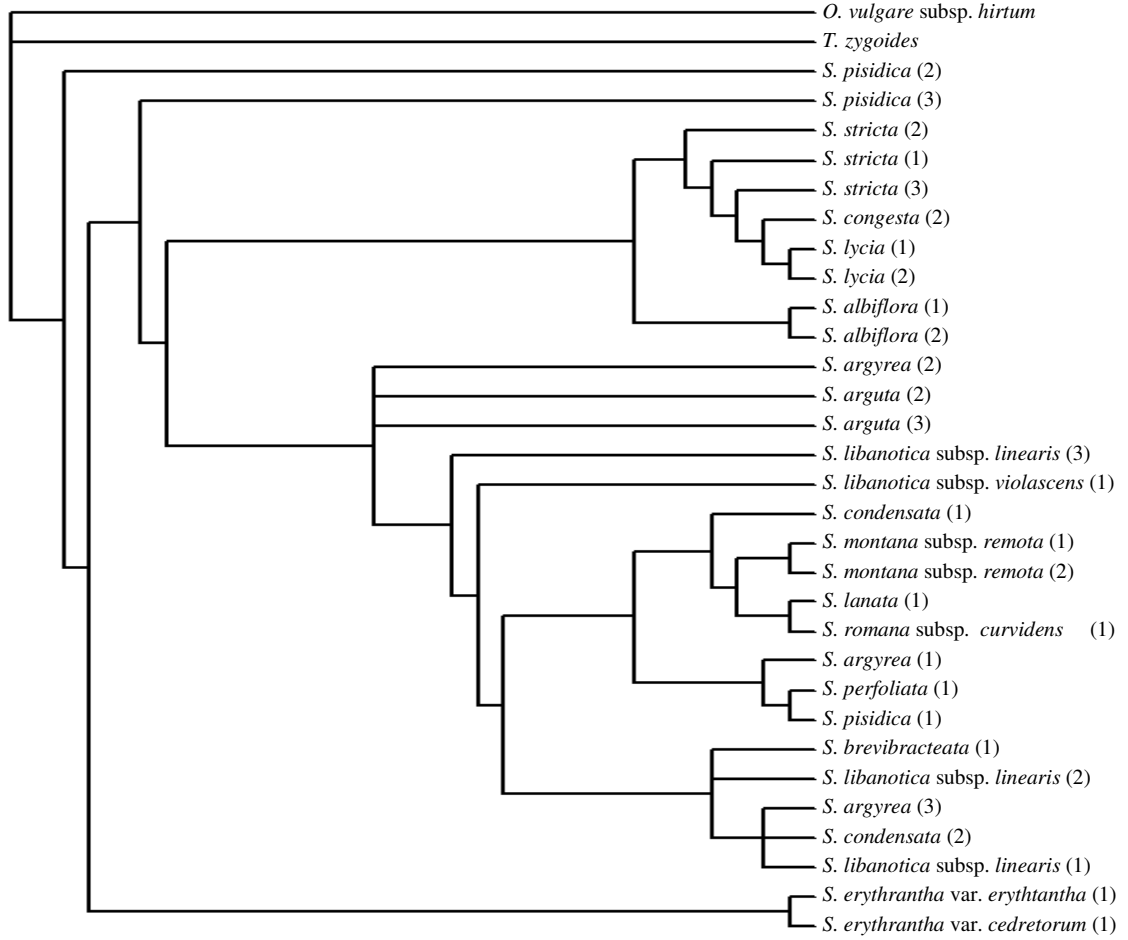
Şekil 4.27. 5.8 S gen bölgesinde maximum likelihood analizi sonucu elde edilen dendrogram
