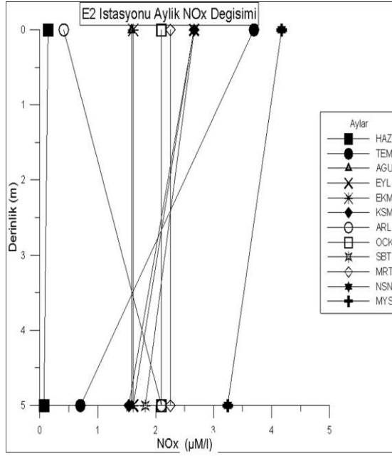
Şekil 4.108. E2 istasyonunda derinliğe bağlı aylık NOx değişimi
