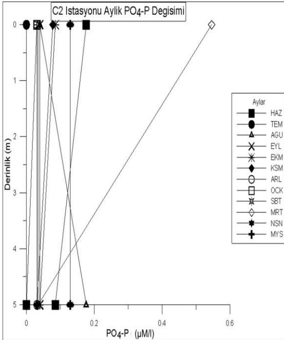
Şekil 4.117. C2 istasyonunda derinliğe bağlı aylık PO 4 -P değişimi
