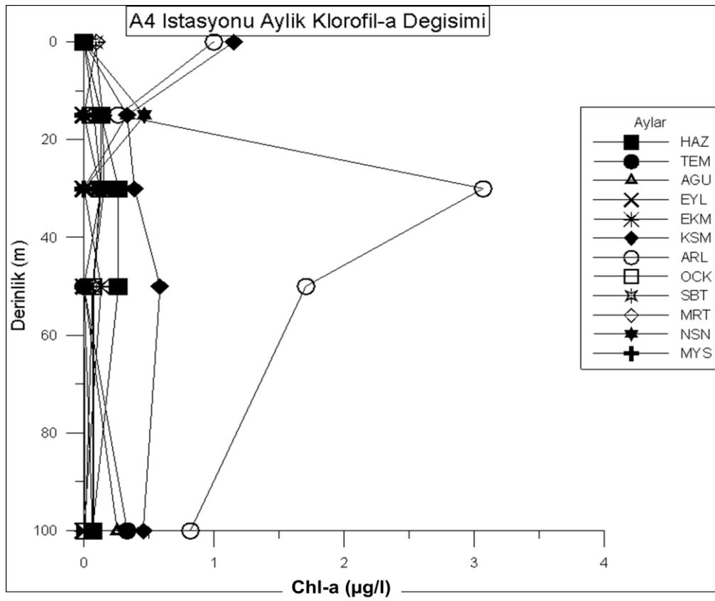
Şekil 4.78. A4 istasyonunda derinliğe bağlı aylık klorofil-a değişimi
