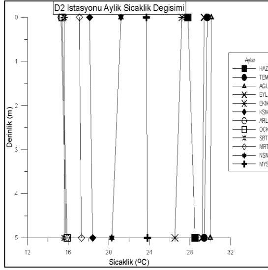
Şekil 4.10. D2 istasyonunda derinliğe bağlı aylık sıcaklık değişimi
