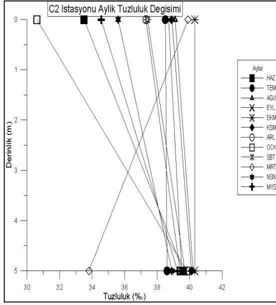
Şekil 4.22. C2 istasyonunda derinliğe bağlı aylık tuzluluk değişimi
