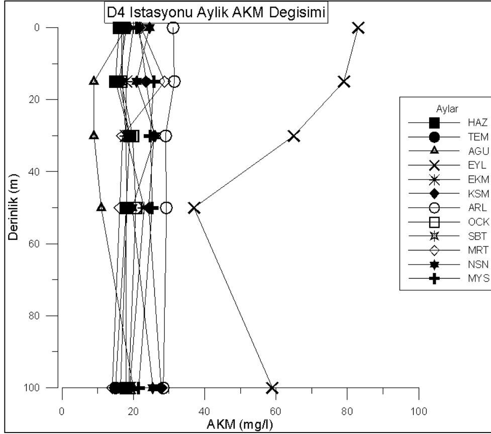
Şekil 4.72. D4 istasyonunda derinliğe bağlı aylık AKM değişimi
