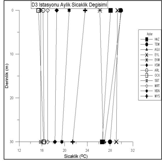
Şekil 4.11. D3 istasyonunda derinliğe bağlı aylık sıcaklık değişimi
