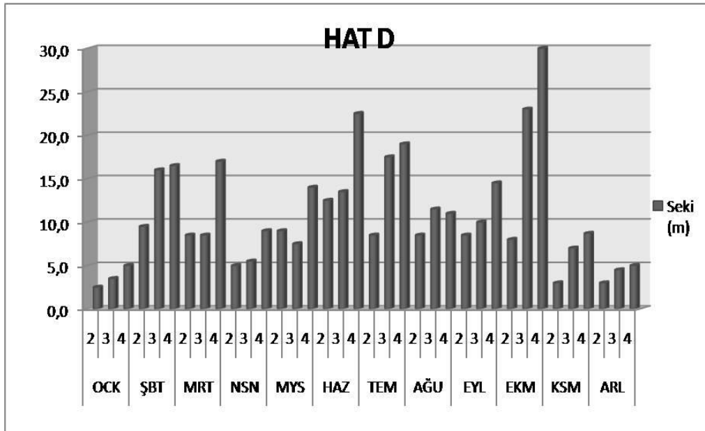
Şekil 4.94. D hattı üzerindeki istasyonların aylara göre seki derinlikleri
