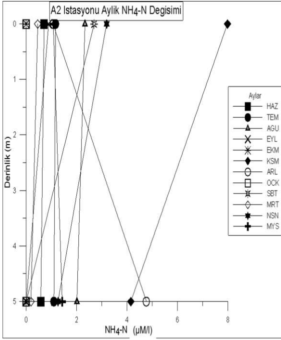
Şekil 4.126. A2 istasyonunda derinliğe bağlı aylık NH 4 -N değişimi
