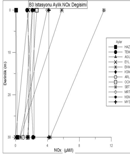
Şekil 4.100. B3 istasyonunda derinliğe bağlı aylık NOx değişimi
