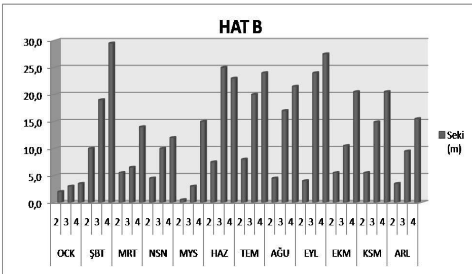
Şekil 4.92. B hattı üzerindeki istasyonların aylara göre seki derinlikleri
