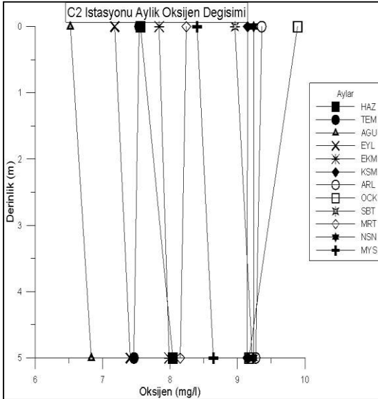
Şekil 4.37. C2 istasyonunda derinliğe bağlı aylık oksijen değişimi
