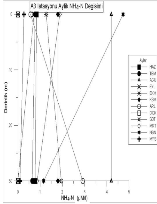
Şekil 4.127. A3 istasyonunda derinliğe bağlı aylık NH 4 -N değişimi
