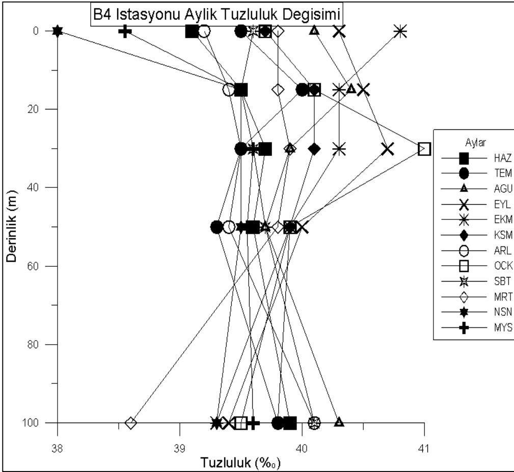
Şekil 4.21. B4 istasyonunda derinliğe bağlı aylık tuzluluk değişimi
