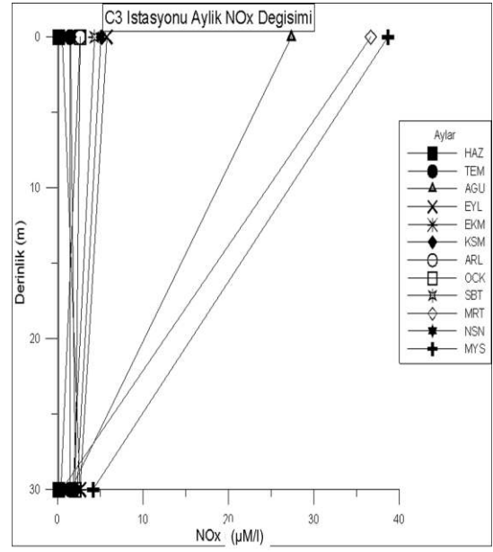
Şekil 4.103. C3 istasyonunda derinliğe bağlı aylık NOx değişimi
