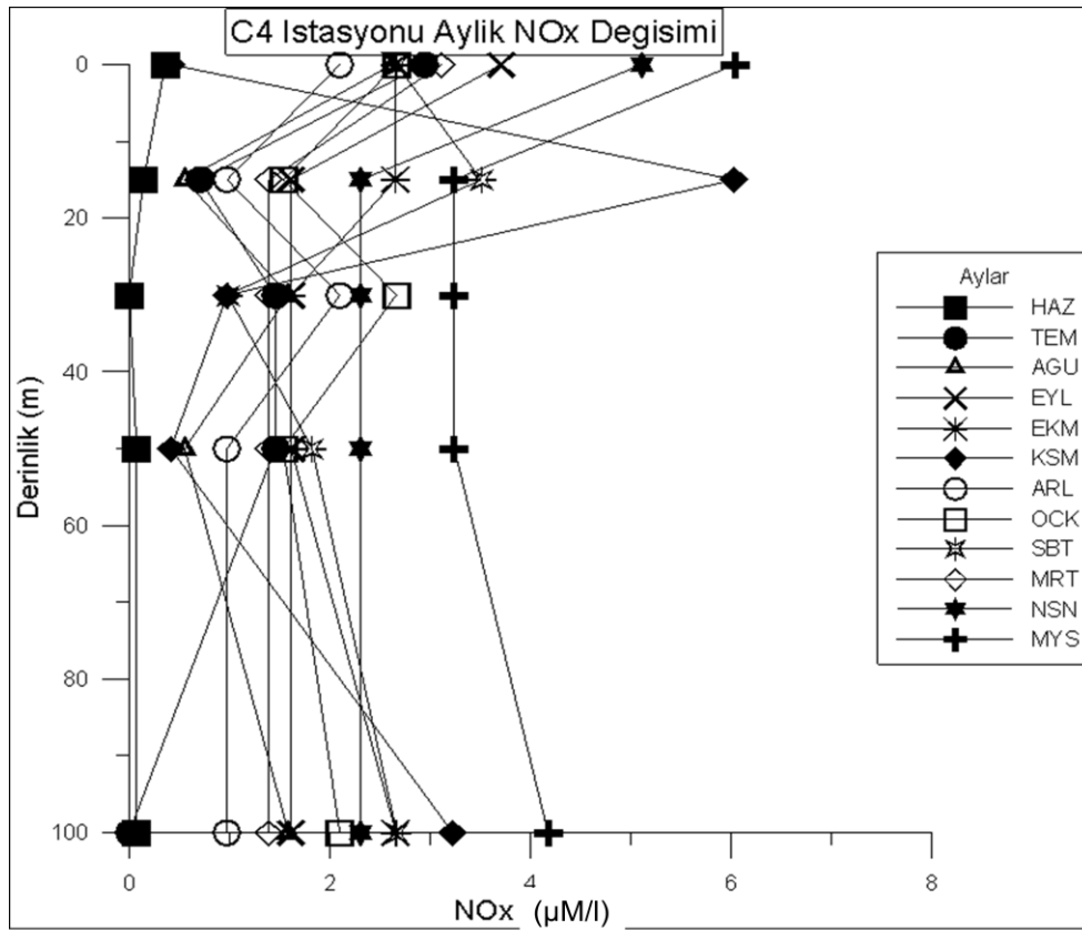
Şekil 4.104. C4 istasyonunda derinliğe bağlı aylık NOx değişimi
