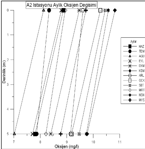
Şekil 4.31. A2 istasyonunda derinliğe bağlı aylık oksijen değişimi
