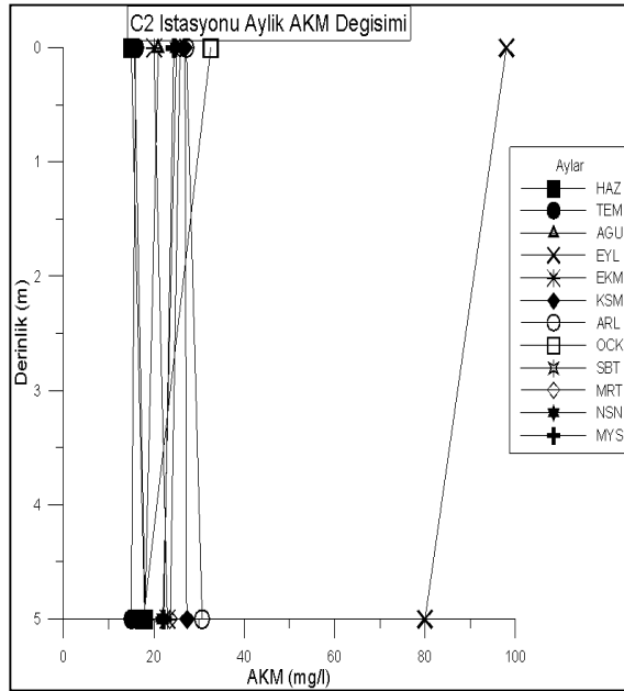
Şekil 4.67. C2 istasyonunda derinliğe bağlı aylık AKM değişimi
