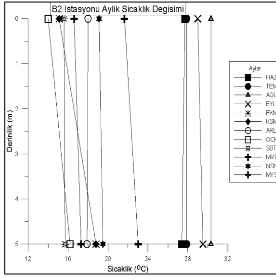
Şekil 4.4. B2 istasyonunda derinliğe bağlı aylık sıcaklık değişimi
