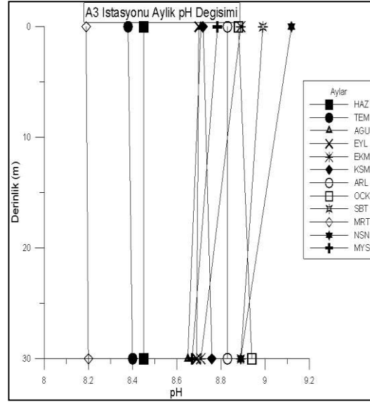
Şekil 4.47. A3 istasyonunda derinliğe bağlı aylık pH değişimi
