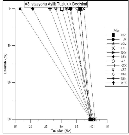
Şekil 4.17. A3 istasyonunda derinliğe bağlı aylık tuzluluk değişimi
