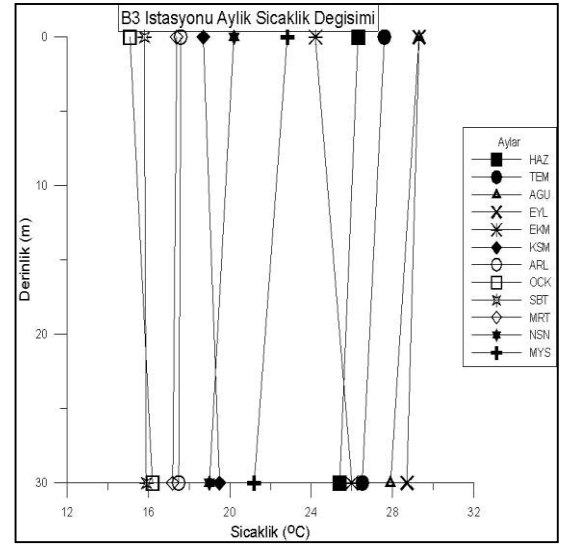
Şekil 4.5. B3 istasyonunda derinliğe bağlı aylık sıcaklık değişimi
