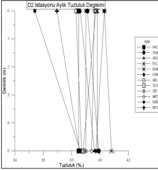
Şekil 4.25. D2 istasyonunda derinliğe bağlı aylık tuzluluk değişimi
