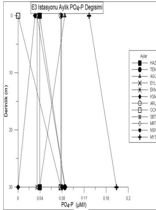
Şekil 4.124. E3 istasyonunda derinliğe bağlı aylık PO 4 -P değişimi
