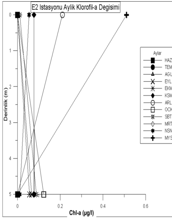
Şekil 4.88. E2 istasyonunda derinliğe bağlı aylık klorofil-a değişimi
