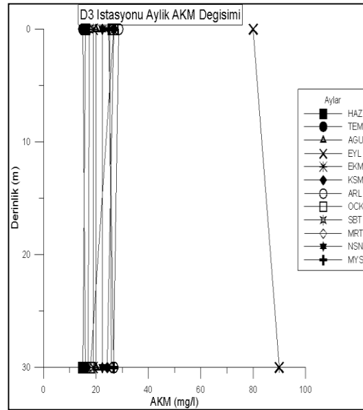
Şekil 4.71. D3 istasyonunda derinliğe bağlı aylık AKM değişimi
