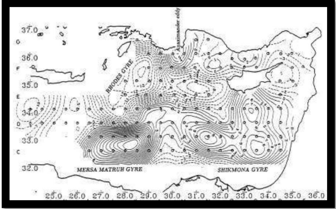
Şekil 2.2. Levant Baseni sirkülasyonunun elemanları (Özsoy vd 1993)
