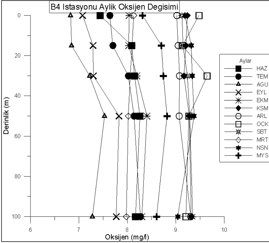
Şekil 4.36. B4 istasyonunda derinliğe bağlı aylık oksijen değişimi
