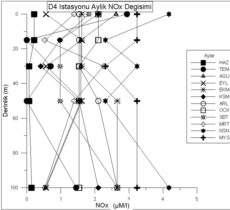
Şekil 4.107. D4 istasyonunda derinliğe bağlı aylık NOx değişimi
