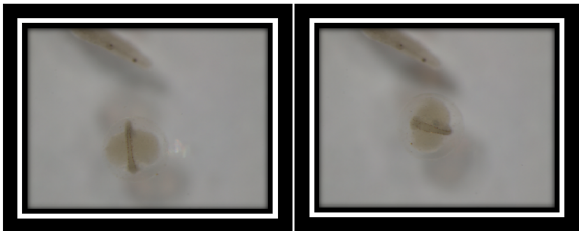
Capros aper
