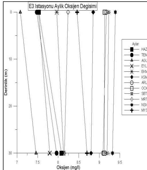
Şekil 4.44. E3 istasyonunda derinliğe bağlı aylık oksijen değişimi
