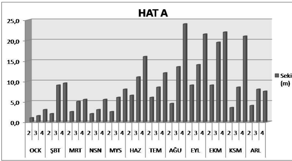
Şekil 4.91. A hattı üzerindeki istasyonların aylara göre seki derinlikleri
