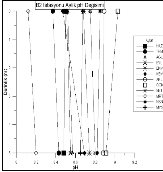
Şekil 4.49. B2 istasyonunda derinliğe bağlı aylık pH değişimi
