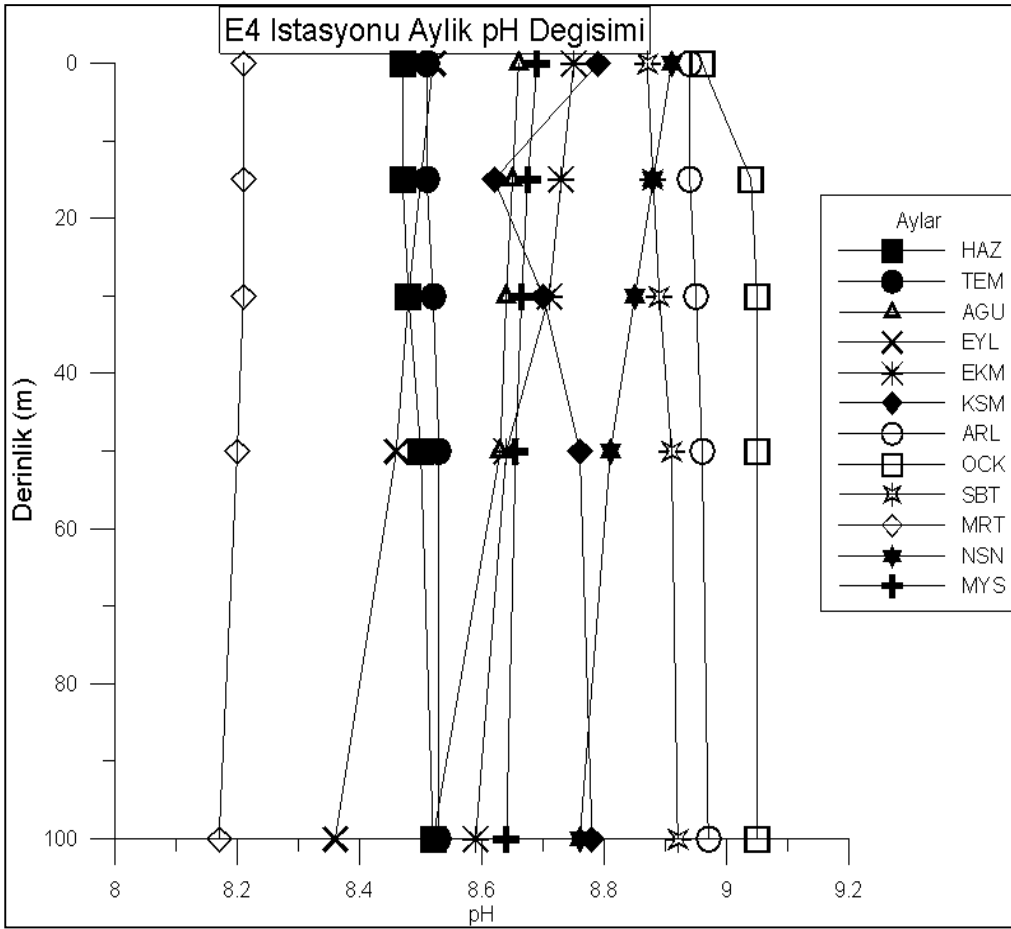
Şekil 4.60. E4 istasyonunda derinliğe bağlı aylık pH değişimi
