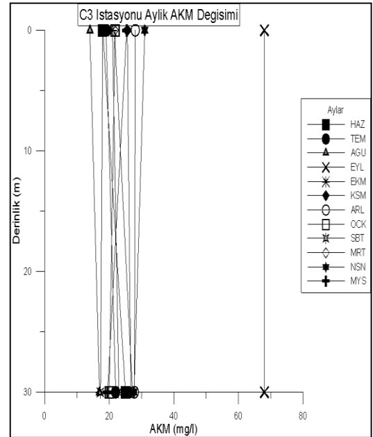
Şekil 4.68. C3 istasyonunda derinliğe bağlı aylık AKM değişimi
