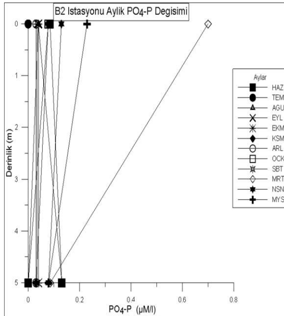
Şekil 4.114. B2 istasyonunda derinliğe bağlı aylık PO 4 -P değişimi
