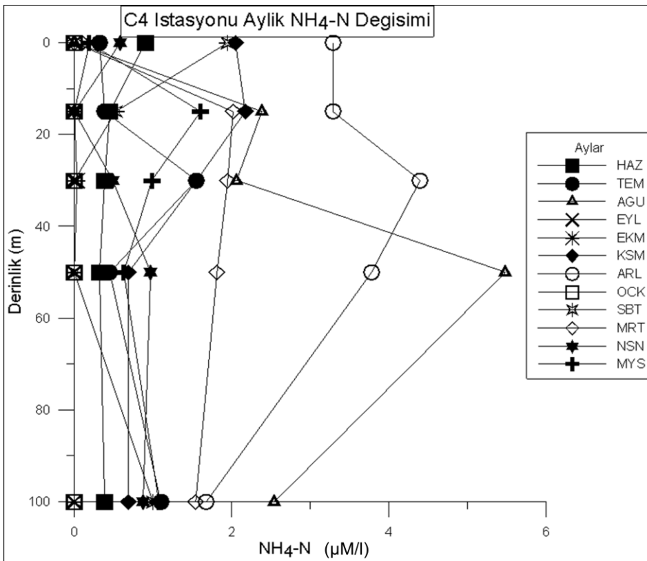
Şekil 4.134. C4 istasyonunda derinliğe bağlı aylık \text{NH}_4\text{-N} değişimi
