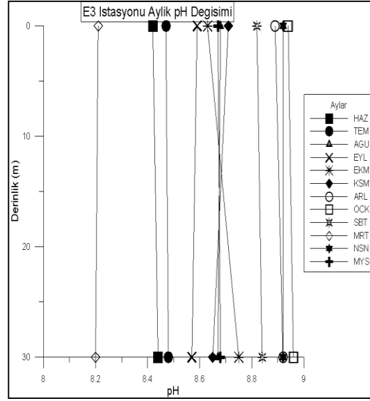
Şekil 4.59. E3 istasyonunda derinliğe bağlı aylık pH değişimi
