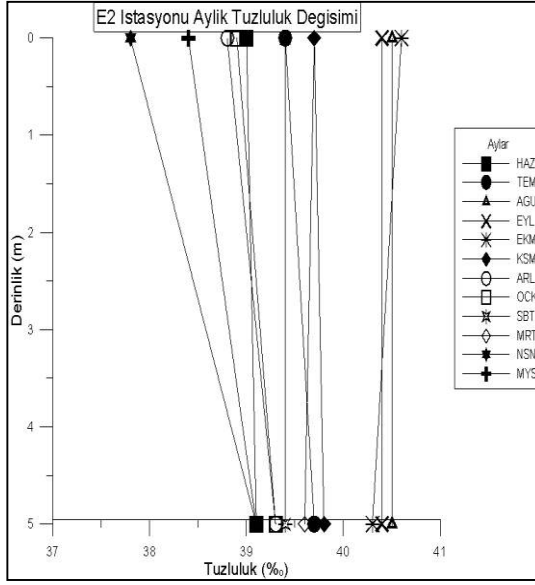
Şekil 4.28. E2 istasyonunda derinliğe bağlı aylık tuzluluk değişimi
