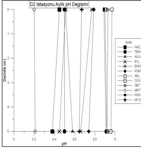
Şekil 4.55. D2 istasyonunda derinliğe bağlı aylık pH değişimi
