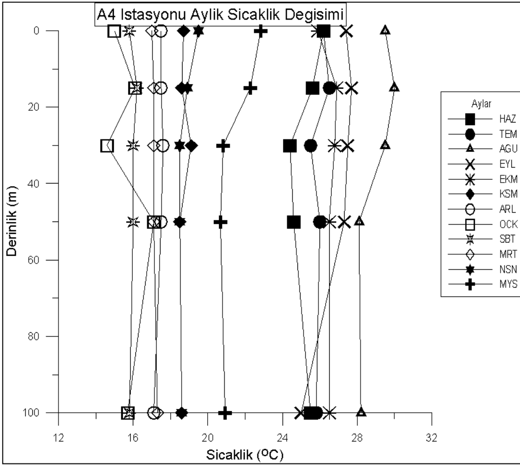
Şekil 4.3. A4 istasyonunda derinliğe bağlı aylık sıcaklık değişimi
