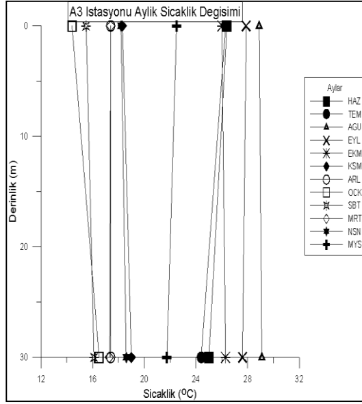
Şekil 4.2. A3 istasyonunda derinliğe bağlı aylık sıcaklık değişimi
