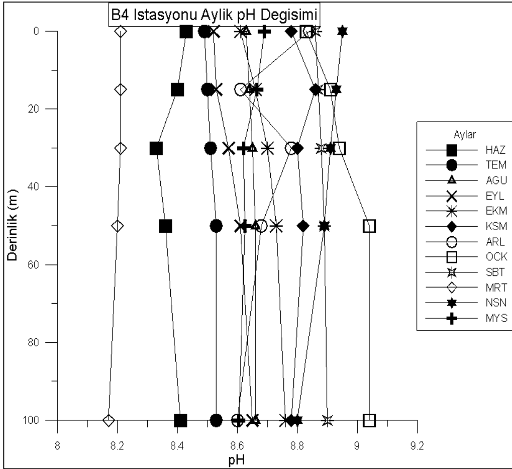
Şekil 4.51. B4 istasyonunda derinliğe bağlı aylık pH değişimi
