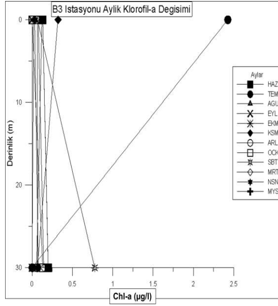
Şekil 4.80. B3 istasyonunda derinliğe bağlı aylık klorofil-a değişimi
