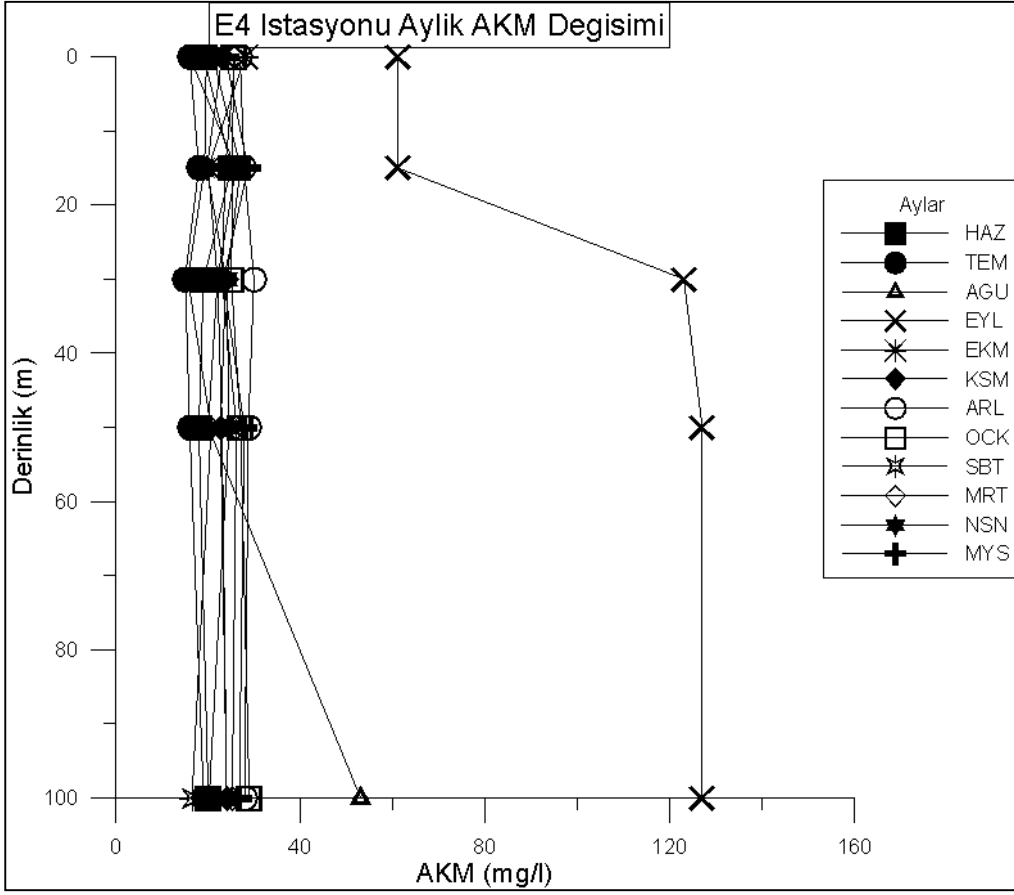
Şekil 4.75. E4 istasyonunda derinliğe bağlı aylık AKM değişimi
