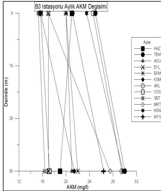
Şekil 4.65. B3 istasyonunda derinliğe bağlı aylık AKM değişimi
