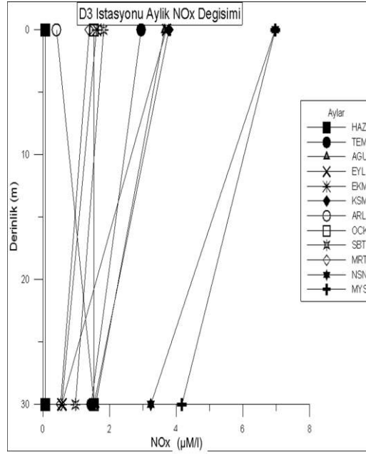
Şekil 4.106. D3 istasyonunda derinliğe bağlı aylık NOx değişimi
