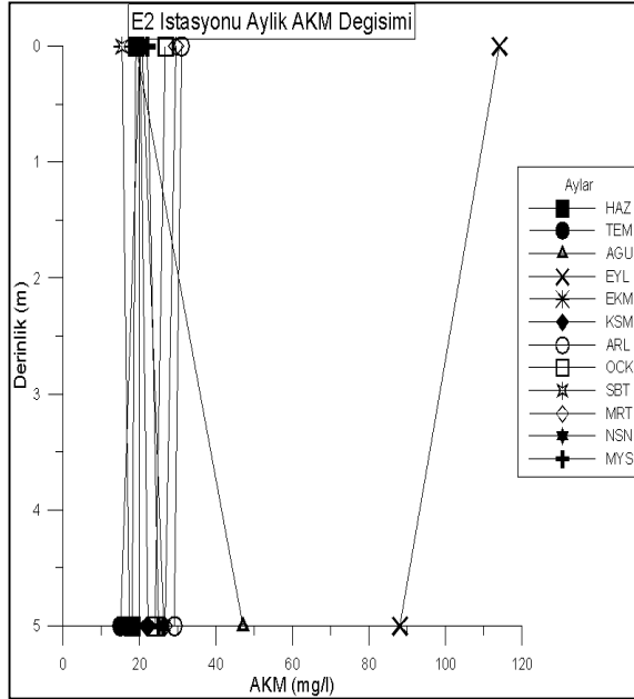
Şekil 4.73. E2 istasyonunda derinliğe bağlı aylık AKM değişimi
