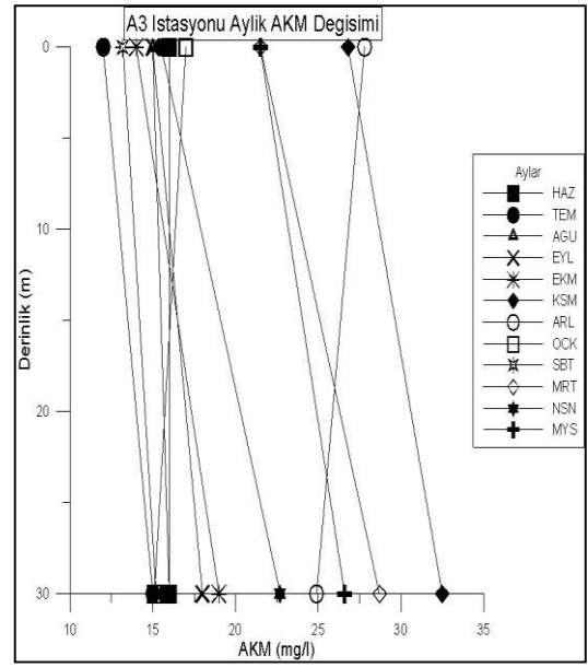
Şekil 4.62. A3 istasyonunda derinliğe bağlı aylık AKM değişimi
