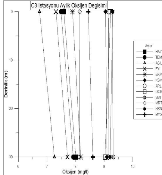
Şekil 4.38. C3 istasyonunda derinliğe bağlı aylık oksijen değişimi
