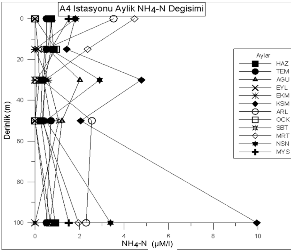
Şekil 4.128. A4 istasyonunda derinliğe bağlı aylık NH 4 -N değişimi
