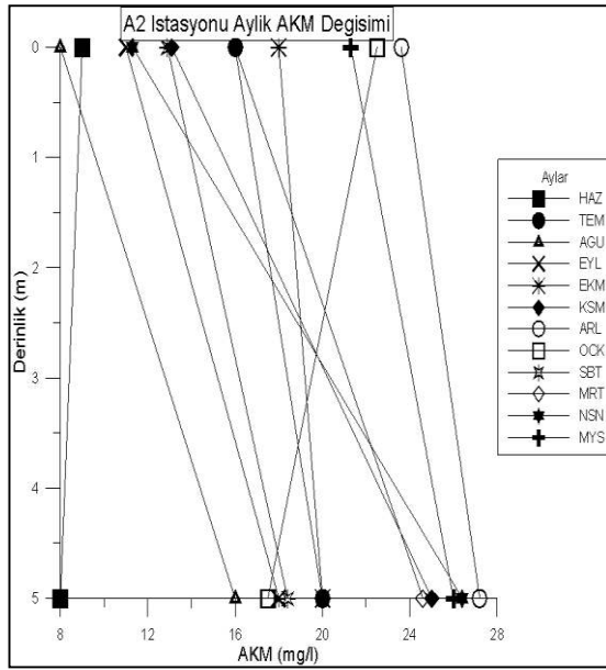
Şekil 4.61. A2 istasyonunda derinliğe bağlı aylık AKM değişimi
