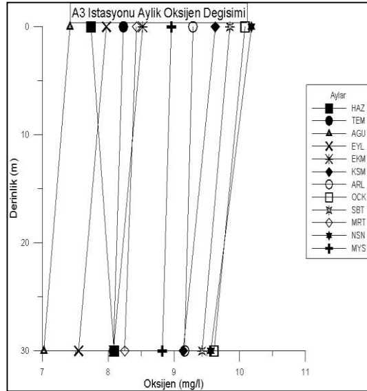
Şekil 4.32. A3 istasyonunda derinliğe bağlı aylık oksijen değişimi
