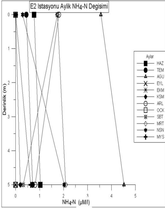
Şekil 4.138. E2 istasyonunda derinliğe bağlı aylık \text{NH}_4\text{-N} değişimi
