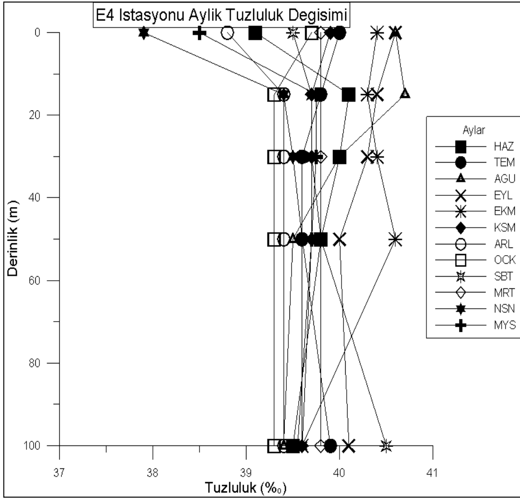
Şekil 4.30. E4 istasyonunda derinliğe bağlı aylık tuzluluk değişimi
