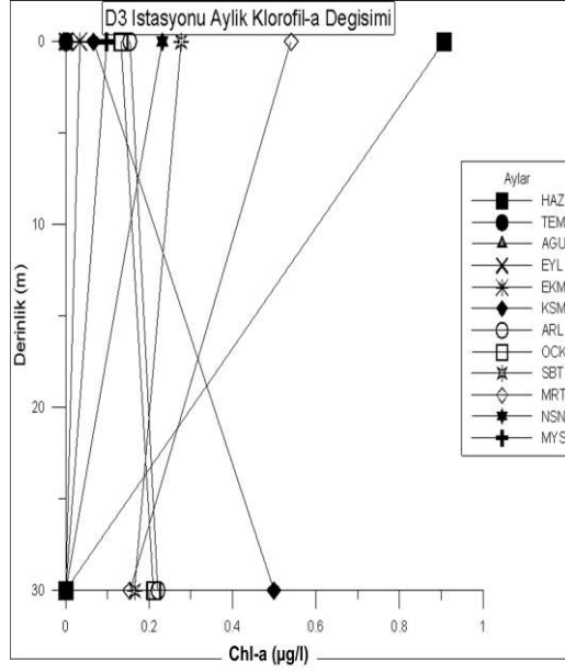
Şekil 4.86. D3 istasyonunda derinliğe bağlı aylık klorofil-a değişimi
