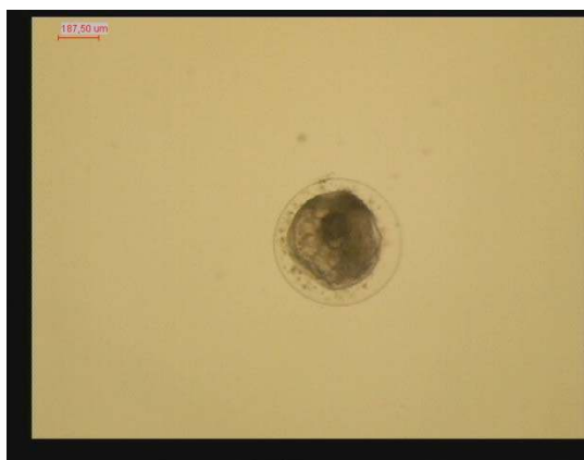
Mugilidae sp.2
