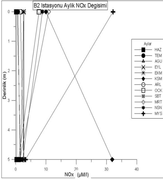
Şekil 4.99. B2 istasyonunda derinliğe bağlı aylık NOx değişimi
