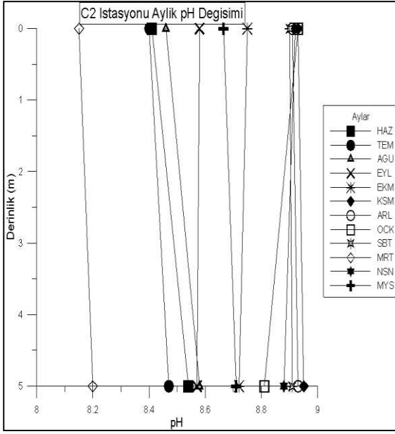
Şekil 4.52. C2 istasyonunda derinliğe bağlı aylık pH değişimi
