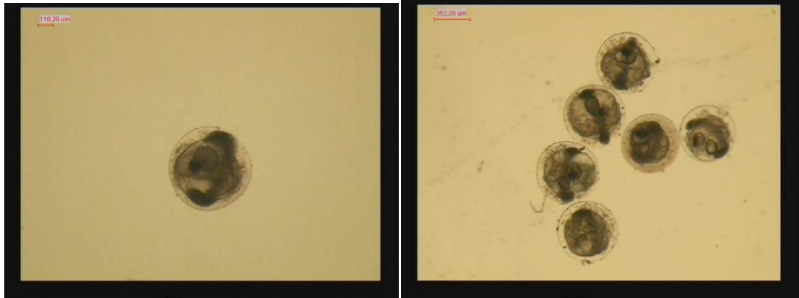
Upeneus moluccensis
