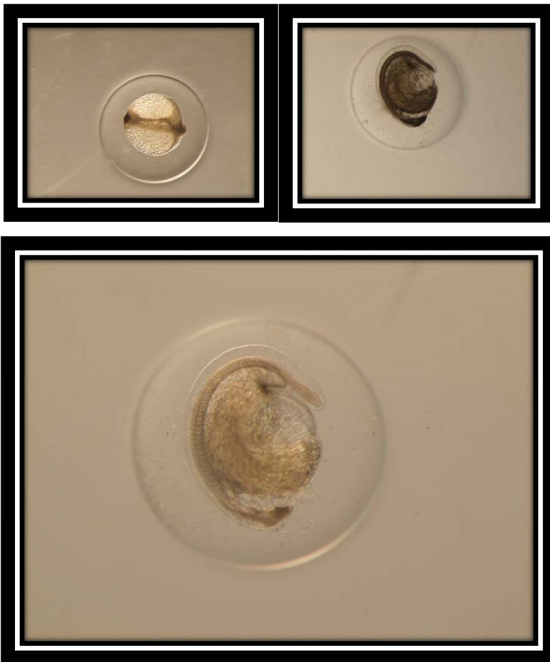
Gymnothorax unicolor
