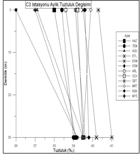
Şekil 4.23. C3 istasyonunda derinliğe bağlı aylık tuzluluk değişimi
