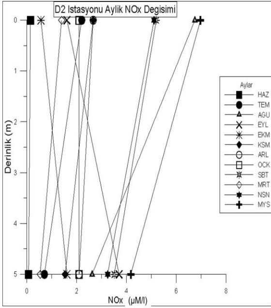
Şekil 4.105. D2 istasyonunda derinliğe bağlı aylık NOx değişimi
