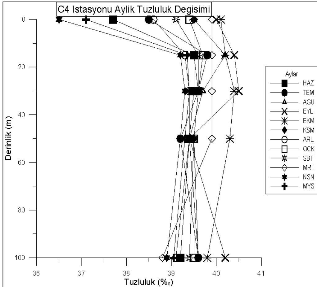
Şekil 4.24. C4 istasyonunda derinliğe bağlı aylık tuzluluk değişimi
