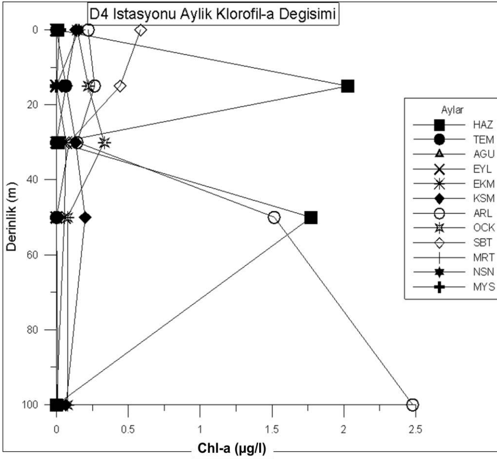
Şekil 4.87. D4 istasyonunda derinliğe bağlı aylık klorofil-a değişimi
