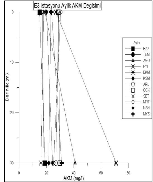
Şekil 4.74. E3 istasyonunda derinliğe bağlı aylık AKM değişimi
