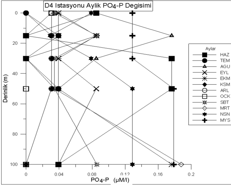
Şekil 4.122. D4 istasyonunda derinliğe bağlı aylık PO 4 -P değişimi
