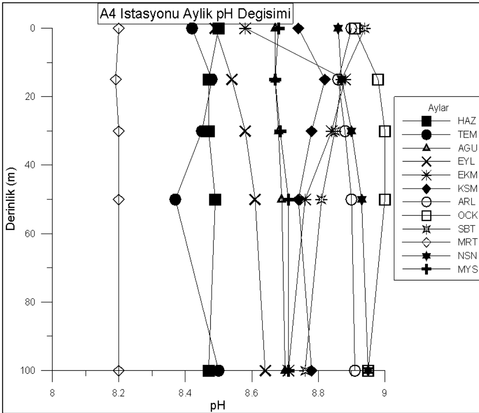
Şekil 4.48. A4 istasyonunda derinliğe bağlı aylık pH değişimi
