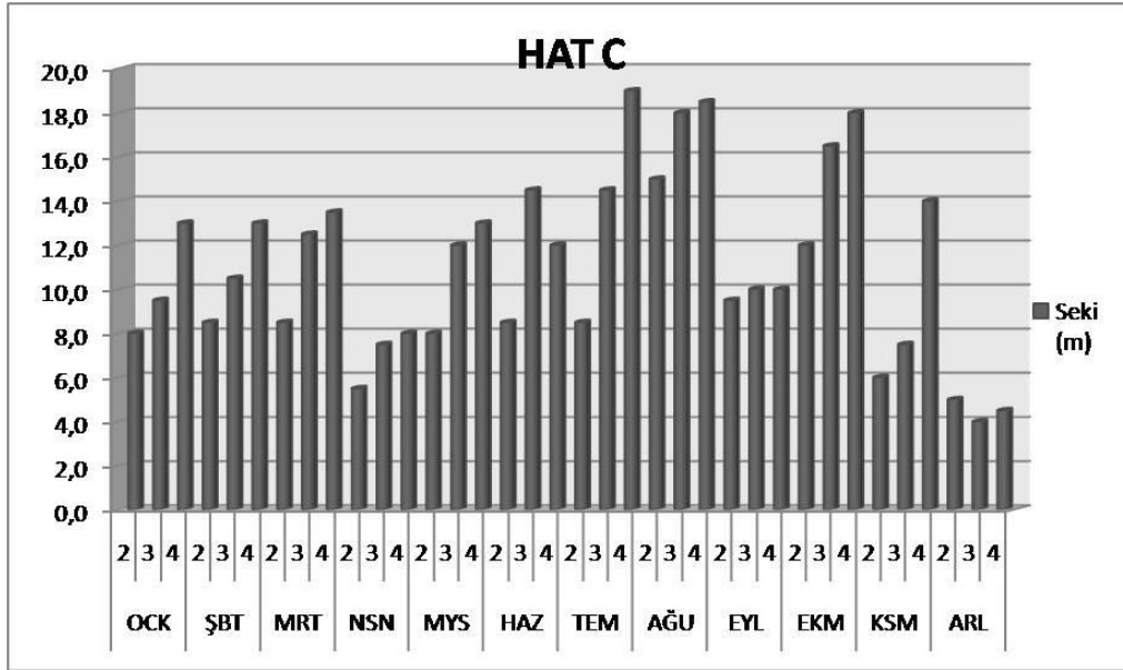
Şekil 4.93. C hattı üzerindeki istasyonların aylara göre seki derinlikleri
