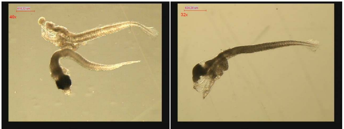
Chlorophthalmus agassizi
