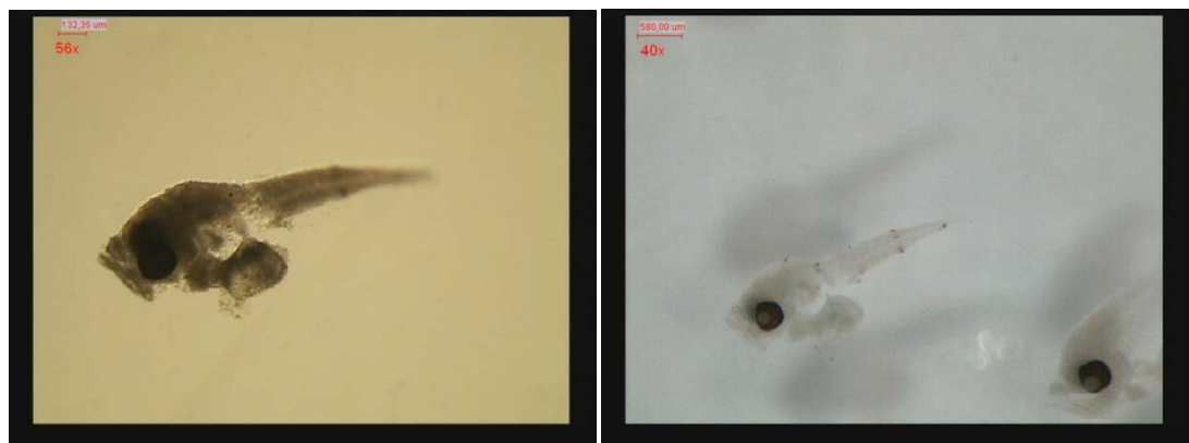
Bregmaceros atlanticus
