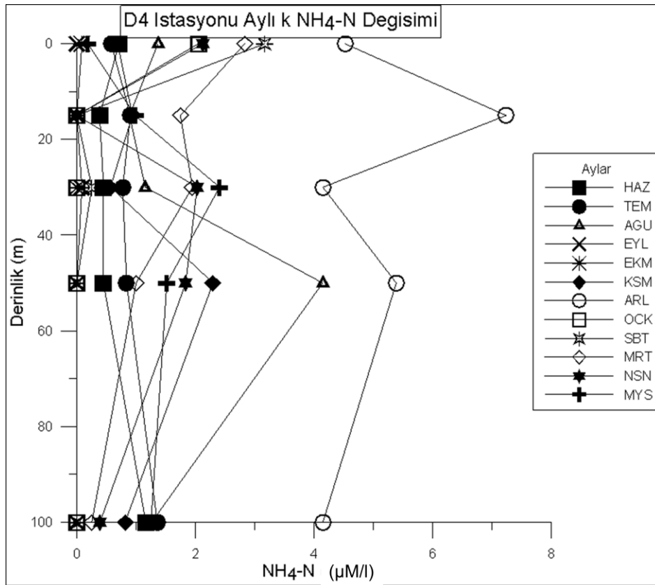
Şekil 4.137. D4 istasyonunda derinliğe bağlı aylık NH 4 -N değişimi
