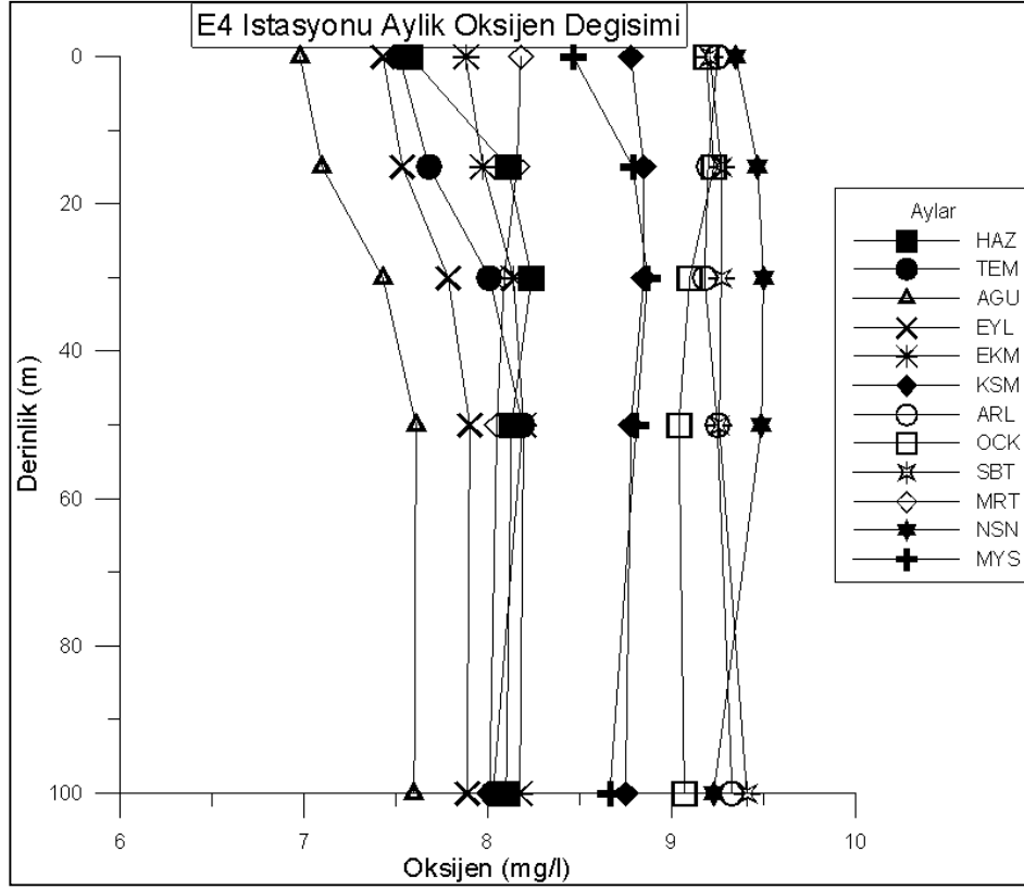
Şekil 4.45. E4 istasyonunda derinliğe bağlı aylık oksijen değişimi
