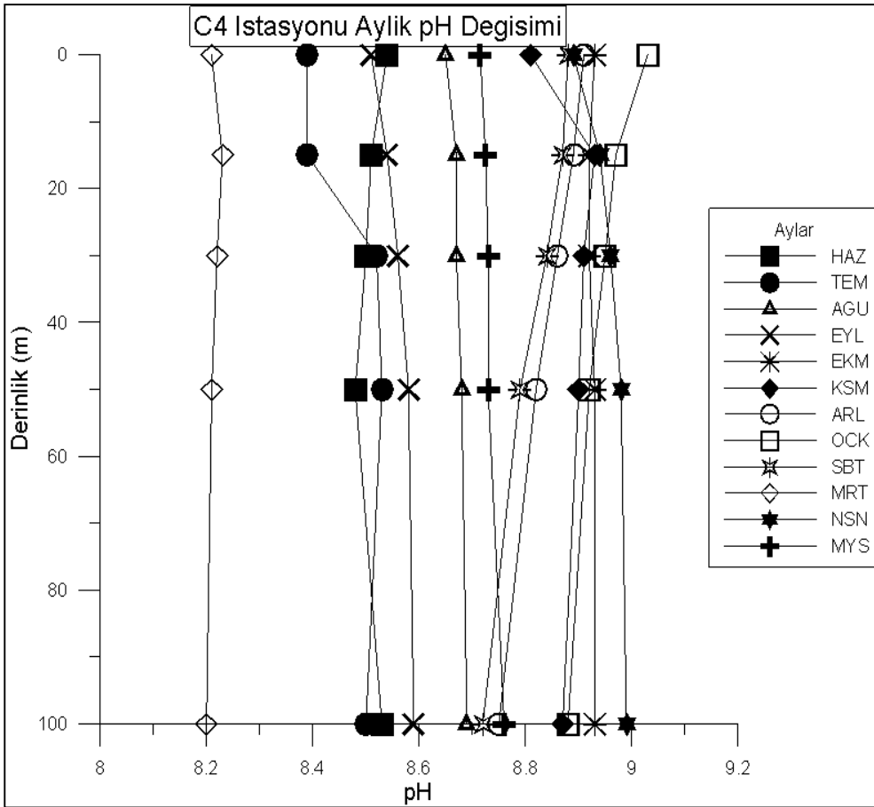
Şekil 4.54. C4 istasyonunda derinliğe bağlı aylık pH değişimi
