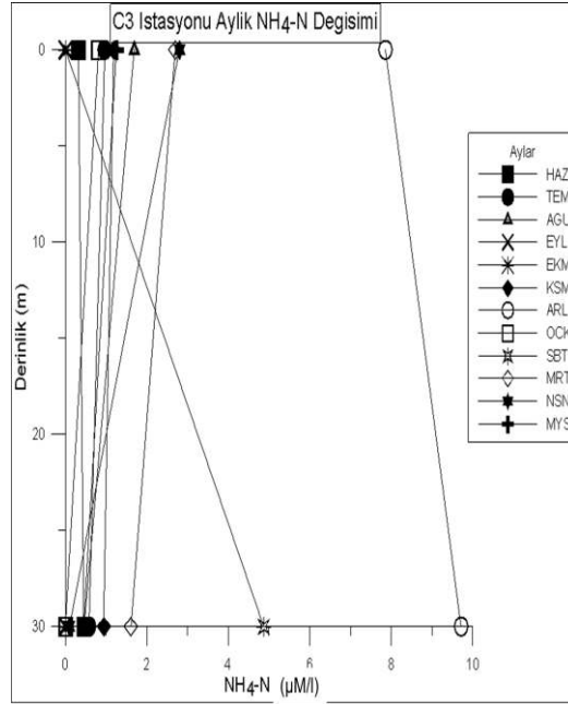
Şekil 4.133. C3 istasyonunda derinliğe bağlı aylık \text{NH}_4\text{-N} değişimi
