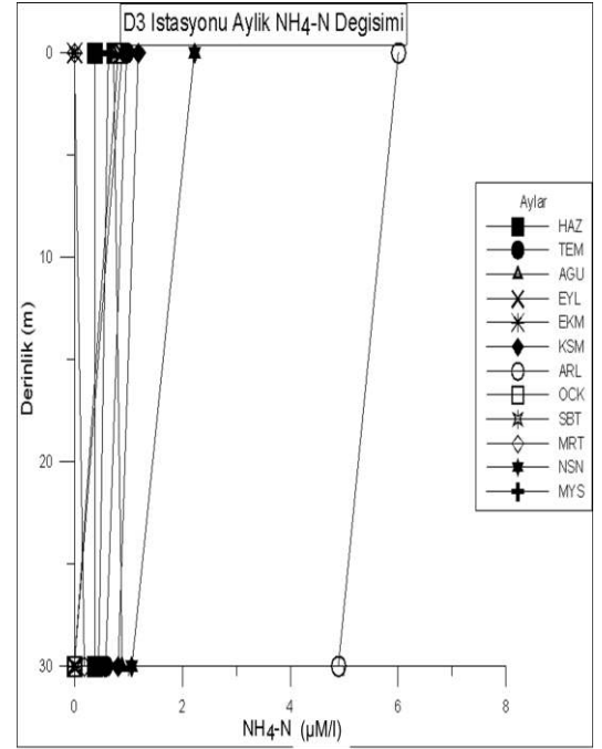
Şekil 4.136. D3 istasyonunda derinliğe bağlı aylık NH 4 -N değişimi
