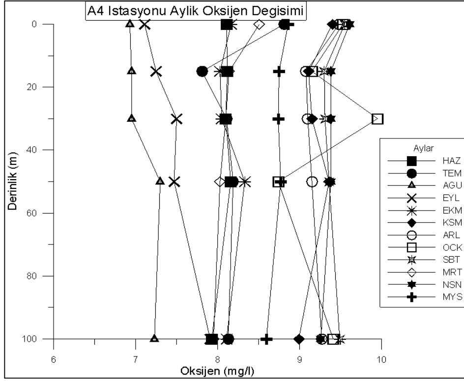
Şekil 4.33. A4 istasyonunda derinliğe bağlı aylık oksijen değişimi
