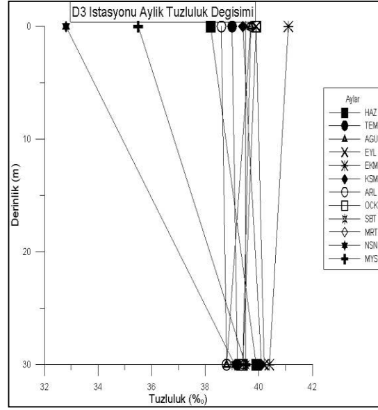
Şekil 4.26. D3 istasyonunda derinliğe bağlı aylık tuzluluk değişimi
