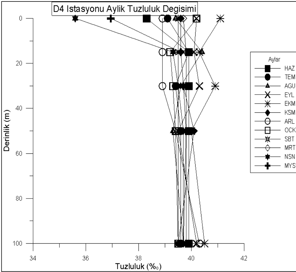
Şekil 4.27. D4 istasyonunda derinliğe bağlı aylık tuzluluk değişimi
