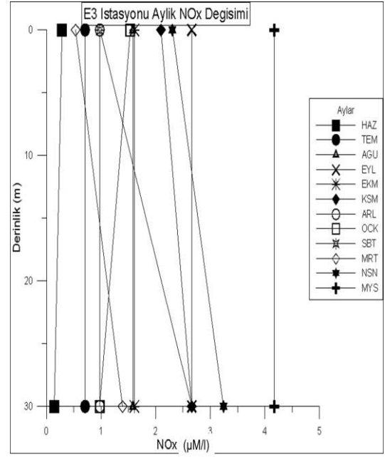
Şekil 4.109. E3 istasyonunda derinliğe bağlı aylık NOx değişimi
