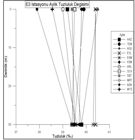
Şekil 4.29. E3 istasyonunda derinliğe bağlı aylık tuzluluk değişimi
