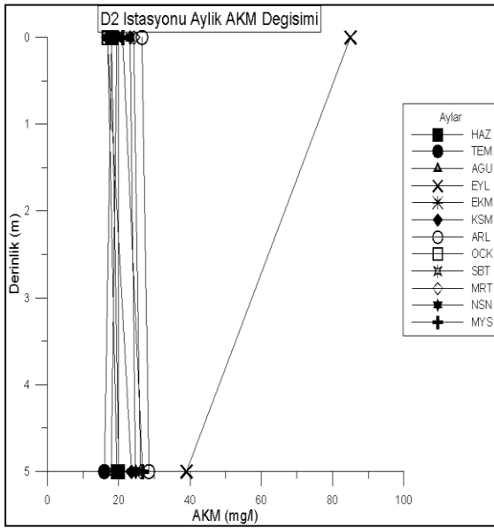
Şekil 4.70. D2 istasyonunda derinliğe bağlı aylık AKM değişimi
