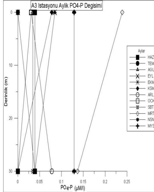
Şekil 4.112. A3 istasyonunda derinliğe bağlı aylık PO 4 -P değişimi
