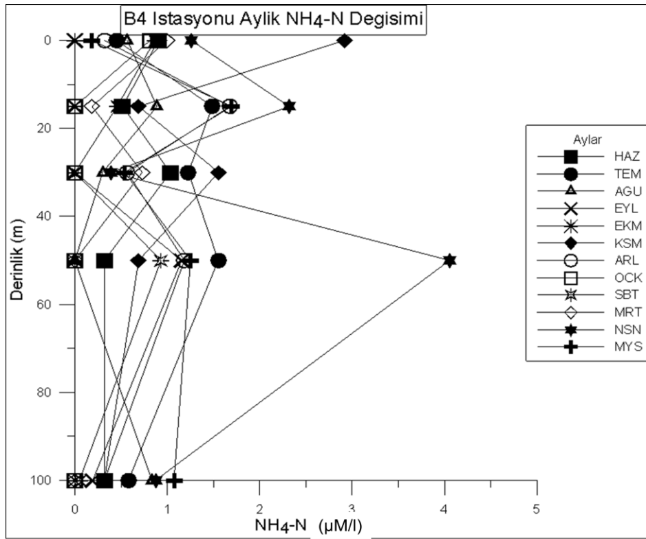
Şekil 4.131. B4 istasyonunda derinliğe bağlı aylık \text{NH}_4\text{-N} değişimi
