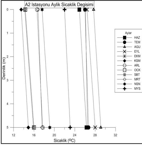
Şekil 4.1. A2 istasyonunda derinliğe bağlı aylık sıcaklık değişimi
