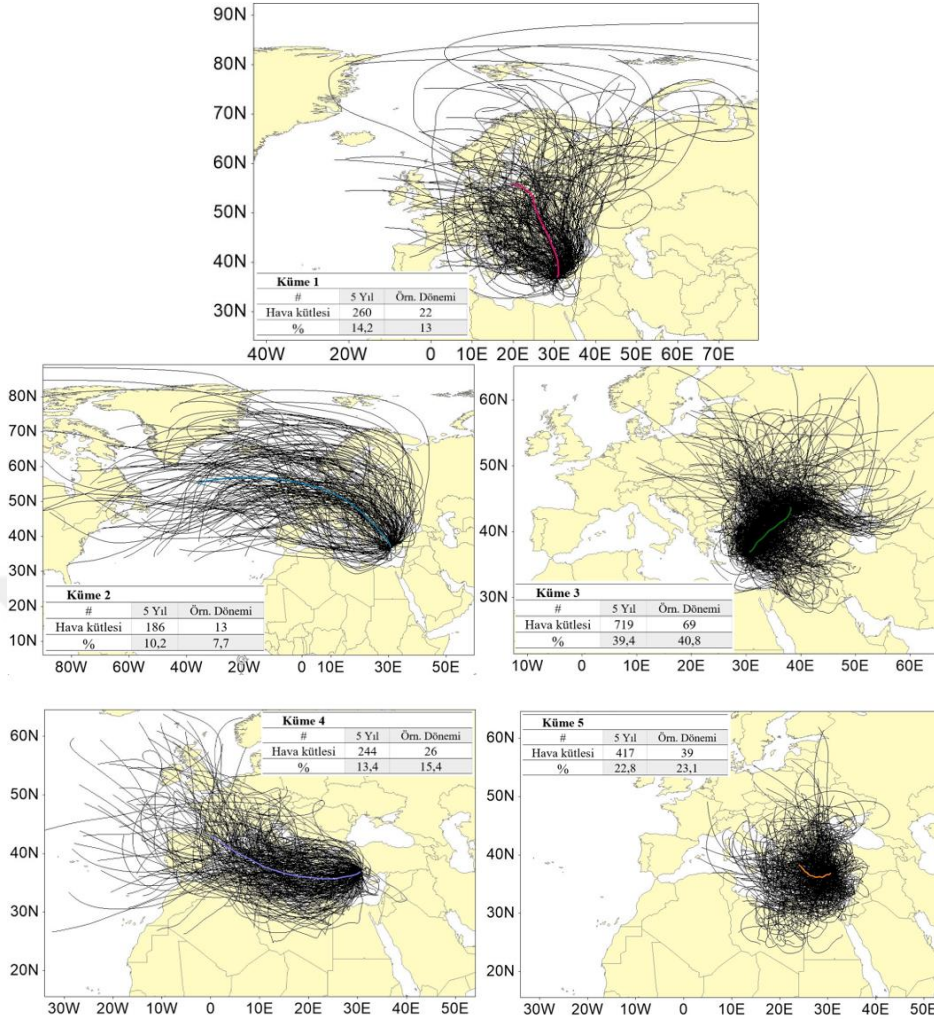
Şekil 4.24. Her bir kümeden gelen hava kütlesi sayısı ve oranı ve her bir kümenin içindeki geri hava yörüngeleri
