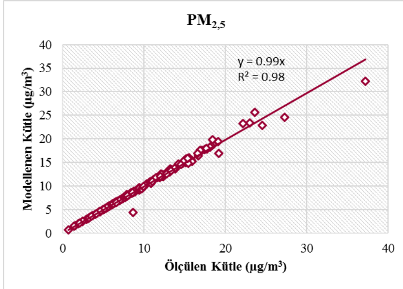
Şekil 4.28. Ölçülen PM 2,5 konsantrasyonun modellenen PM 2,5 konsantrasyon ile karşılaştırması
