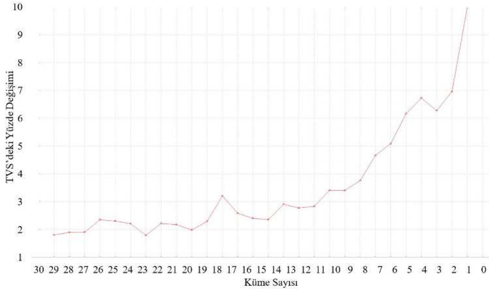
Şekil 4.21. Azalan küme sayıları ile birlikte TVS'deki yüzde değişimi
