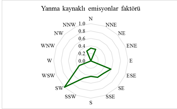
Şekil 4.67. Yanma kaynaklı emisyonlar faktörü için sadece Temmuz ve Ağustos aylarının G-skorları kullanılarak hazırlan KOF grafiği
