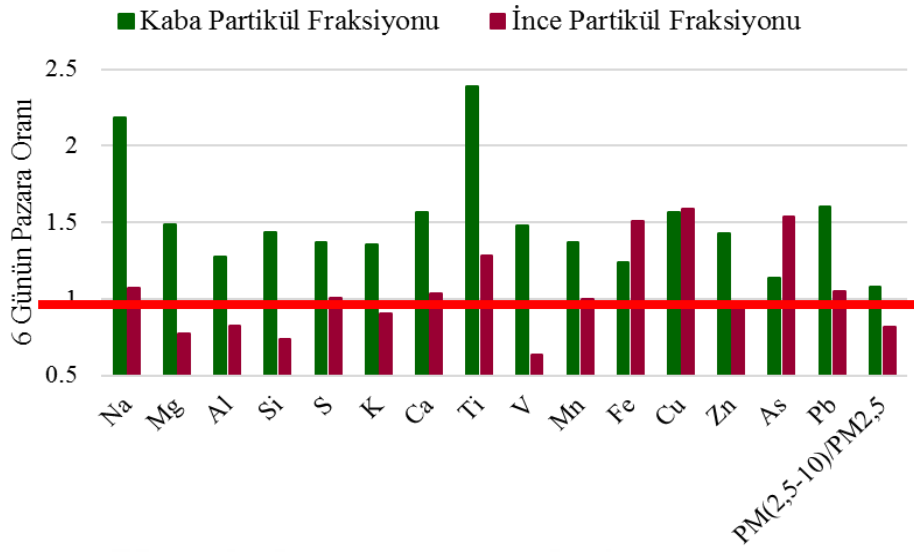
Şekil 4.17. Elementlerin kaba ve ince partikül boyutundaki Pazartesi-Cumartesi (6 Gün) ortalama konsantrasyonlarının Pazar günü ortalama konsantrasyonlarına oranı
