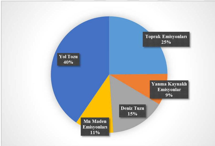
Şekil 4.58. Faktörlerin modellenen PM 2,5-10 kütle konsantrasyonuna yaptıkları yüzde katkılar
