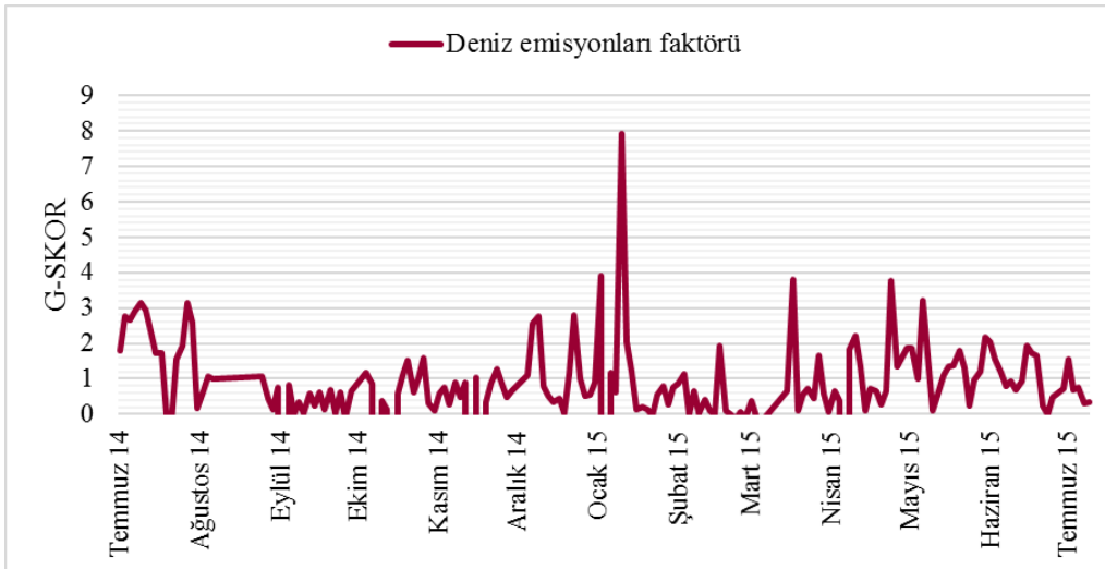
Şekil 4.48. Deniz emisyonları faktörünün G-skorlarının zamansal değişimi
