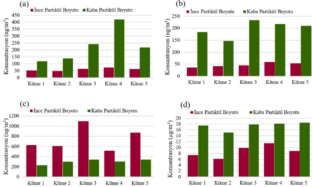
Şekil 4.23. Her bir kümede kaba ve ince partikül fraksiyonunda (a) Na, (b) Al, (c) S ve (d) PM'in günlük ortalama konsantrasyon değerleri
