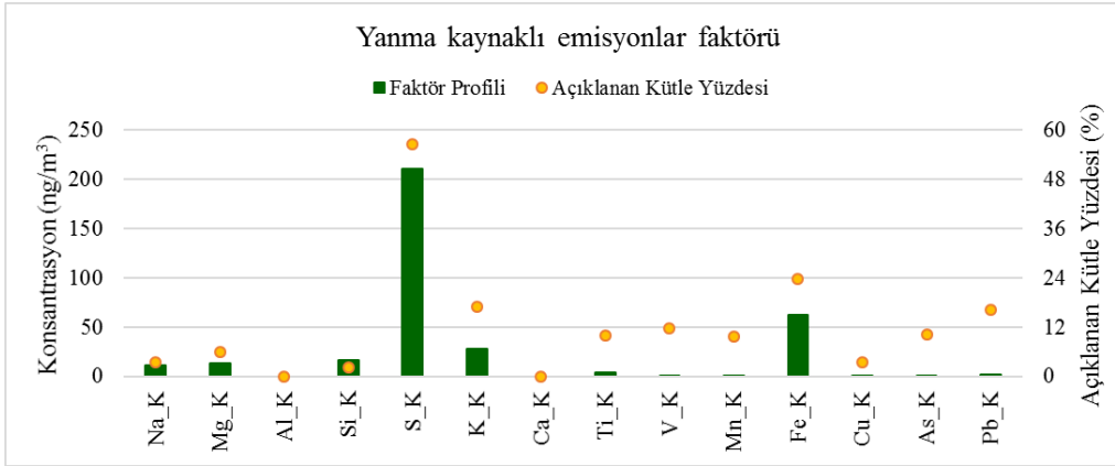
Şekil 4.64. Yanma kaynaklı emisyonlar faktörünün faktör profili ile elementlerin açıklanan yüzde kütleleri
