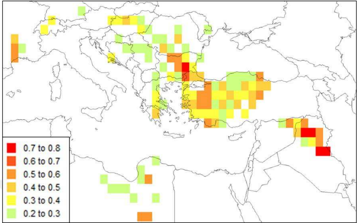
Şekil 4.39. İkincil kükürt faktörünün G-skorum ile hazırlanan PKKFK sonuçları
