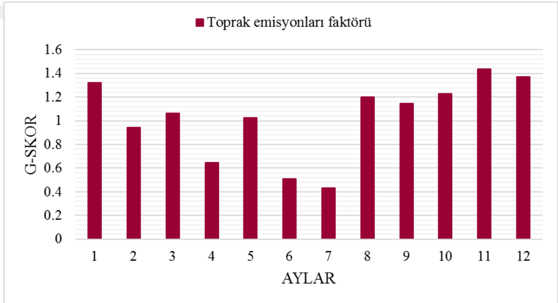
Şekil 4.53. Toprak emisyonları faktörünün G-skorların aylık değişimi
