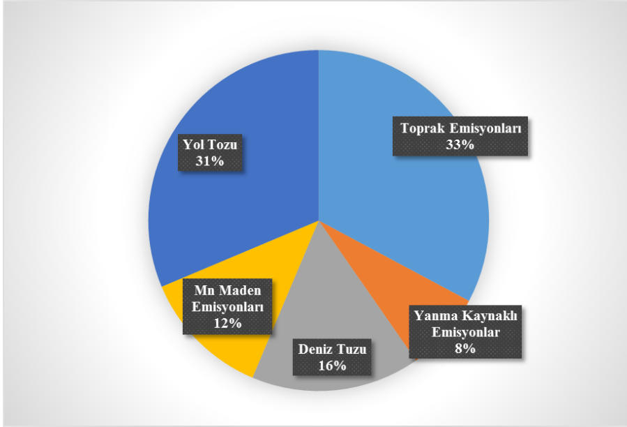
Şekil 4.57. Faktörlerin modellenen elementel kütle konsantrasyonuna yaptıkları yüzde katkılar
