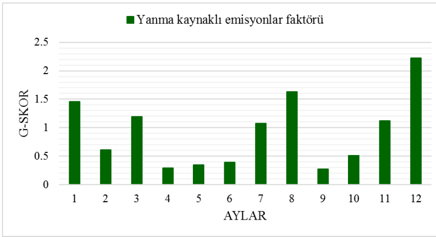
Şekil 4.65. Yanma kaynaklı emisyonlar faktörünün aylık G-skor değişimleri
