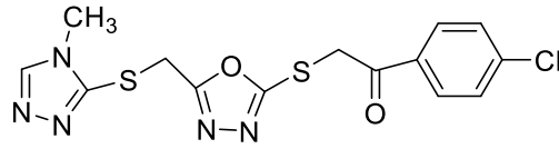
Şekil 5.21. 1-(4-Klorofenil)-2-((5-(((4-metil-4H-1,2,4-triazol-3-il)tiyo)metil)-1,3,4-oksadiazol-2-il)tiyo)etan-1-on ( 4f )
