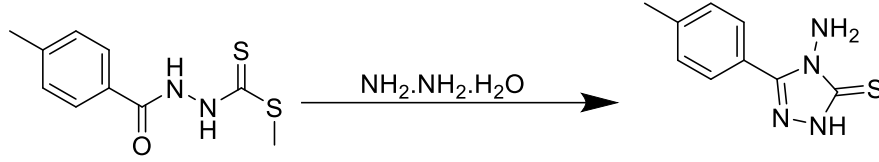
Şekil 2.9. Hidrazin'den triazol sentezi
