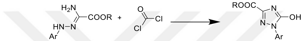
Şekil 2.13. Fosgen ile triazol sentezi
