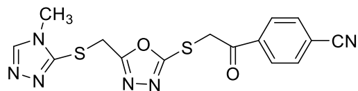
Şekil 5.9. 4-(2-((5-(((4-Metil-4H-1,2,4-triazol-3-il)tiyo)metil)-1,3,4-oksadiazol-2-il)tiyo)asetil)benzonitril (4c)
