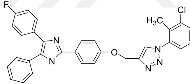
Şekil 2.55. 1-(3-Kloro-2-metilfenil)-4-((4-(4-(4-florofenil)-5-fenil-1,1,2-imidazol-2-il)fenoksi)metil)-1H-1,2, 3-triazol
