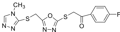
Şekil 5.17. 1-(4-Florofenil)-2-((5-(((4-metil-4H-1,2,4-triazol-3-il)tiyo)metil)-1,3,4-oksadiazol-2-il)tiyo)etan-1-on ( 4e )
