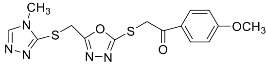
Şekil 5.5. 1-(4-Metoksifenil)-2-((5-(((4-metil-4H-1,2,4-triazol-3-il)tiyo)metil)-1,3,4-oksadiazol-2-il)tiyo)etan-1-on ( 4b )
