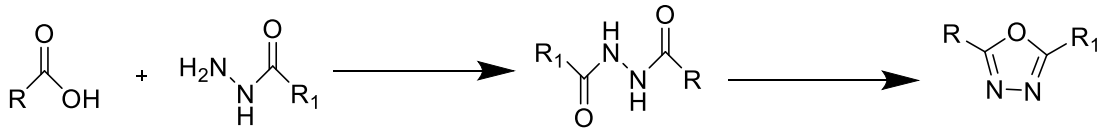
Şekil 2.16. Karboksilik asit türevi ile açılhidrazit türevinden oksadiazol sentezi
