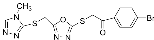
Şekil 5.25. 1-(4-Bromofenil)-2-(((5-(((4-metil-4H-1,2,4-triazol-3-il)tiyo)metil)-1,3,4-oksadiazol-2-il)tiyo)etan-1-on ( 4g )
