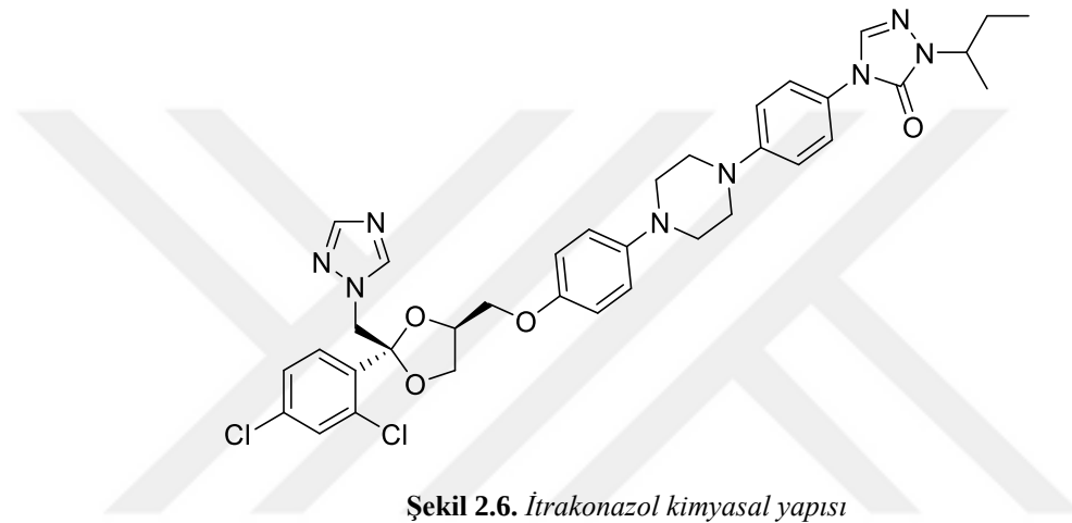
Şekil 2.6. İtrakonazol kimyasal yapısı
