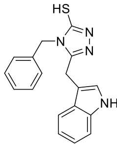
Şekil 2.30. 5-((1H-İndol-3-il)metil)-4-benzil-4H-1,2,4-triazol-3-tiyo
