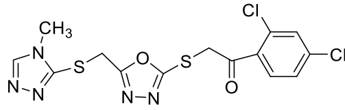
Şekil 5.37. 1-(2,4-Diklorofenil)-2-(((4-metil-4H-1,2,4-triazol-3-il)tiyo)metil)-1,3,4-oksadiazol-2-il)tiyo)etan-1-on (4j)
