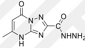
Şekil 2.34. 5-Metil-7-okso-4,7-dihidro-[1,2,4]triazolo[1,5-a]pirimidine-2-karbohidrazid
