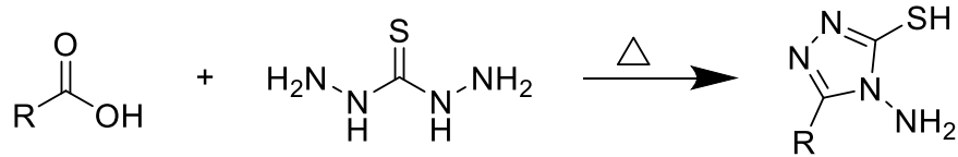
Şekil 2.14. Tiyokarbohidrazid türevi bileşiğinin karboksilli asit ile reaksiyonu
