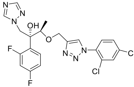
Şekil 2.22. (2R,3R)-3-((1-(2,4-Diklorofenil)-1H-1,2,3-triazol-4-il)metoksi)-2-(2,4-diflorofenil)-1-(1H-1,2,4-triazol-1-il)butan-2-ol
