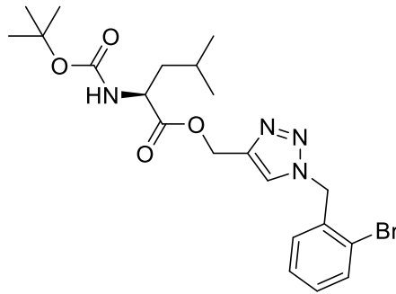
Şekil 2.35. 1-(2-Bromobenzil)-1H-1,2,3-triazol-4-il)metil (ter-butoksi-karbonil)-L-lösinat
