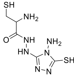
Şekil 2.33. 2-Amino-N'-(4-amino-5-merkapto-4H-1,2,4-triazol-3-il)-3merkaptopropanhidrazid
