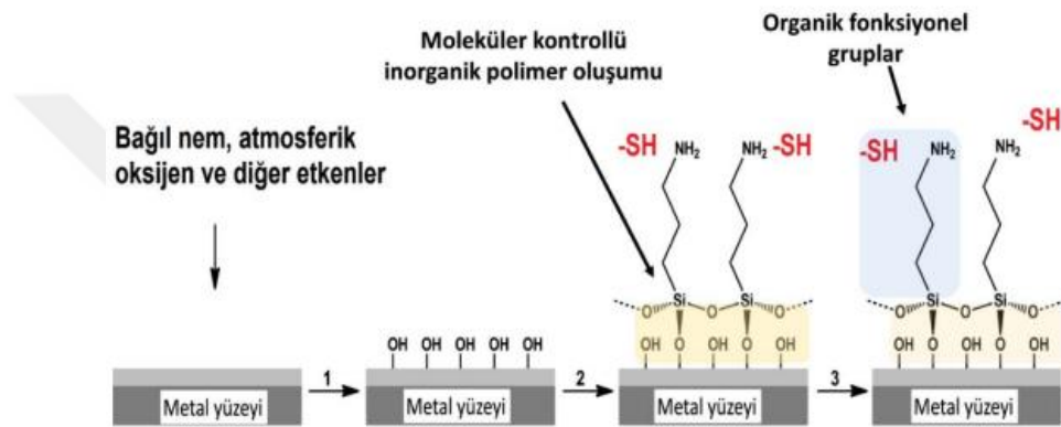
Şekil 2.9 Yüzeyinde -SH ve \text{NH}_2 grupları içeren kaplamaların yüzeye tutunması.
