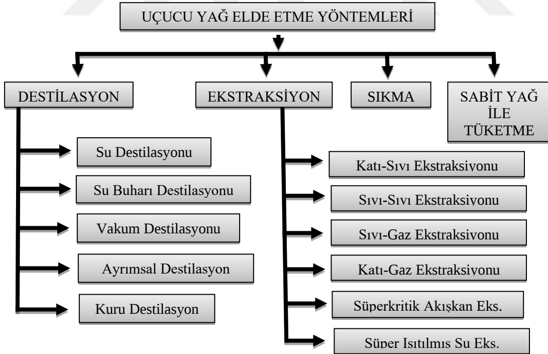
Şekil 2. 13 Uçucu yağ elde etme yöntemleri.
