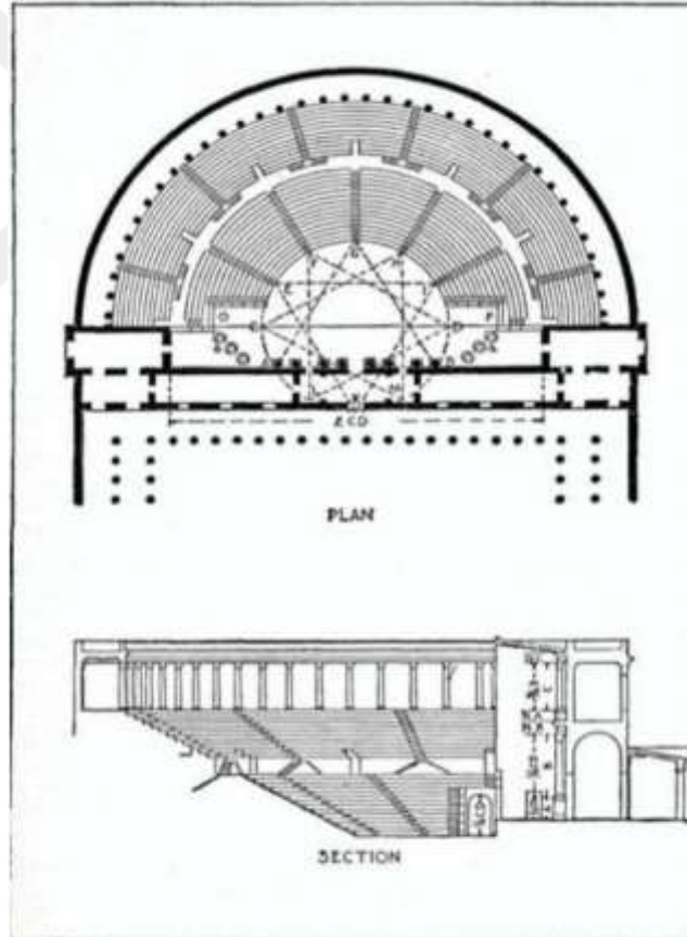
Resim 38: Vitruvius'a göre Roma Tiyatro Planı (Fişenk ve Satıcı,2021:129)
