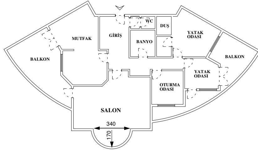
Şekil 3.4. Çağrı sitesi normal kat planı
