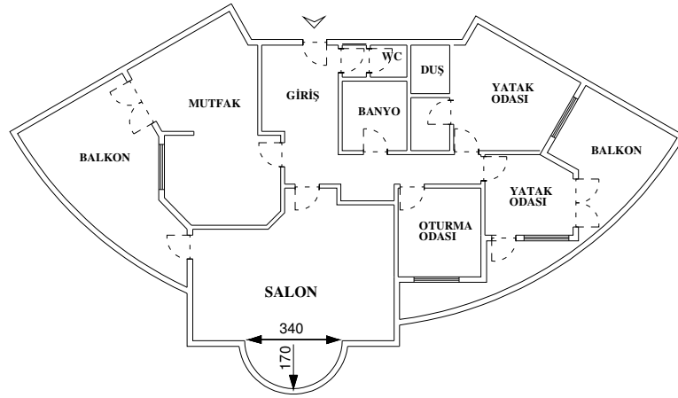
Şekil 3.5. Açelya sitesi normal kat planı
