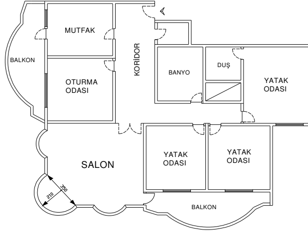
Şekil 3.3. Menekşe sitesi kat planı
