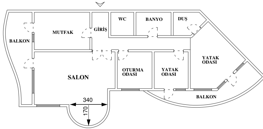
Şekil 3.2. Seymen Seley sitesi normal kat planı
