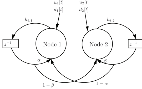
(b) CTA diffusion adaptation scheme
