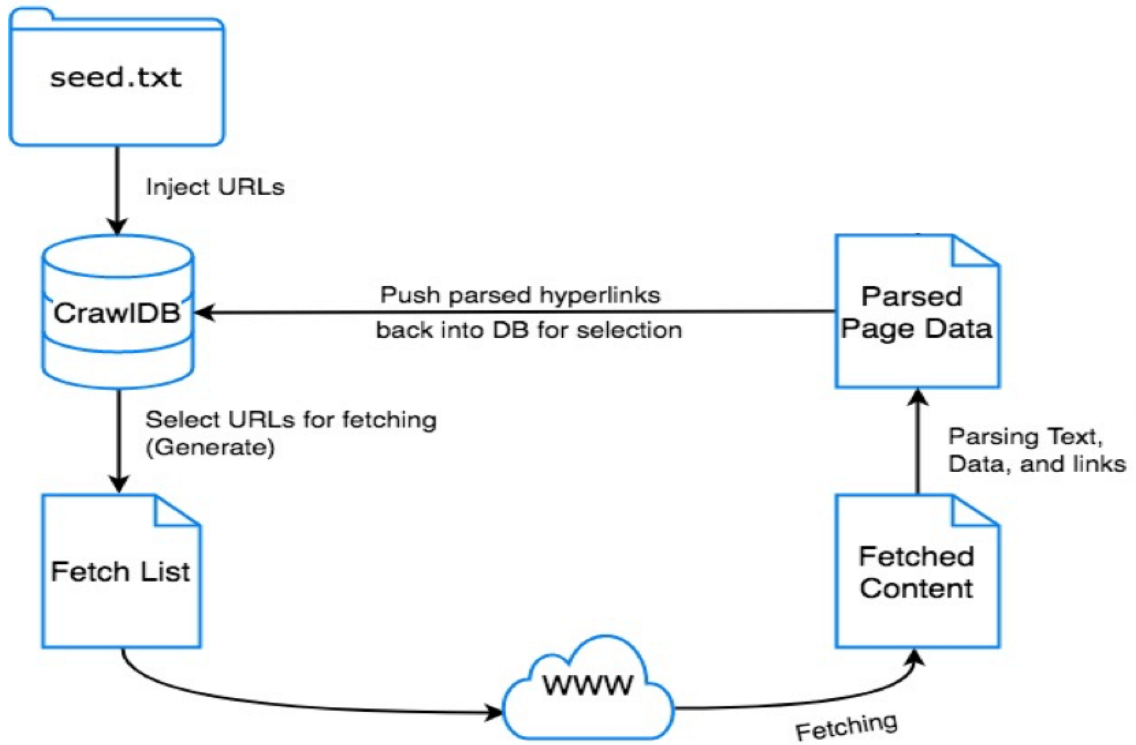
Şekil 3.13 Apache Nutch Çalışma Mimarisi (Anonim, 2017b)
