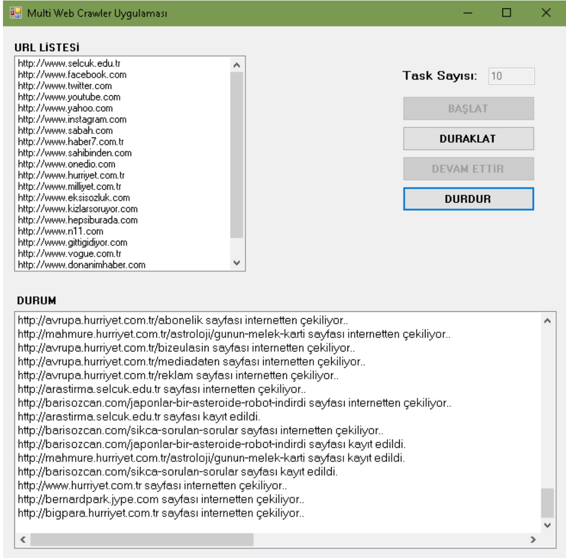
Şekil 4.3 WebCrawler Uygulaması
