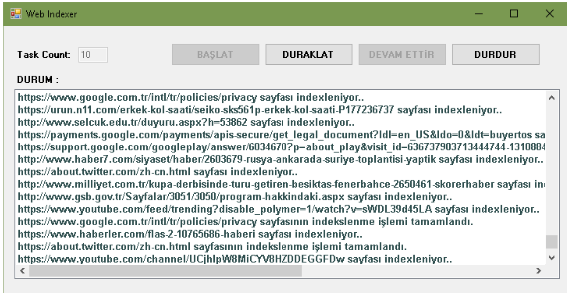
Şekil 4.5 WebIndexer Uygulaması
