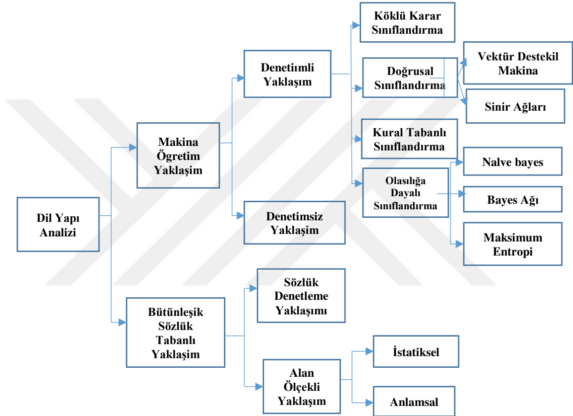
Şekil 2.2. Dil yapı analiz tekniğinin genel yapısı
