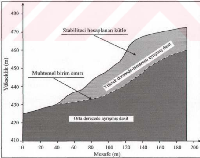
Şekil 51. Stabilité hesaplamalarında kullanılan jeolojik kesit
