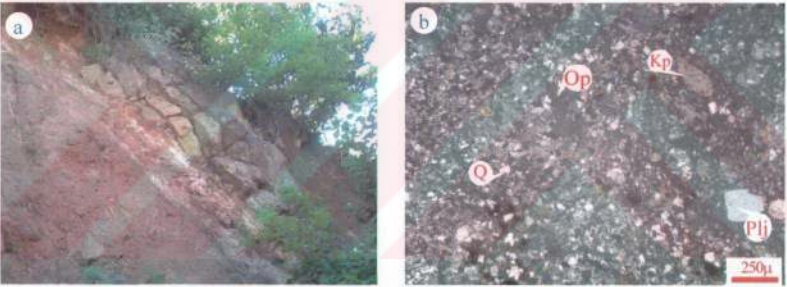
Şekil 15. (a ve b) Hemşindere Formasyonuna ait kumtaşlarının görünüşleri (Ç.N.) (Q: Kuvars, Plj: Plajiyoklas, Kp: Kayaç parçası, Op: Opak)
