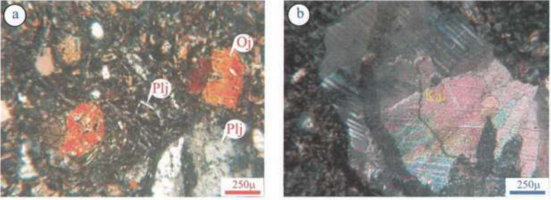
Şekil 8. (a ve b) Bazaltın polarizan mikroskoptaki görünümüleri (Ç.N.) (Plj: Plajiyoklas, Oj: Ojit, Kal: Kalsit)
