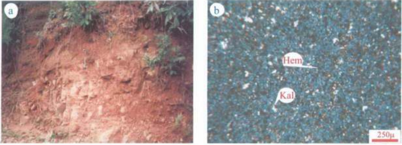
Şekil 14. (a ve b) Hemşindere Formasyonuna ait ince taneli tüflerin görünüşleri (Ç.N.) (Hem: Hematitleşme, Kal: Kalsit)
