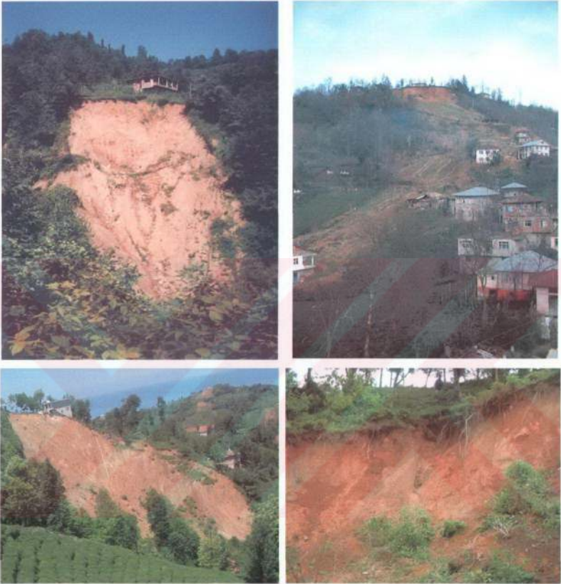
Şekil 34. Çalışma alanında görülen farklı kayma yüzeyli heyelanlar
