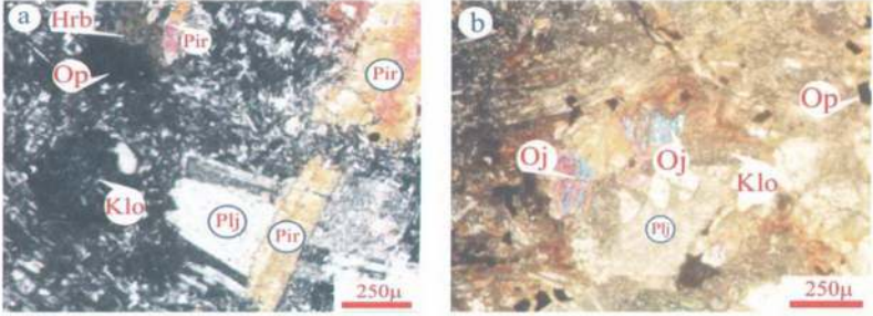
Şekil 7. (a ve b) Hemşidere Formasyonu'na ait andezitlerin polarizan mikroskoptaki görünüşleri (Ç.N.) (Plj: Plajiyoklas, Pir: Piroksen, Klor: Klorit, Hrb: Hornblend, Oj: Ojit, Op: Opak)
