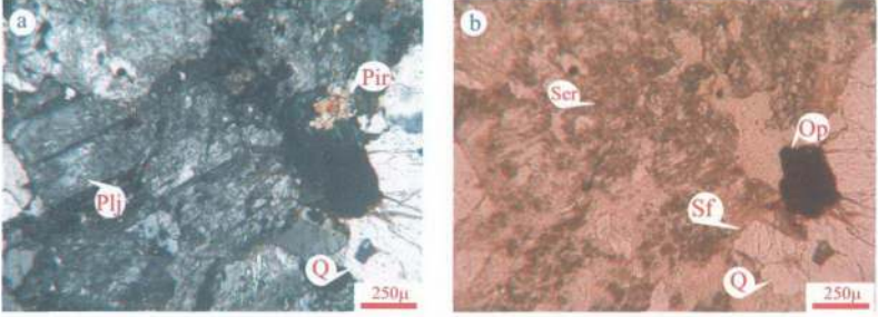
Şekil 21. (a ve b) Tonalitlerin polarizan mikroskobundaki görünimleri (Ç.N. ve T.N.) (Plj: Plajiyoklas, Q: Kuvars, Pir: Piroksen, Ser: Serizitleşme, Sf: Sfen)
