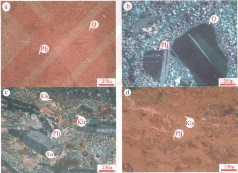
Şekil 12. (a,b,c ve d) Hemşindere Formasyonu'na ait riyoitlerin polarizan mikroskoptaki görünüşleri (Ç.N.) (Plj: Plajiyoklas, Q: Kuvars, Kls: Kalsitleşme, Klr: Kloritleşme, Ser: Serizitleşme, Klo: Klorit)
