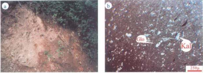
Şekil 17. (a ve b) Hemşindere Formasyonuna ait kireçtaşlarının görünimleri (T.N.) (Kal: Kalsit, Glo: Globotruncana fosili)
