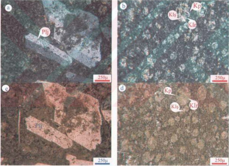
Şekil 9. (a,b,c ve d) Hemşindere Formasyonu'na ait andezitik tüflerin mikroskoptaki görünümüleri (T.N. ve Ç.N.) (Plj: Plajiyoklas, Kp:Kayaç parçası, Kls: Kalsitleşme, Klr: Kloritleşme)
