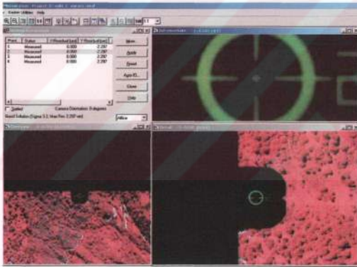
Şekil 27. İç yöneltme işlemi
