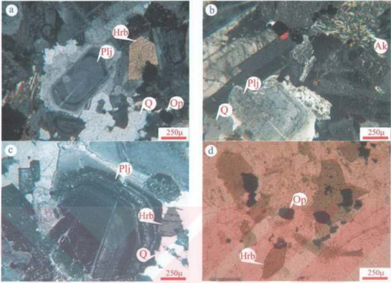
Şekil 19. (a,b,c ve d) Hornblendli kuvarslı diyoritlerin polarizan mikroskobundaki görünüşleri (Ç.N.) (Q: Kuvars, Plj:Plajiyoklas, Hrb: Hornblend, Op: Opak Ak: Aktinolit, Hrb: Hornblend)
