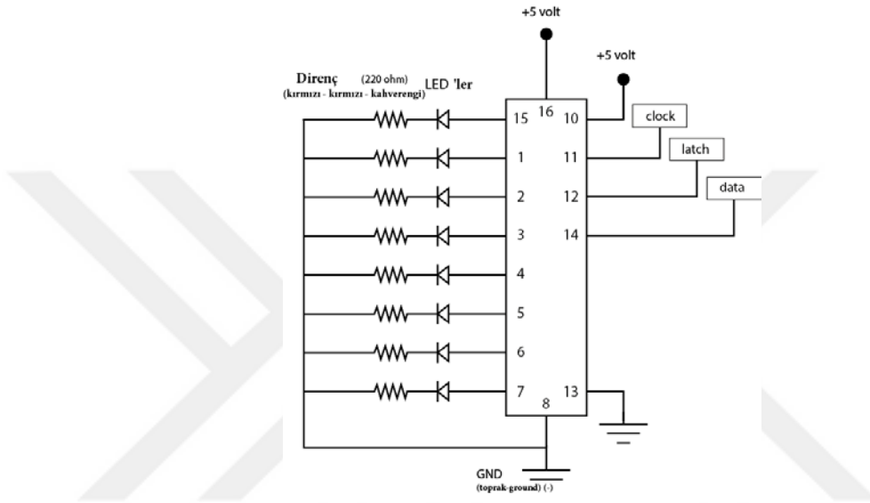
Şekil 29. 74HC595 Şematik Çizimi
