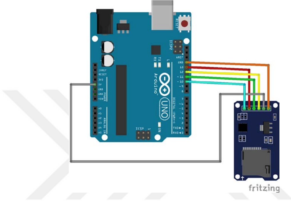
Şekil 27. SD Kart Şematik
