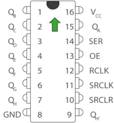
Şekil 28. SN74HC595N
