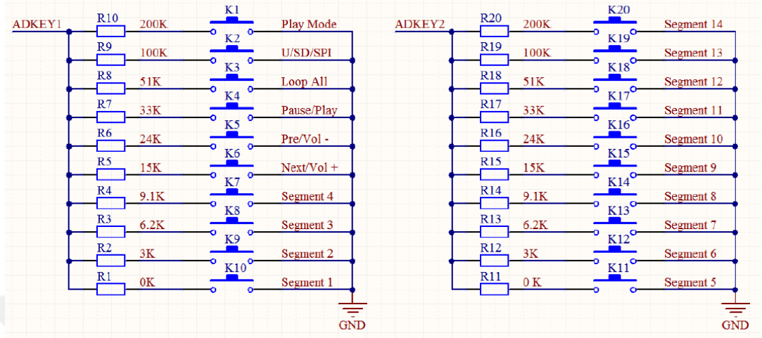
Şekil 24. ADKEY
