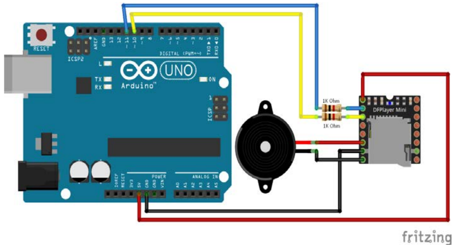
Şekil 25. DFPlayer Bağlantısı
