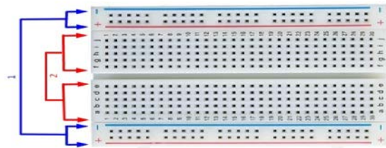
Şekil 22. Breadboard
