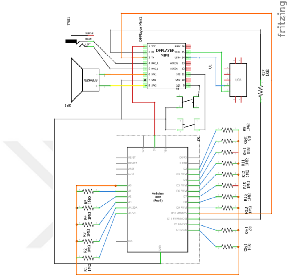
Şekil 63. Dokunmatik Müzik Kutusu Şematik Çizimi
