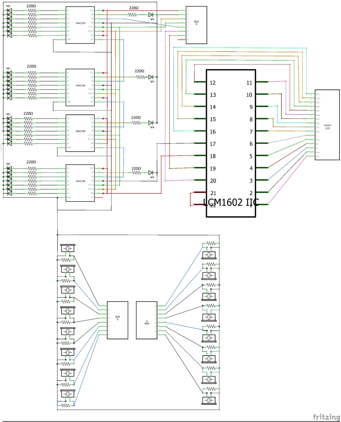
Şekil 72. Melodika ve Müzik Bilgisi Panosu Şematik Çizimi
