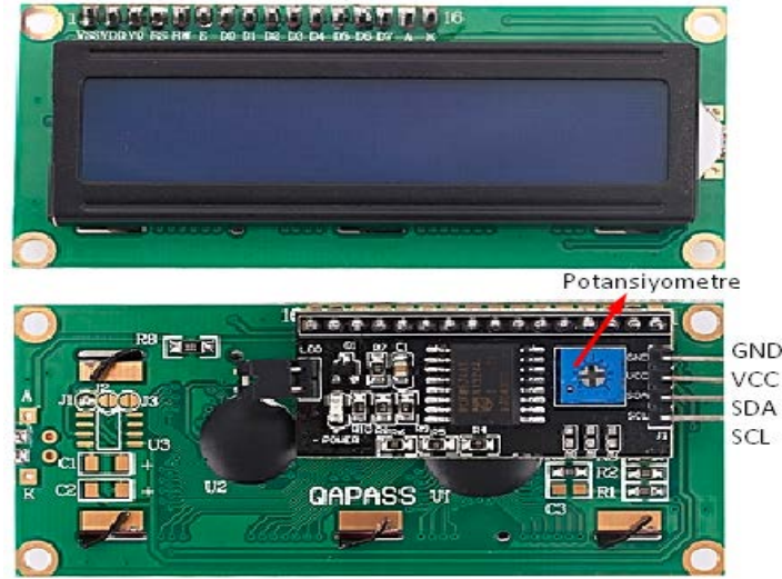
Şekil 31. LCD 1602 I2C
