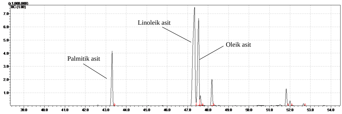
Şekil 4.6. Çörek otu yağına ait GK/KS kromatogramı
