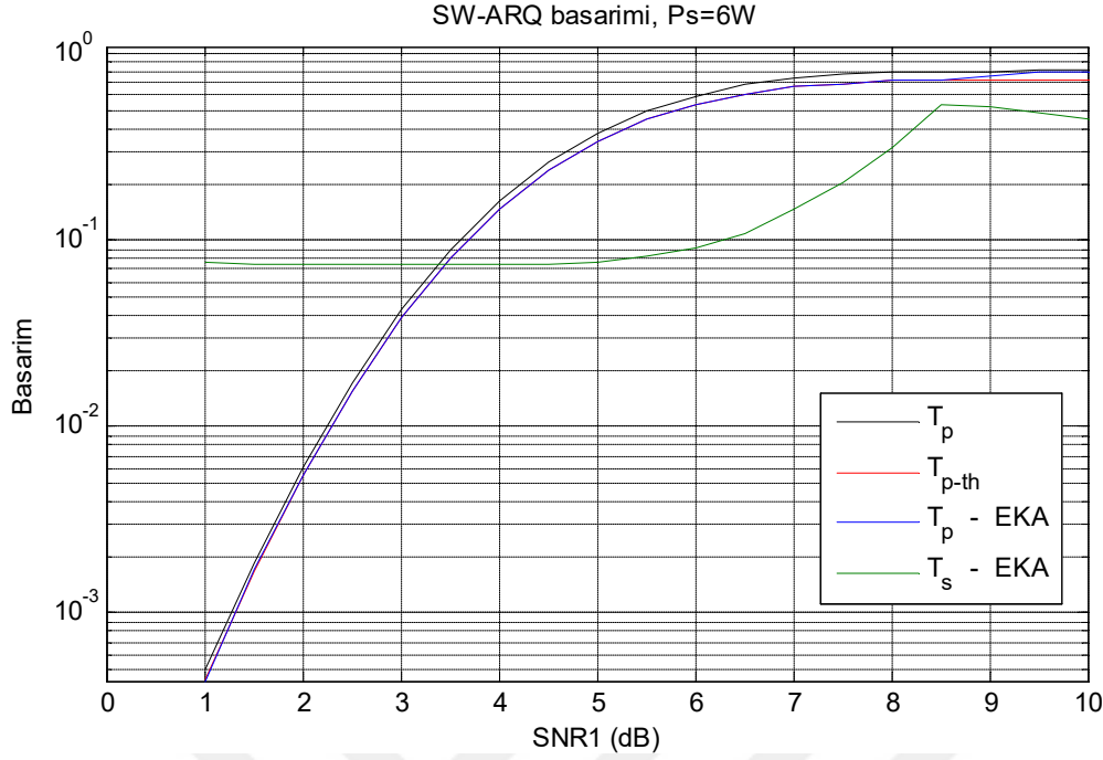
Şekil 4.5. İkincil verici gücü 6 Watt iken SW ARQ birincil ve ikincil başarımları performansları
