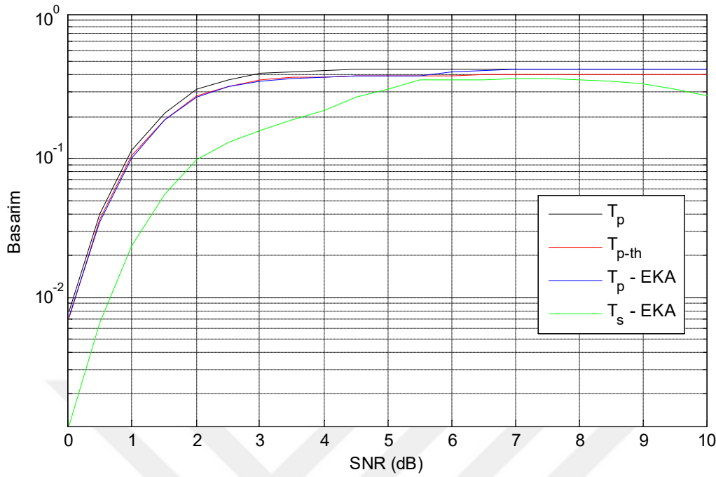
Şekil 4.10. Alt paylaşımlı bilişsel SR HARQ sisteminde birincil ve ikincil kullanıcı başarımları
