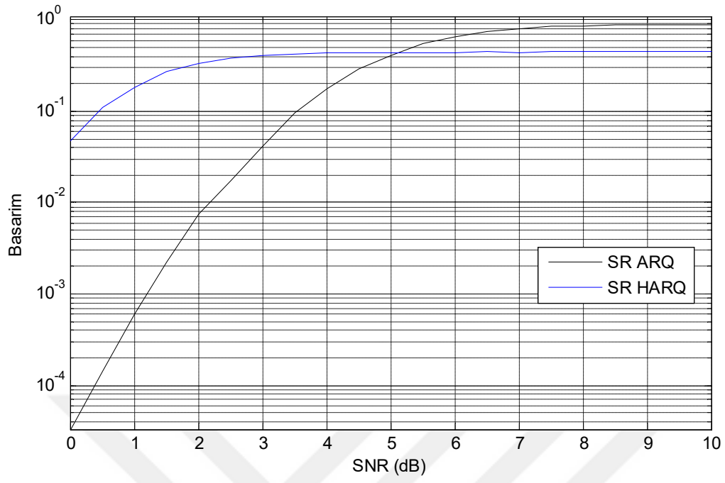
Şekil 2.8. SR ARQ ve SR HARQ sistemlerinin performans kıyaslaması
