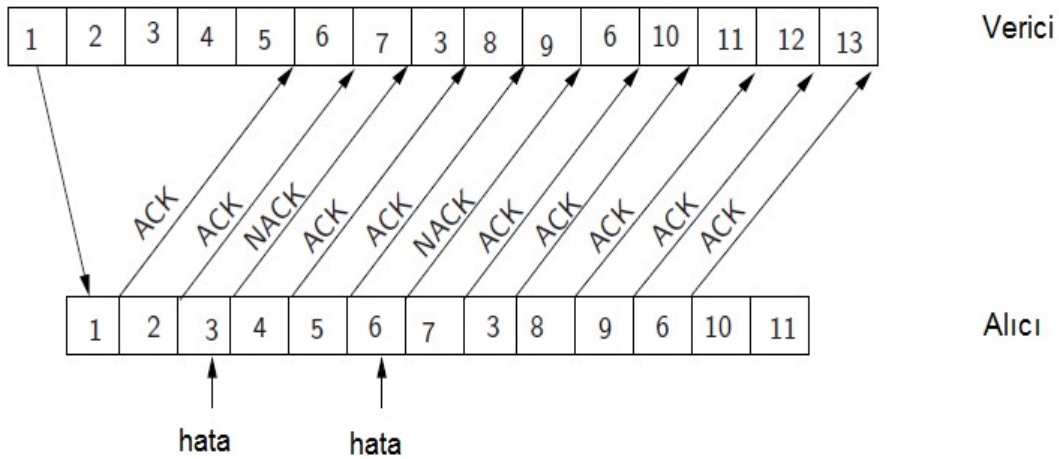
Şekil 2.3. SR ARQ protokolüne bir örnek
