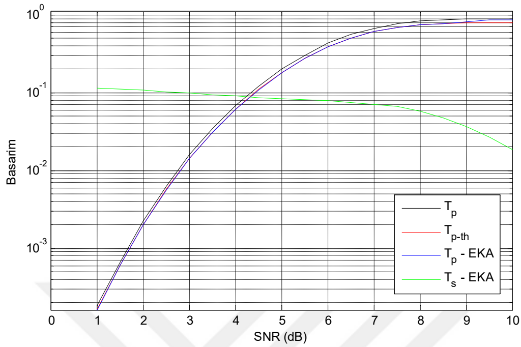
Şekil 4.6. GB-N ARQ birincil ve ikincil başarımları
