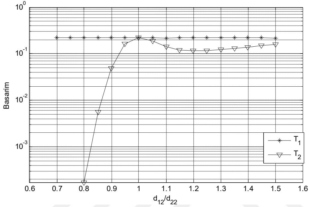
Şekil 4.28. d_{11}=d_{21} ve d_{11}=d_{22} kabulüyle d_{12} ile d_{22} arasındaki ilişkiye göre birincil ve ikincil kullanıcı başarımları
