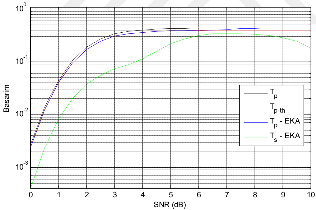
Şekil 4.9. Alt paylaşımlı bilişsel GB-N HARQ sisteminde birincil ve ikincil kullanıcı başarımları
