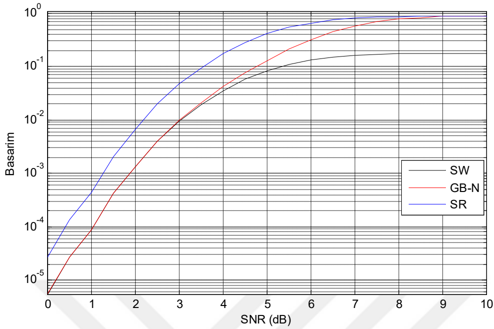
Şekil 2.4. Temel ARQ sistemlerinin performansları
