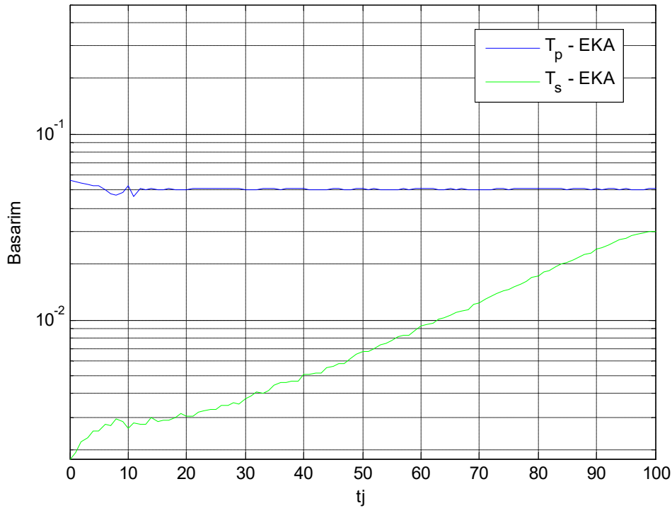
Şekil 4.14. t_{j1} oranına göre birincil ve ikincil kullanıcı başarımların değerleri, SNR=1dB
