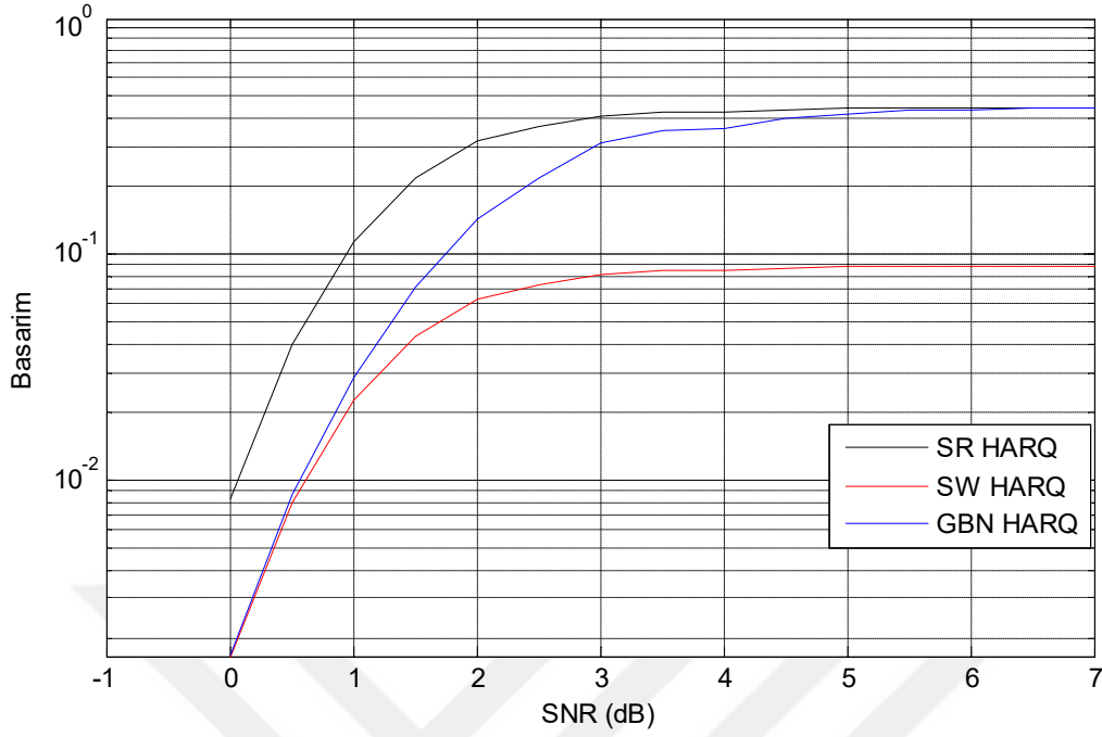
Şekil 2.5. HARQ sistemlerinin performansları
