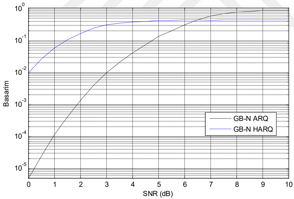
Şekil 2.7. GB-N ARQ ve GB-N HARQ sistemlerinin performans kıyaslaması
