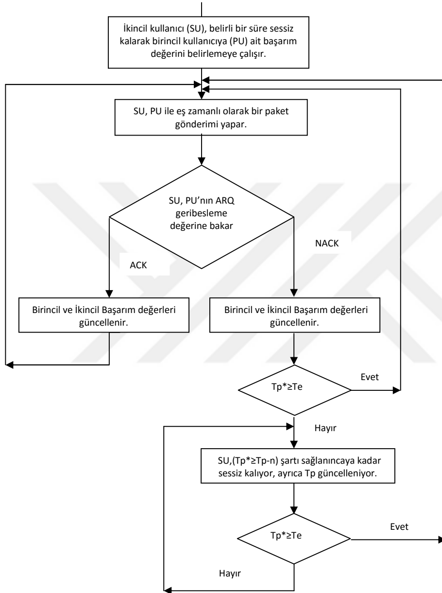
Şekil 4.2. ARQ sistemde Erişim Kontrol Algoritması
