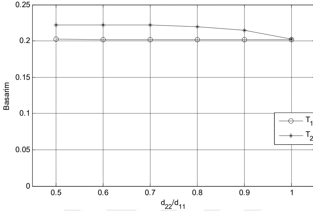
Şekil 4.27. d_{11}=d_{21} ve d_{12}=d_{22} kabulüyle d_{11} ile d_{22} arasındaki ilişkiye göre birincil ve ikincil başarımlar
