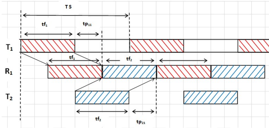
Şekil 4.24. Birincil ve ikincil iletim süresince birincil alıcının durumu
