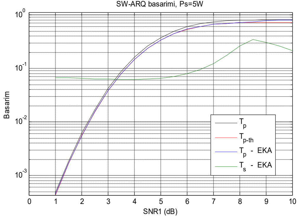
Şekil 4.4. İkincil verici gücü 5Watt iken SW ARQ birincil ve ikincil başarımları
