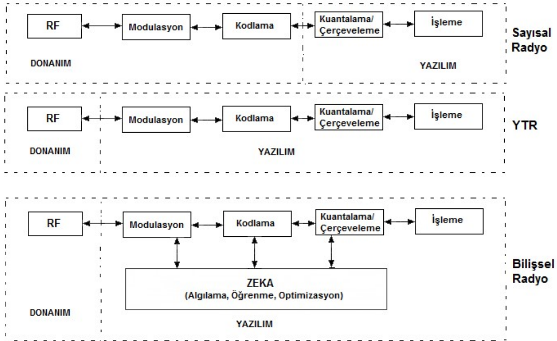
Şekil 3.3. BR gelişim süreci
