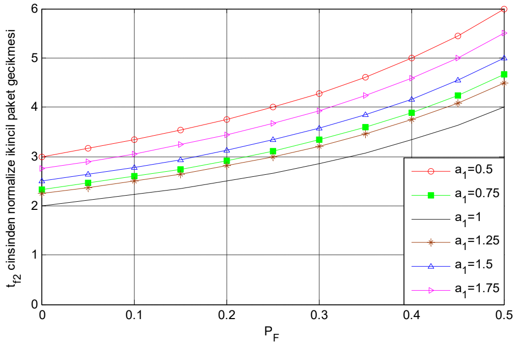
Şekil 4.20. İkincil SW HARQ kullanıcının ortalama gecikme performansı
