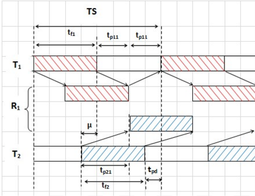
Şekil 4.25. d_{11} , d_{21} ilişkisine bağlı olarak birincil alıcıdaki paket çerçeve düzeni
