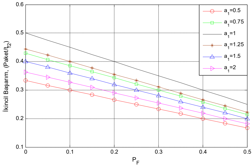
Şekil 4.19. İkincil SW HARQ kullanıcısının başarıım performansı
