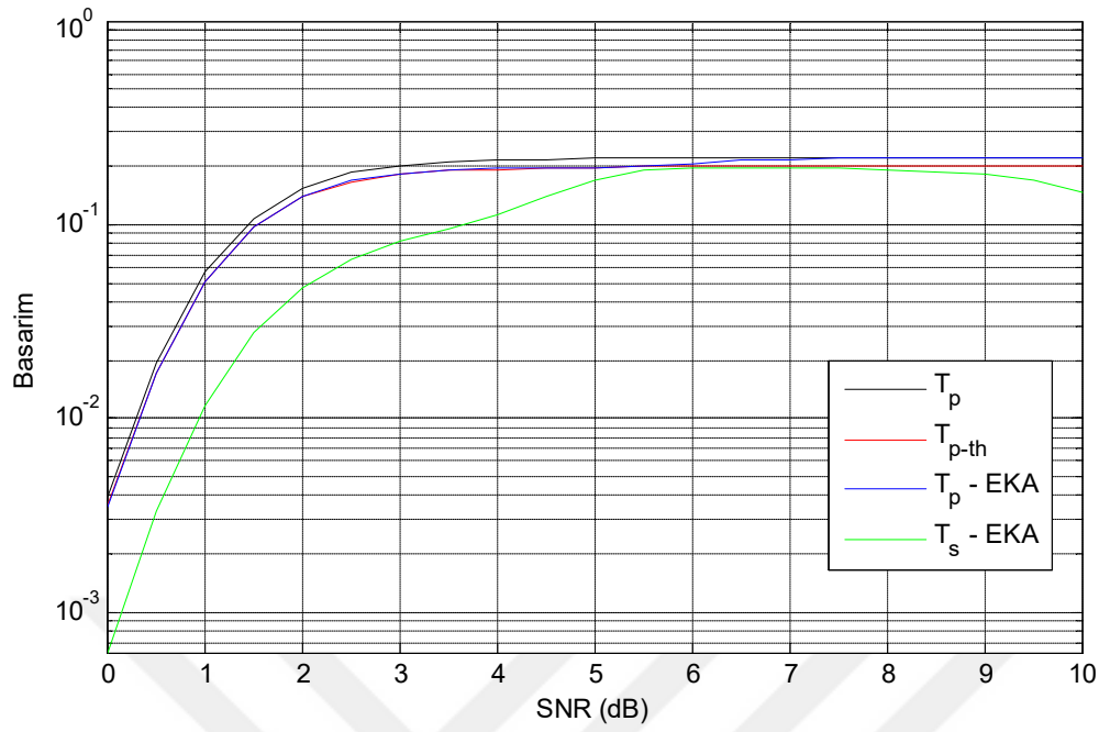
Şekil 4.8. Alt paylaşımlı bilişsel SW HARQ sisteminde birincil ve ikincil kullanıcı başarımları
