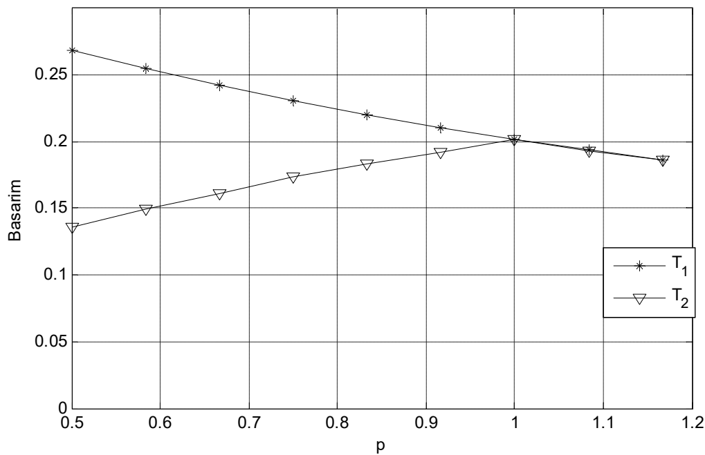
Şekil 4.30. \rho değerine göre birincil ve ikincil başarımların performansları
