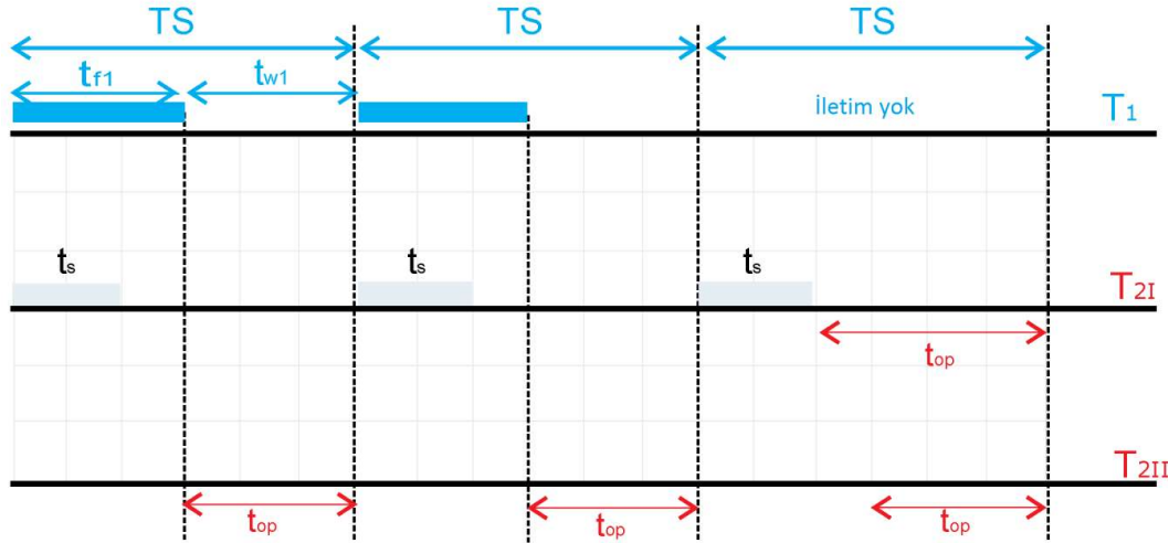
Şekil 4.16. Birincil ve ikincil SW HARQ vericilerinin davranışı
