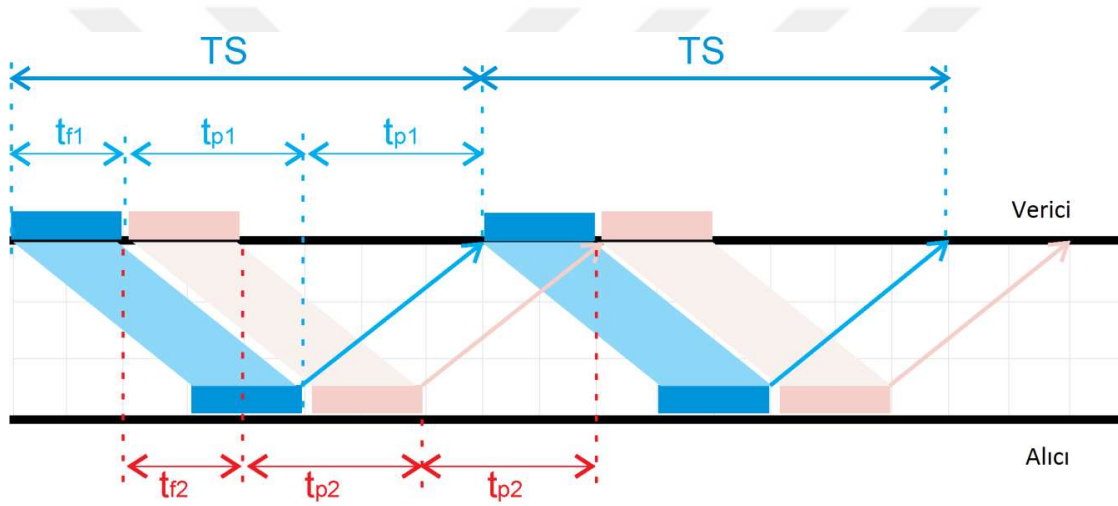
Şekil 4.17. Uzun gecikmeli SW HARQ sisteminin ikincil kullanımı
