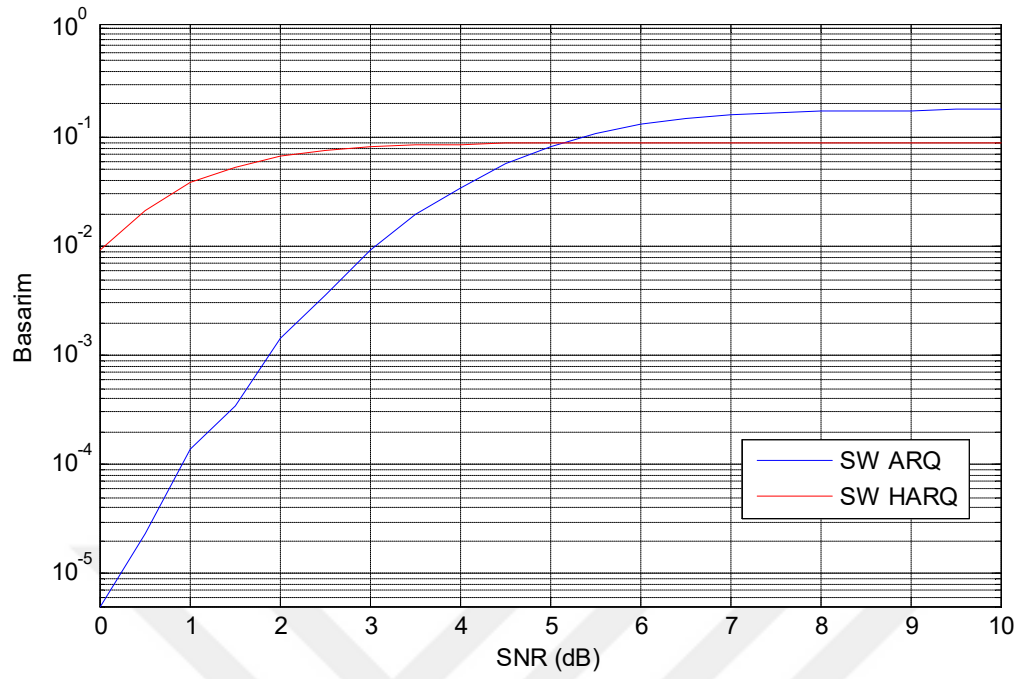
Şekil 2.6. SW ARQ ve SW HARQ sistemlerinin performans kıyaslaması
