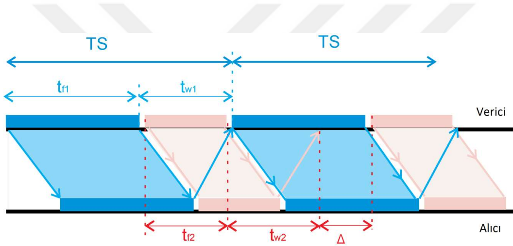
Şekil 4.18. Kısa gecikmeli SW HARQ sisteminin ikincil kullanımı
