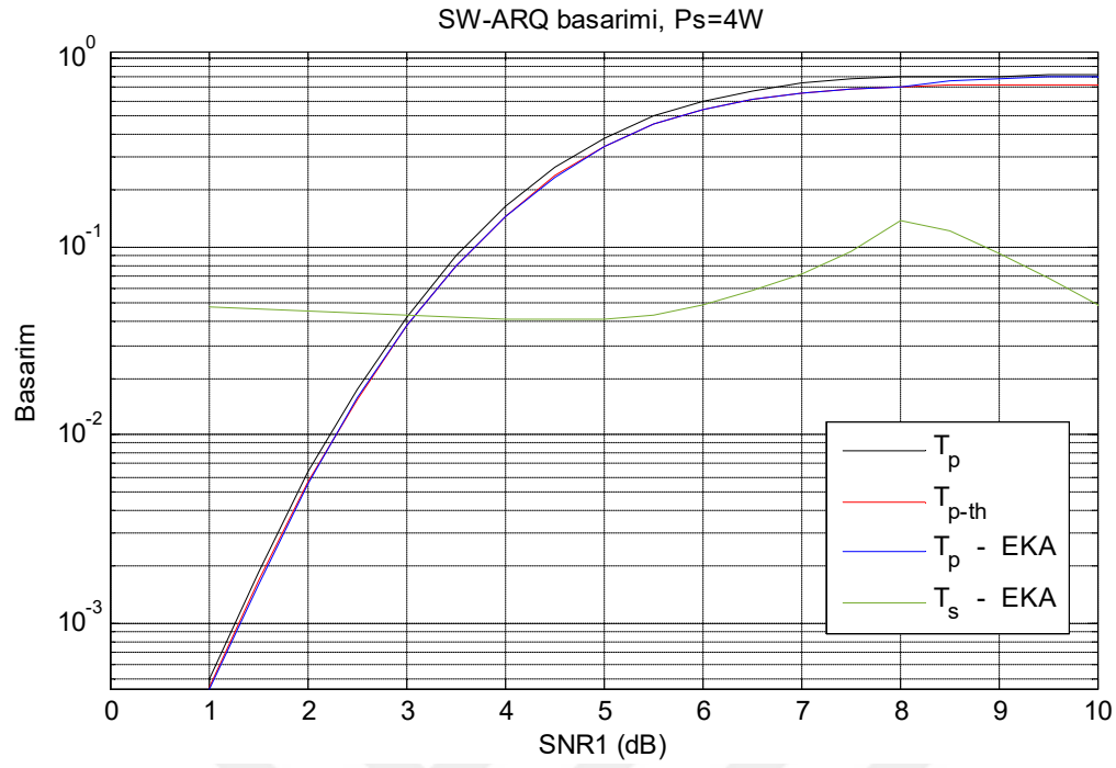
Şekil 4.3. İkincil verici gücü 4Watt iken SW ARQ birincil ve ikincil başarımları
