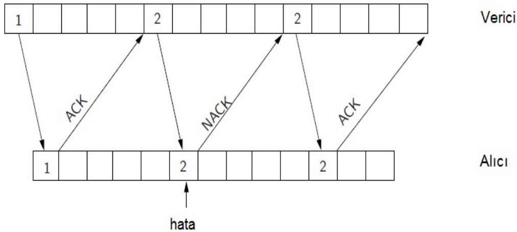
Şekil 2.1. SW ARQ protokolü
