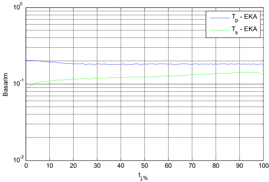
Şekil 4.15. t_{j1} oranına göre birincil ve ikincil kullanıcı başarımlar oranları, SNR=3dB
