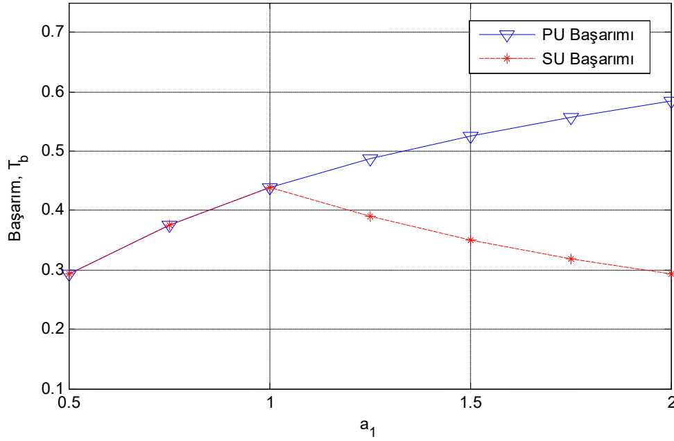
Şekil 4.21. Birincil ve ikincil kullanıcıların uçtan uca bit başarımları
