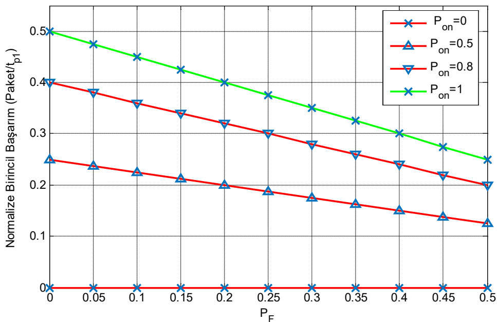
Şekil 4.23. Farklı P_{on} değerleri için birincil başarımları ( a_1=1 )
