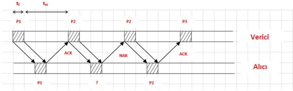
Şekil 4.11. SW HARQ çalışma prensibi
