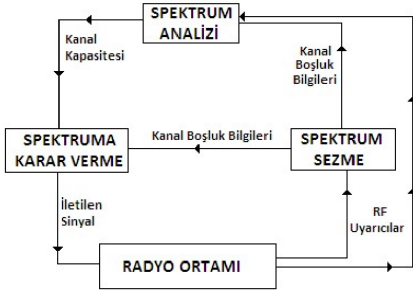
Şekil 3.5. Radyo ortamı için kullanılan genel bilişsel yöntem
