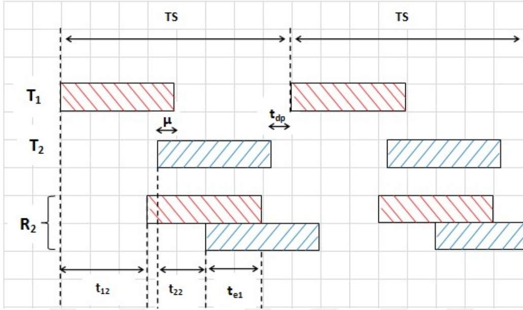
Şekil 4.26. d_{11} > d_{21} ve d_{12} > d_{22} durumlarında ikincil alıcıda paket çerçeve düzeni
