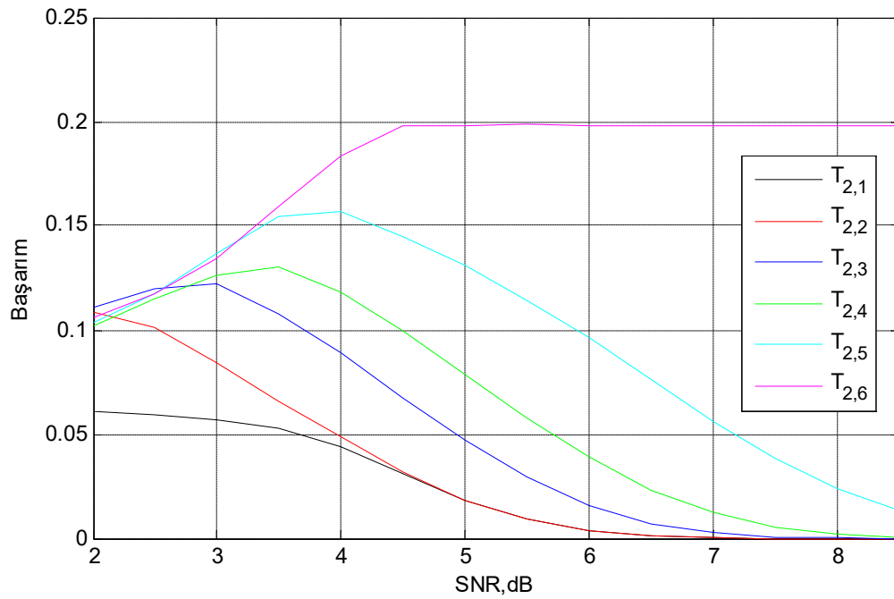
Şekil 4.13. Farklı t_i sürelerini esas alan SU'ların SNR-Başarım performansı
