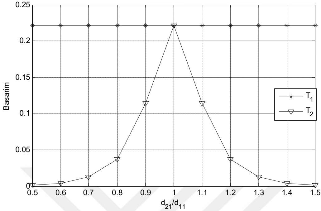
Şekil 4.29. d_{11}=d_{22} ve d_{12}=d_{22} kabulüyle d_{21} ile d_{11} arasındaki ilişkiye göre birincil ve SU başarımları
