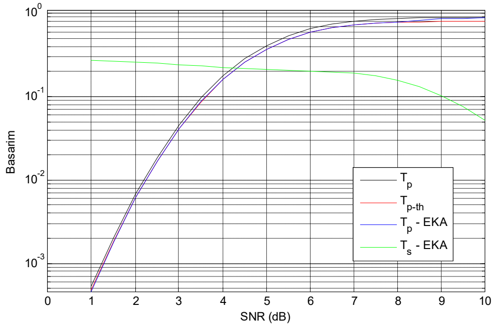
Şekil 4.7. SR ARQ birincil ve ikincil başarımları
