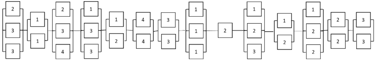
Şekil 5.2 P22 problemi için tamir edilen bileşenlerin yer aldığı örnek sistem tasarımı
