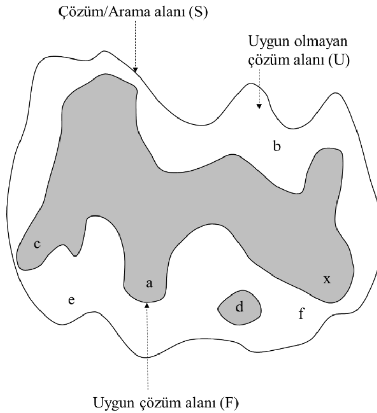
Şekil 4.8. Bir çözüm alanı/arama uzayı örneği [117]
