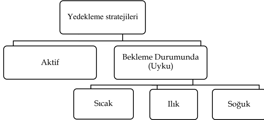
Şekil 2.4.Yedekleme stratejileri seçenekleri
