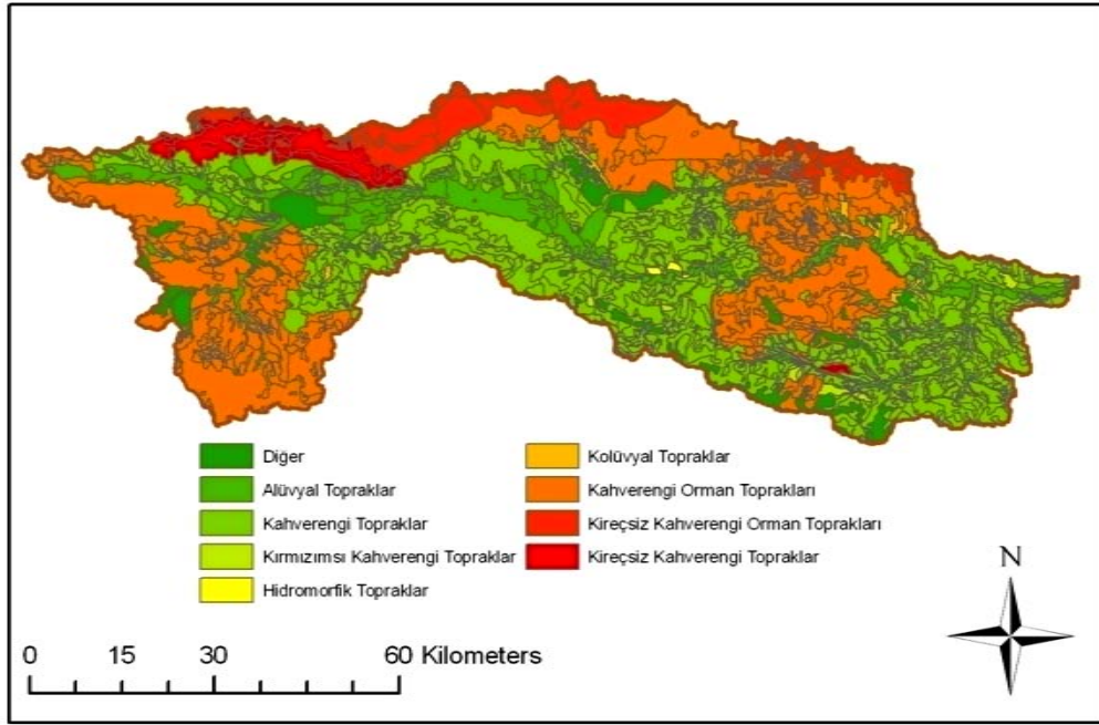
Şekil 6.2. Çalışma alanı büyük toprak grupları (KHGM, 2009)
