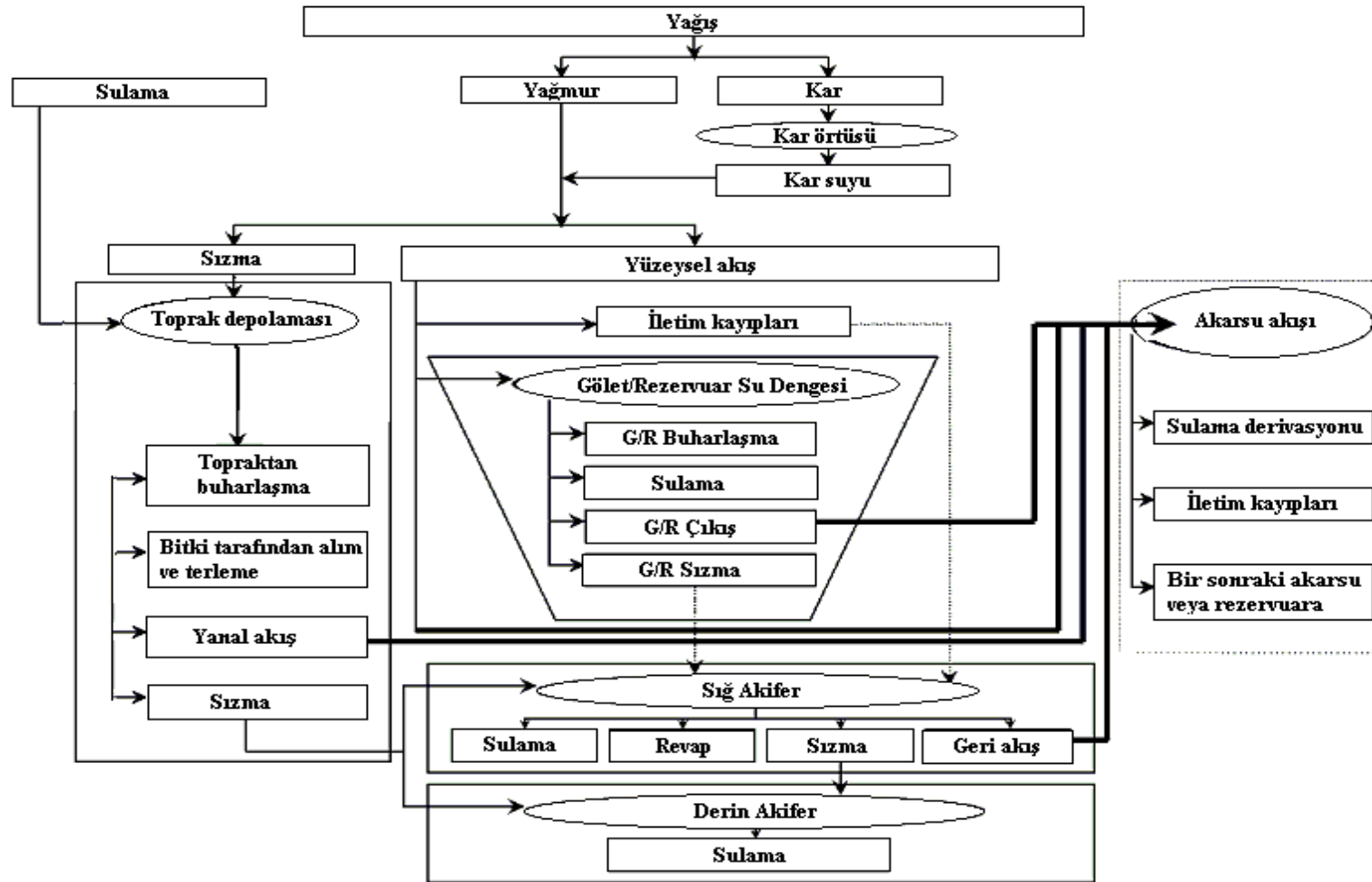
Şekil 4.1. SWAT modelindeki su hareketinin şematik gösteri
