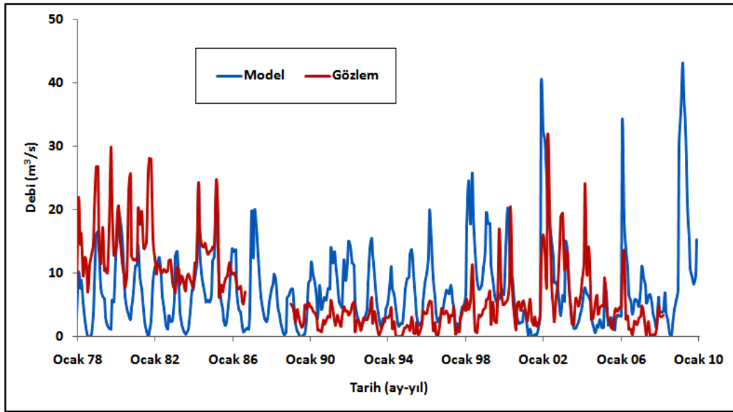
Şekil 8.9. Kıranharmanı ve Sazılar istasyonu için aylık model ve gözlem sonuçları
