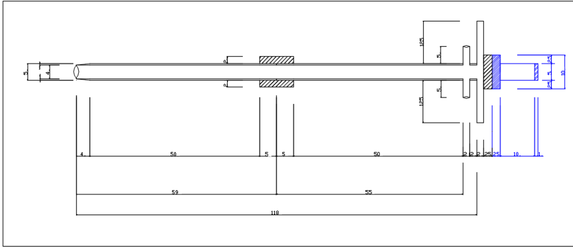
Şekil 3.4. Dip Sediment Örneklemme Aparatı (birimler cm cinsindendir)
