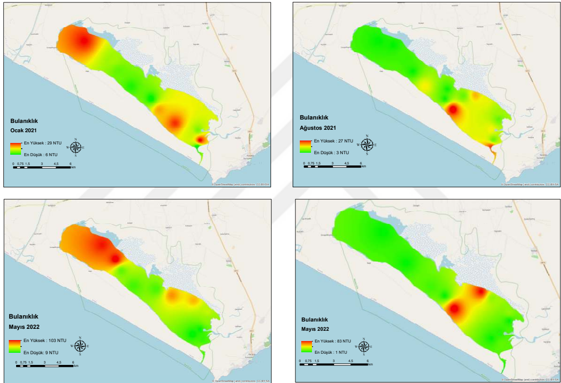
Şekil 4.87. Akçayan lagününde bulanıklık değişiminin CBS ile tahmini
