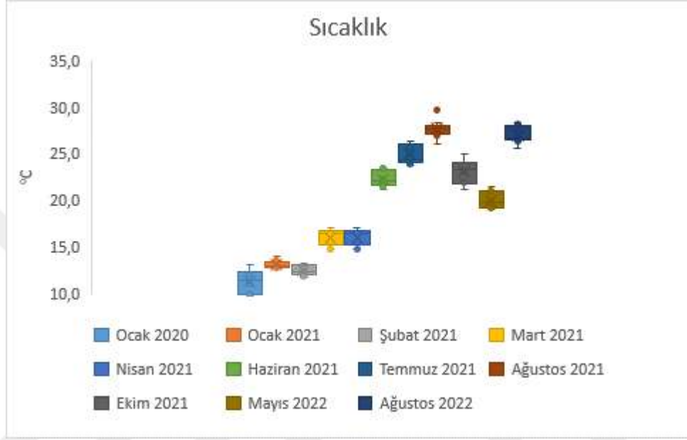
Şekil 4.102. YD3 drenaj kanalında sıcaklık değişimi
