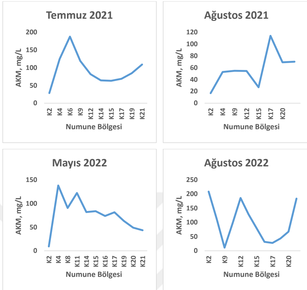
Şekil 4.107. YD3 drenaj kanalında aylara göre AKM değişimleri
