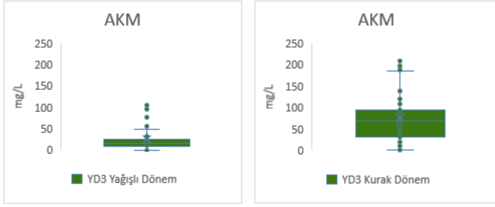
Şekil 4.136. YD3 drenaj kanalında su kalitesinin yağışlı ve kurak dönemlere göre AKM değişimlerinin incelenmesi
