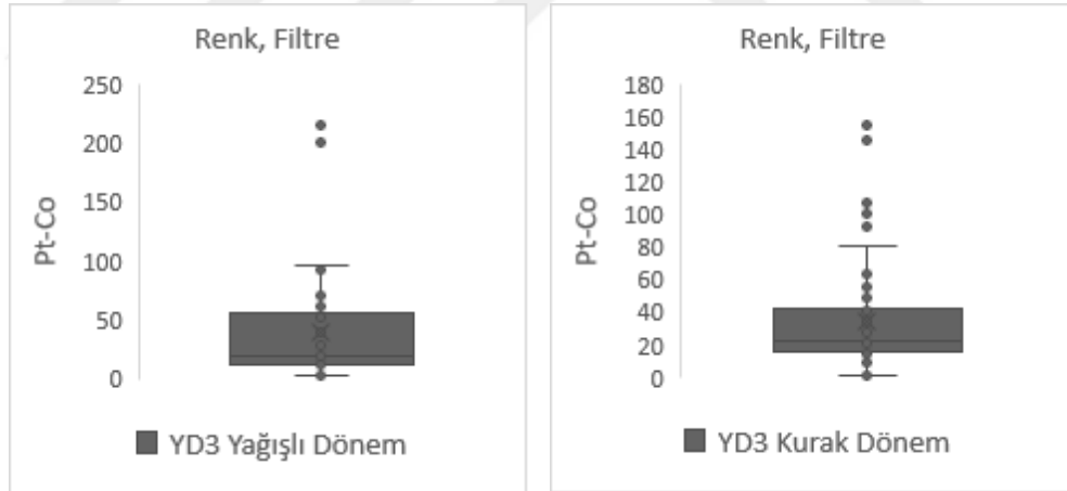
Şekil 4.142. YD3 drenaj kanalında su kalitesinin yağışlı ve kurak dönemlere göre Renk (filtrasyon işlemi sonrasında) değişimlerinin incelenmesi
