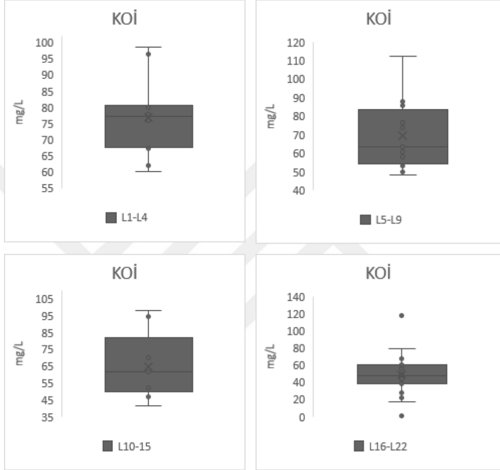
Şekil 4.51. Akyatan lagününde alansal KOİ değişimlerinin incelenmesi
