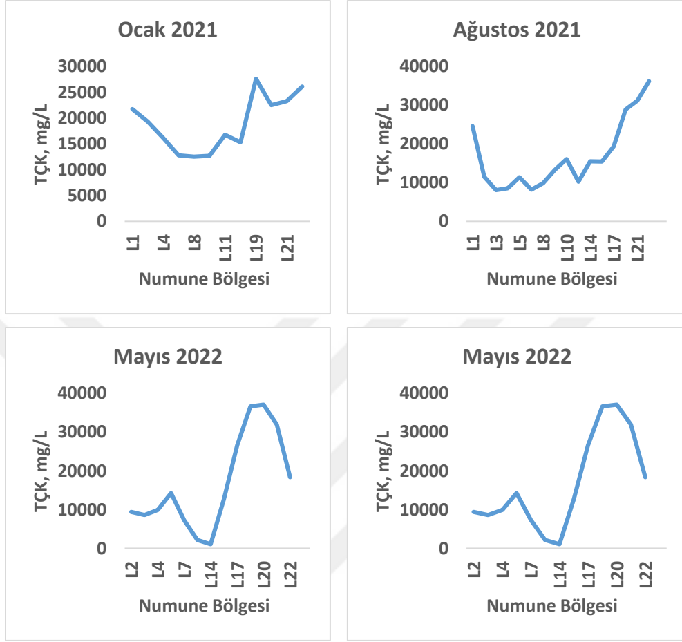
Şekil 4.12. Aylara göre TÇK değişimleri
