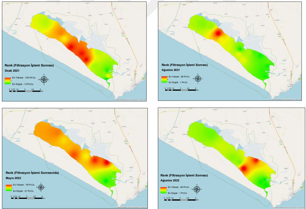
Şekil 4.86. Akyatan lagününde renk (filtrasyon işlemi sonrasında) değişiminin CBS ile tahmini
