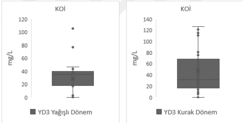
Şekil 4.137. YD3 drenaj kanalında su kalitesinin yağışlı ve kurak dönemlere göre KOİ değişimlerinin incelenmesi
