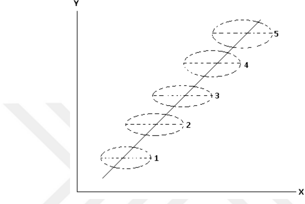
Şekil 1: Heterojen Sabit Parametre ve Homojen Eğim Parametre Durumu
