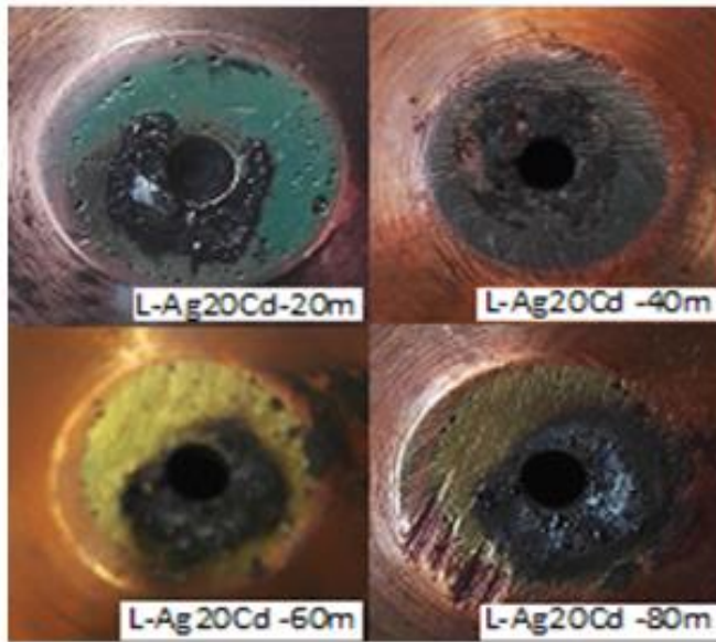
řekil 4.4. L-20AgP doldurulan nozul yüzeyindeki erozyon
