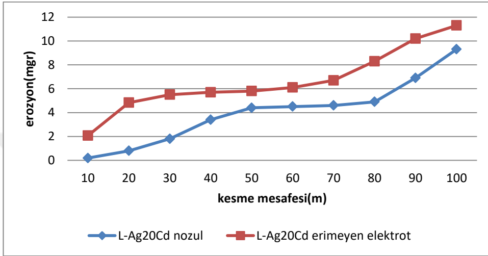
řekil 4.3. Erimeyen Elektrot ve L-20AgP doldurulan nozulda erozyon hızı
