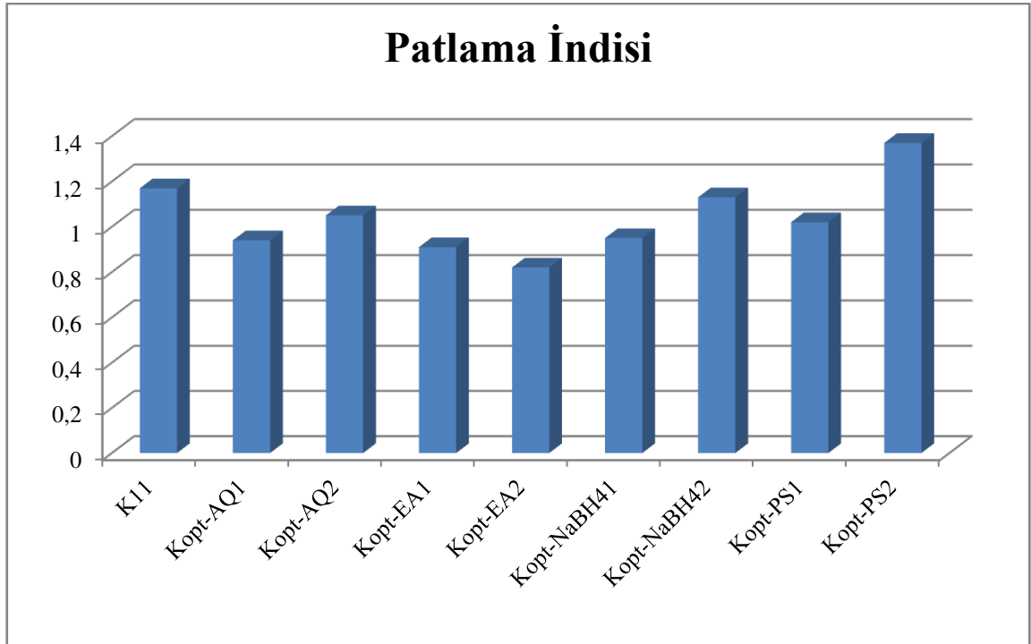
Şekil 4.7 Aspir saptarından 3. kademe dövme derecesinden elde edilen kağıtlarda optimum pişirme koşulu ile modifiyeli kağıtlar arasındaki patlama indisi arasındaki ilişki
