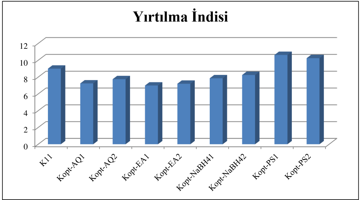
Şekil 4.8 Aspir saplarından 3. kademe dövme derecesinden elde edilen kağıtlarda optimum pişirme koşulu ile modifiyeli kağıtlar arasındaki yırtılma indisi arasındaki ilişki
