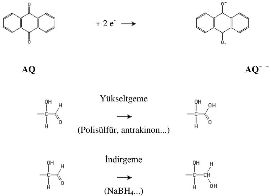
Şekil 2.10: Antrakinon Oksidasyonu, Antrakinonun ve Sodyum borhidrür'ün Yükseltgeme ve İndirgenme reaksiyonları
