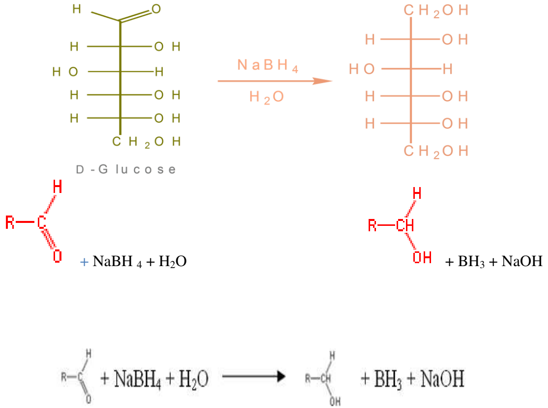
Şekil 2.8: \text{NaBH}_4 'ün Aldehit Keton Gruplarını Hidroksil Grubuna İndirgeme Reaksiyonu
