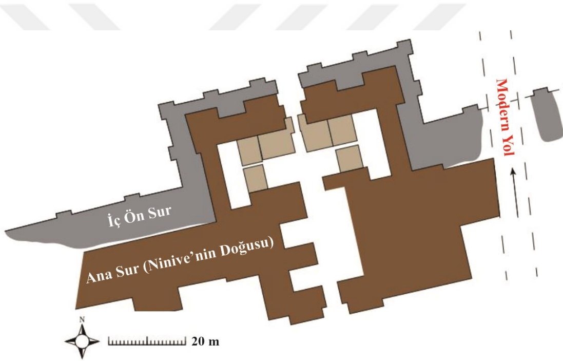
Şekil 4.36: Mullisu Kapısı'nın planı (Sollee, 2020, Abb. 107)
