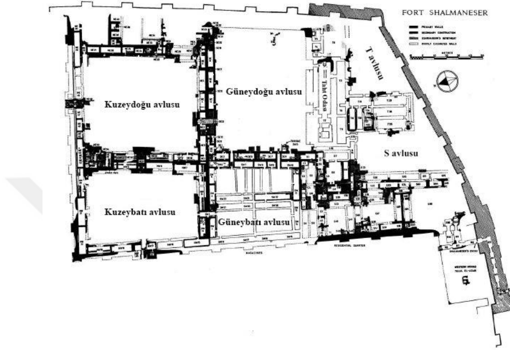
Şekil 4.41: Kalhu'daki ekal māšarti 'nin planı (Mallowan, 1966, Plan VIII)
