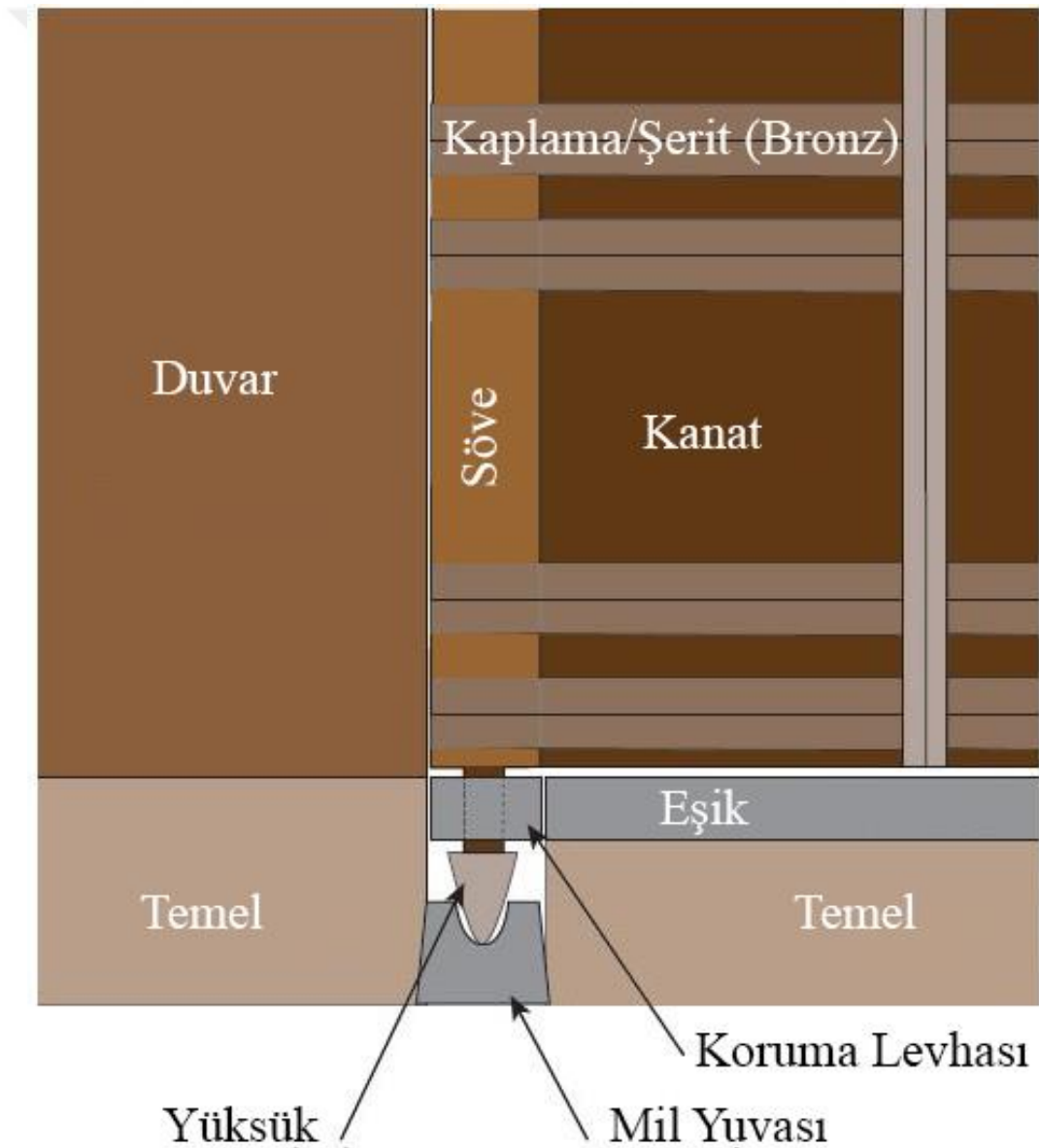
Şekil 4.52: Yeni Assur Dönemi kapılarının bileşenlerini gösteren rekonstrüksiyon çalışması (Sollee, 2020, Abb.157)
