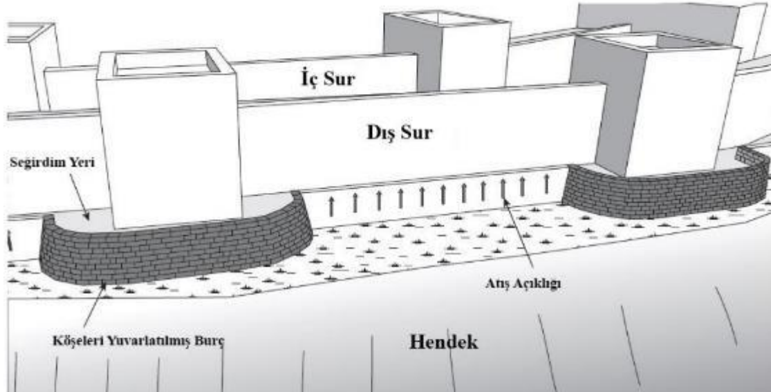
Şekil 4.20: Kule 13-15'in karşısındaki dış sura bağlı kule, burç ve siperlerin rekonstrüksiyonu (Sollee, 2020, Abb. 48)
