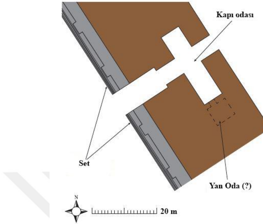
Şekil 4.83: Maški Kapısı'nın planı (Sollee, 2020, Abb. 114)
