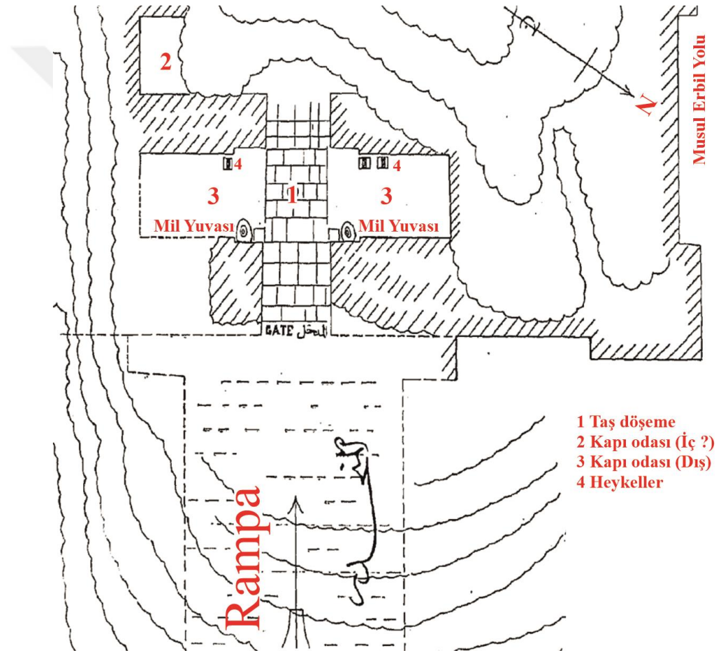
Şekil 5.48: 1954 yılında kazılan kapı yapısının şematik planı (Aslına bağlı kalarak düzenlemelerde bulunulmuştur, al-Asil, 1954, Fig. 1)
