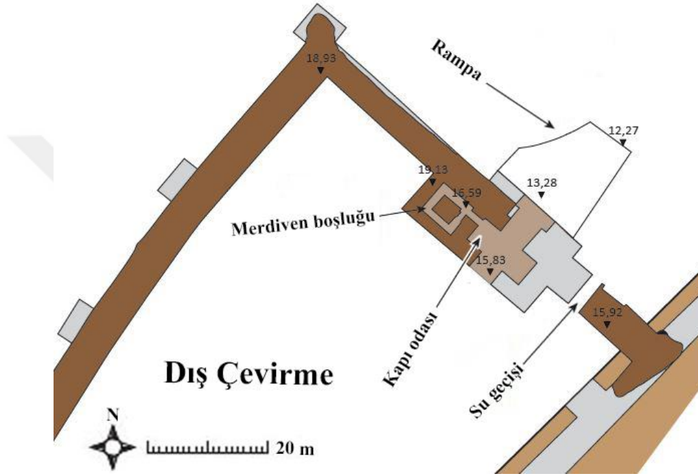
Şekil 4.55: Dış çevirme üzerinde yer alan Aşağı Kapı (Sollee, 2020, Abb. 11)
