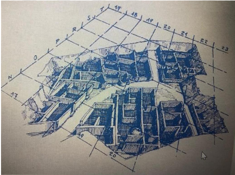
Resim 13: II. kat mahallerinin perspektif rekonstrüksiyonları. 44
