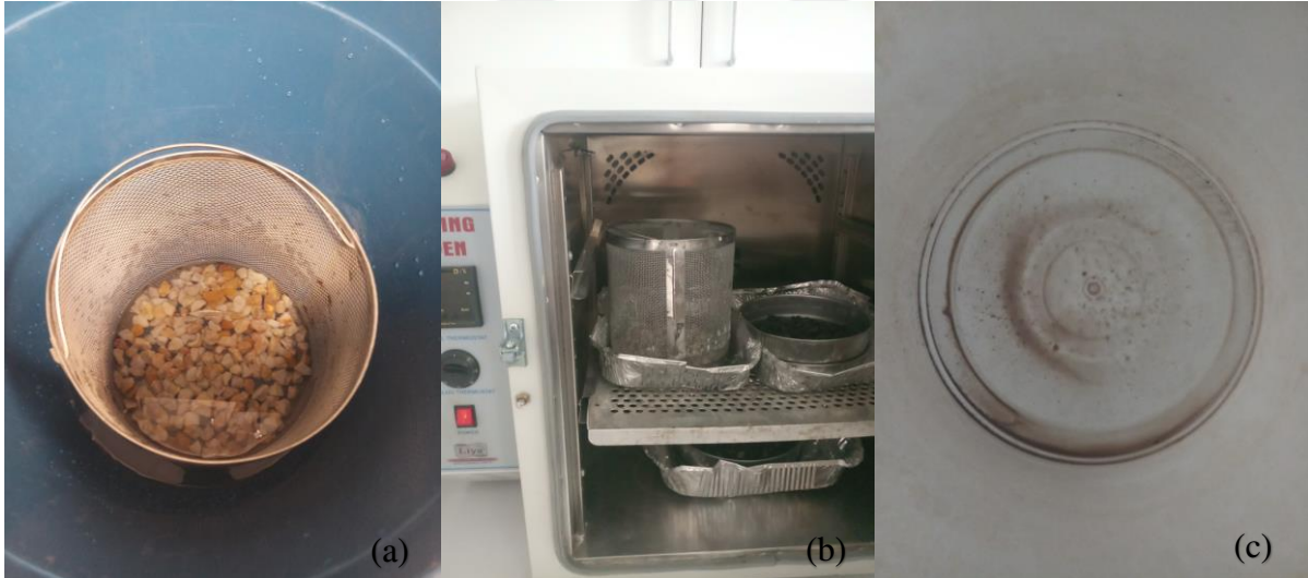
Şekil 4.6. Kimyasal donma çözülme deneyi, a) Tel sepet içinde çözeltide bekletilen numune, b) Numunenin etüvde bekletilmesi, c) Donma çözülme sonucu oluşan kayıp
