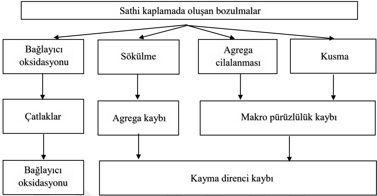
Şekil 2.6. Sathi kaplamada meydana gelen bozulma modeli
