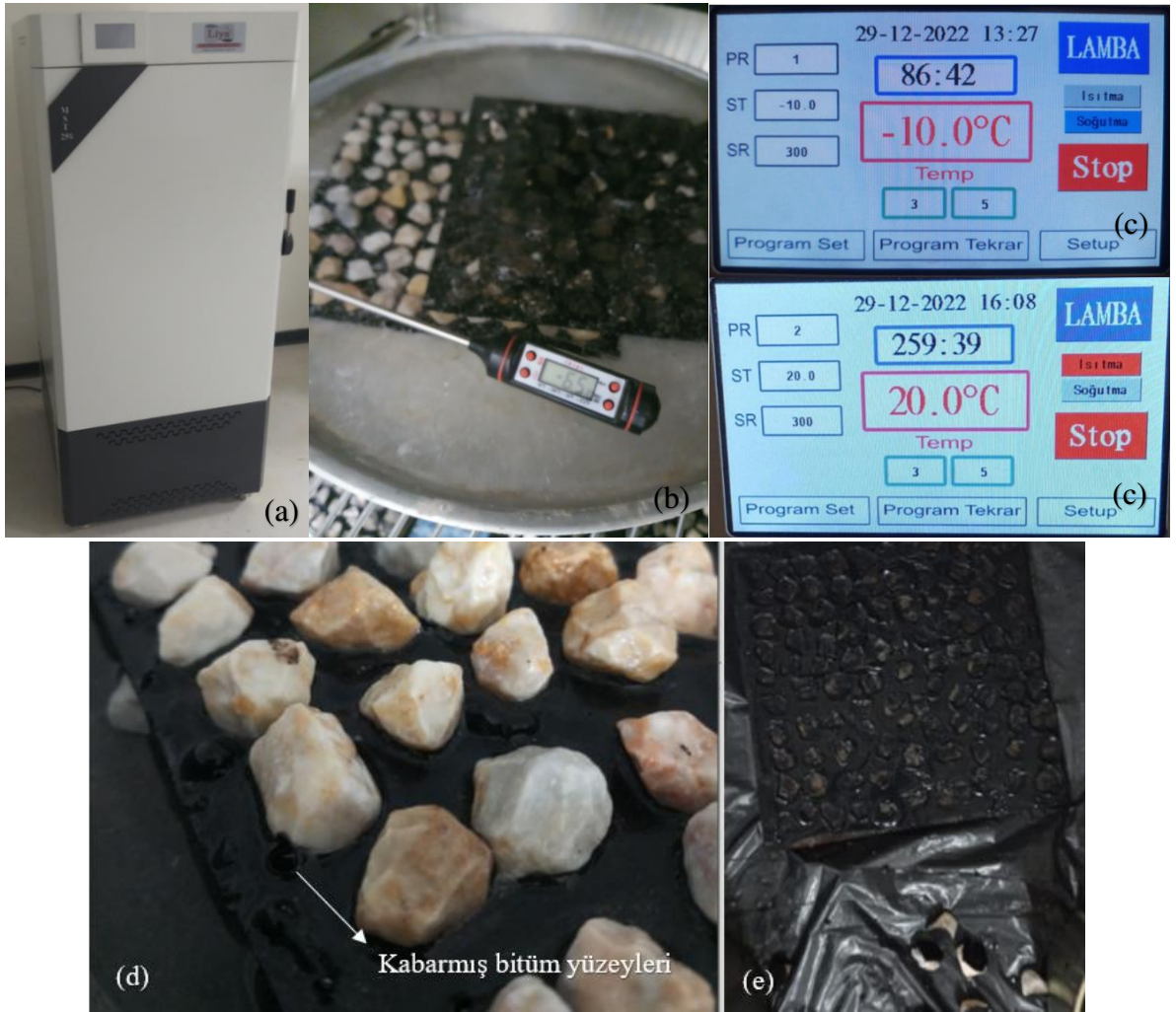
Şekil 4.12. Modifiye vialit deneyi, (a) İklimlendirme kabini, (b) Eksi sıcaklıkta numuneler, (c) İklimlendirme kabinine girilen program, (d) Kabarmış yüzeyler, (e) Eksi sıcaklıkta plakadan tamamen düşen agregalar
