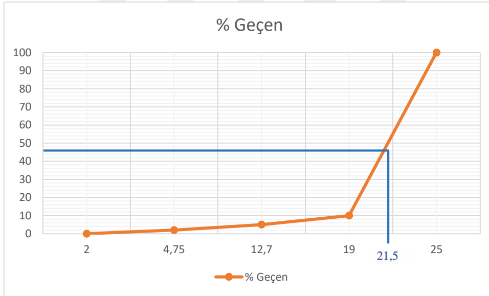
Grafik 2.4. Dane dağılımı grafiğinden OB bulunması
