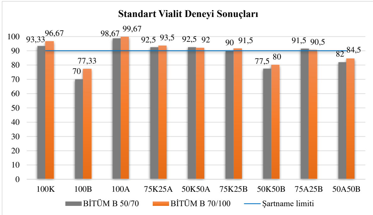
Grafik 5.5. Standart vialit deneyi sonuçları
