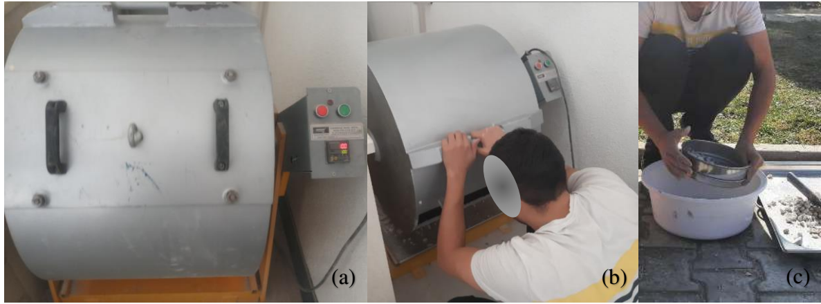
Şekil 4.2. Los Angeles deneyi, a) Los Angeles deney aleti, b) Deney numunelerinin cihaz içerisinden alınması, c) Deney sonunda agrega numunesinin 1,6 mm elekten elenmesi
