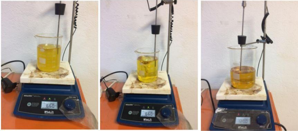
Resim 5.6 Biyodizelin ısıtılması.
