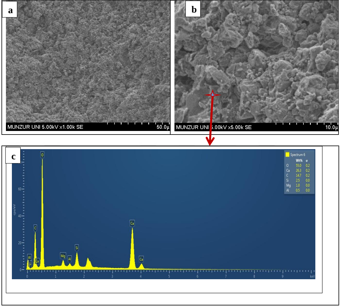
Şekil 3.12. Mardin taşı partiküllerinin (a) 100 k ve (b) 500 k büyütmelelerdeki morfolojisi (c) EDX
