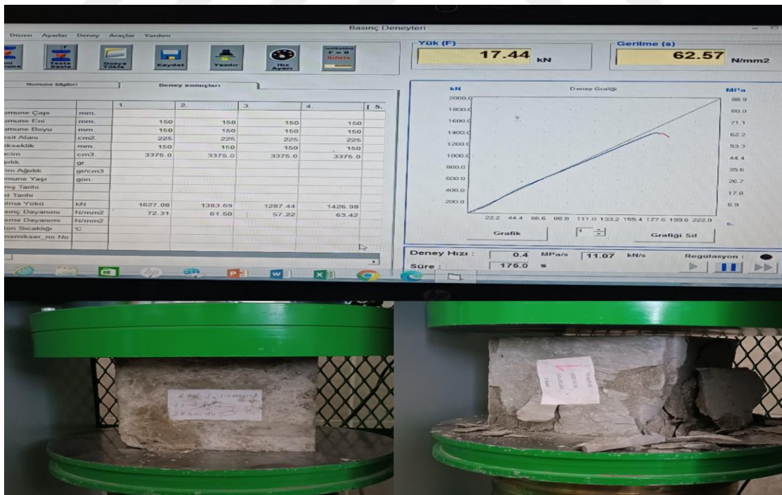
Şekil 0.4. Basınç numunesi ve cihazı
