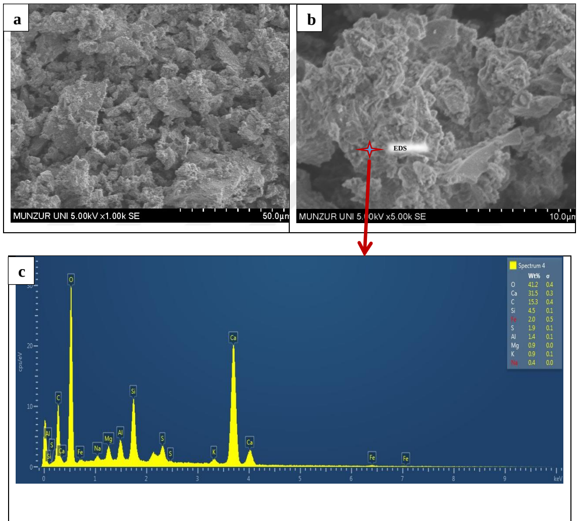
Şekil 3.11. Çimento (CEM II/A-LL 42.5 R) partiküllerinin (a) 100 k ve (b) 500 k büyütme (c) EDX
