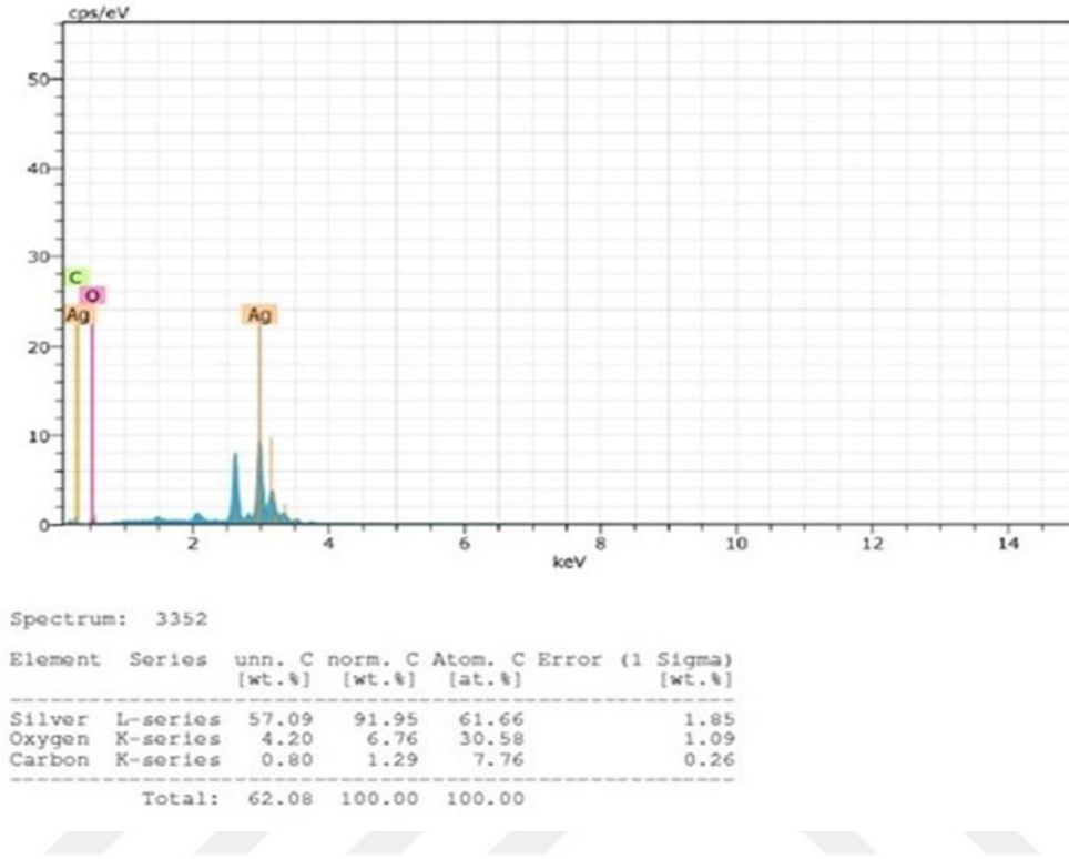
Şekil 4.8. AgNPs EDX Spektrumu Ve Elementel Yüzdeleri
