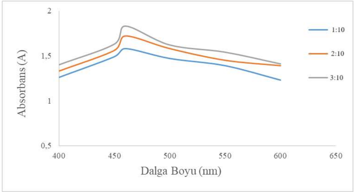
Grafik 4.2. En Uygun Özütleme Oranı
