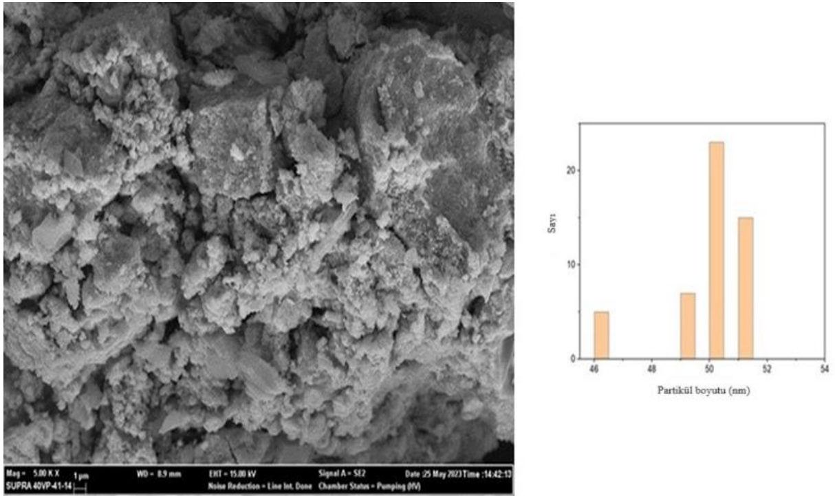
Şekil 4.7. AgNPs SEM Görüntüsü ve Histogramı
