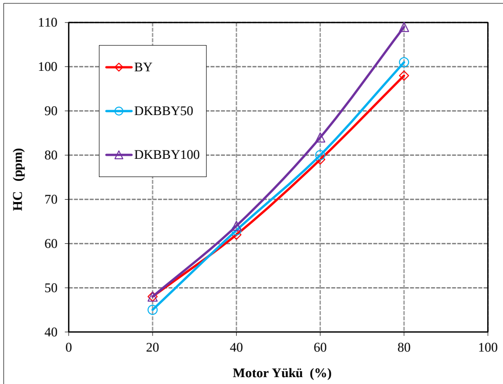
Şekil 10.16. BY, DKBBY50 ve DKBBY100 yakıtlarının değişken yükteki HC emisyonu değerleri
