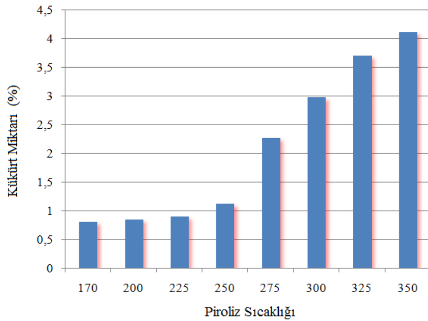
Şekil 8.10. Reaksiyon sıcaklığının dizel benzeri yakıttaki kükürt içeriğine etkisi
