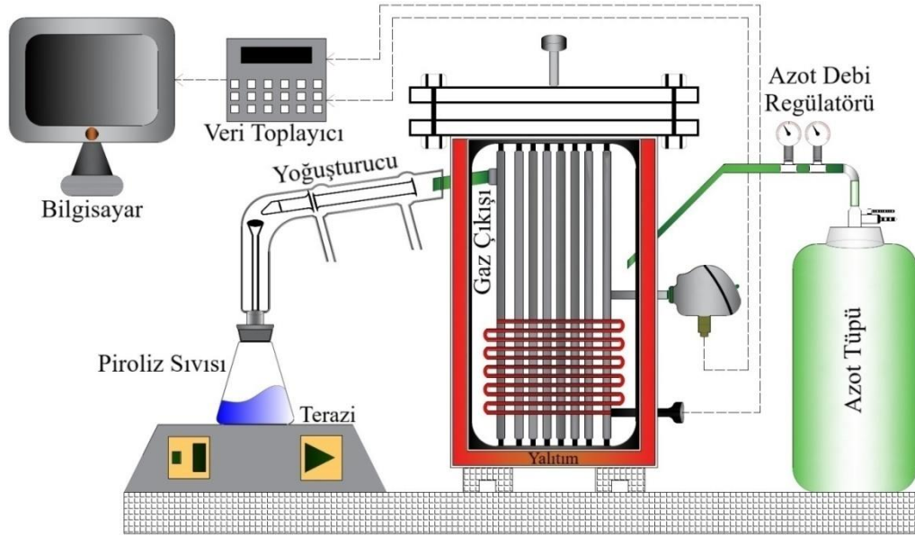
Şekil 7.2. Yakıt üretim prosesinin şematik görüntüsü
