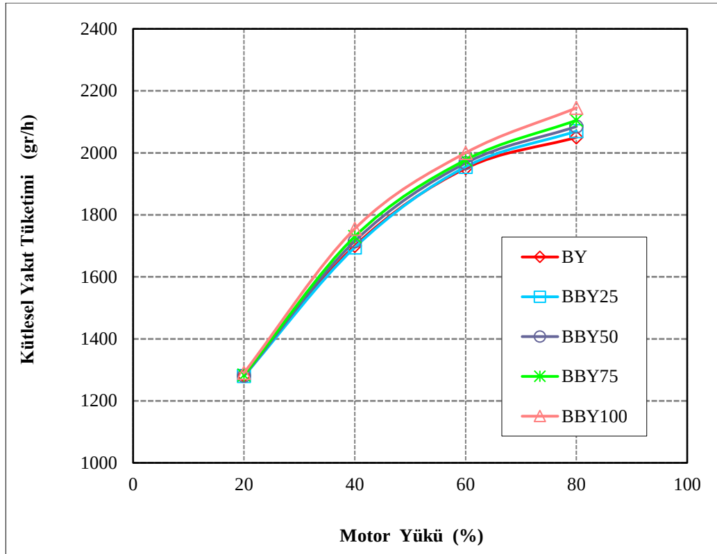
Şekil 10.1. BY, BBY ve BBY/BY karışımlarının değışken yükteki kütleşel yakıt sarfiyatı değeri
