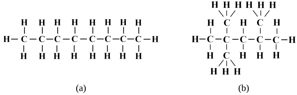
Şekil 6.3. Bağ yapıları arasındaki farklılıklar açısından oktanın gösterimi
