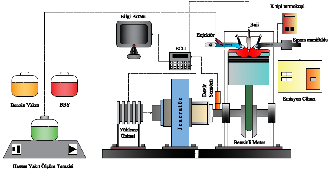
Şekil 7.5. Benzinli motor test düzeneğinin şematik diyagramı
