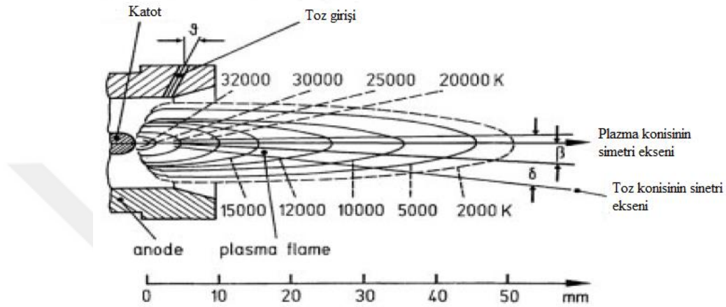
Şekil 5.4. Plazma jetinin sıcaklık dağılımı ve geometrisi [44].
