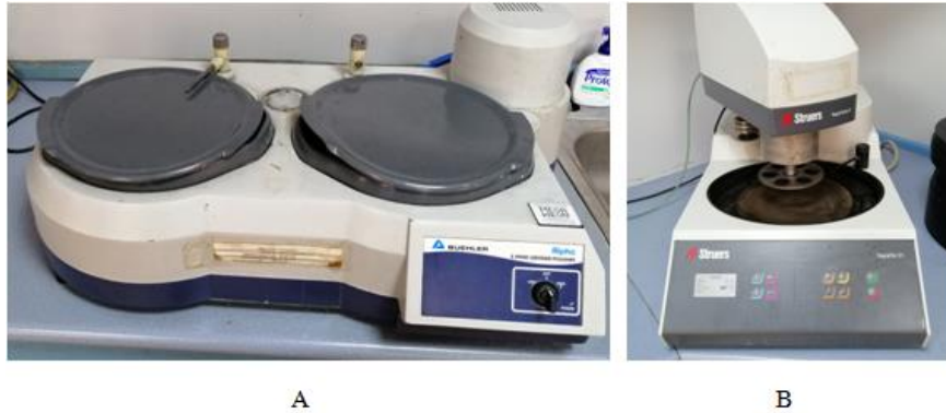
Şekil 6.13. Yarı otomatik (a) ve tam otomatik (b) zımparalama ve parlatma cihazları.
