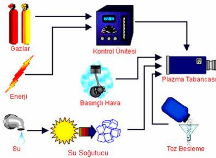
Şekil 5.6. Plazma sprej kaplama sistemi bileşenleri [19].
