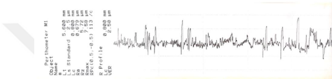
Şekil 6.5. Altlık malzemenin kumlama öncesi yüzey pürüzlülüğü.
