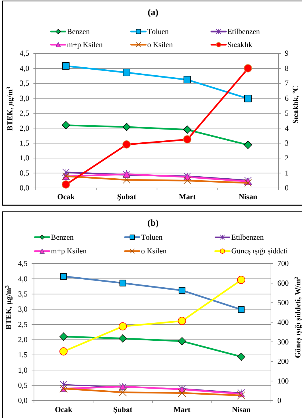
Şekil 5.33. Atmosferik BTEK derişimlerinin (a) sıcaklık ve (b) güneş ışığı şiddetine bağlı deęişimleri
