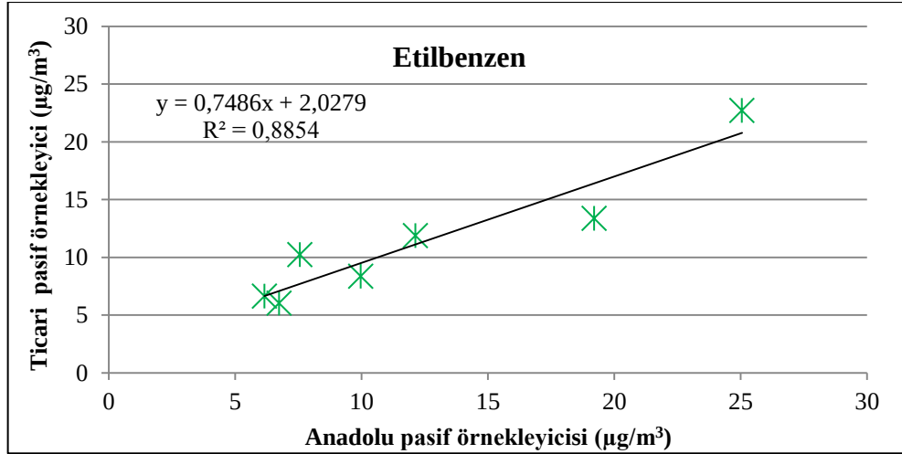
Şekil 5.27. Osmangazi Tüneli pasif örnekleme çalışmasında elde edilen Anadolu pasif örnekleycisi-ticari pasif örnekleycisi karşılaştırma sonuçları
