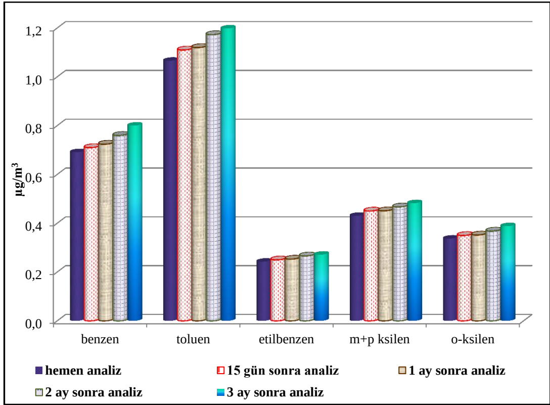
Şekil 5.8. BTEK'ler için örnekleme öncesi saklama süresinin belirlenmesi (Anadolu pasif örnekleycisi)
