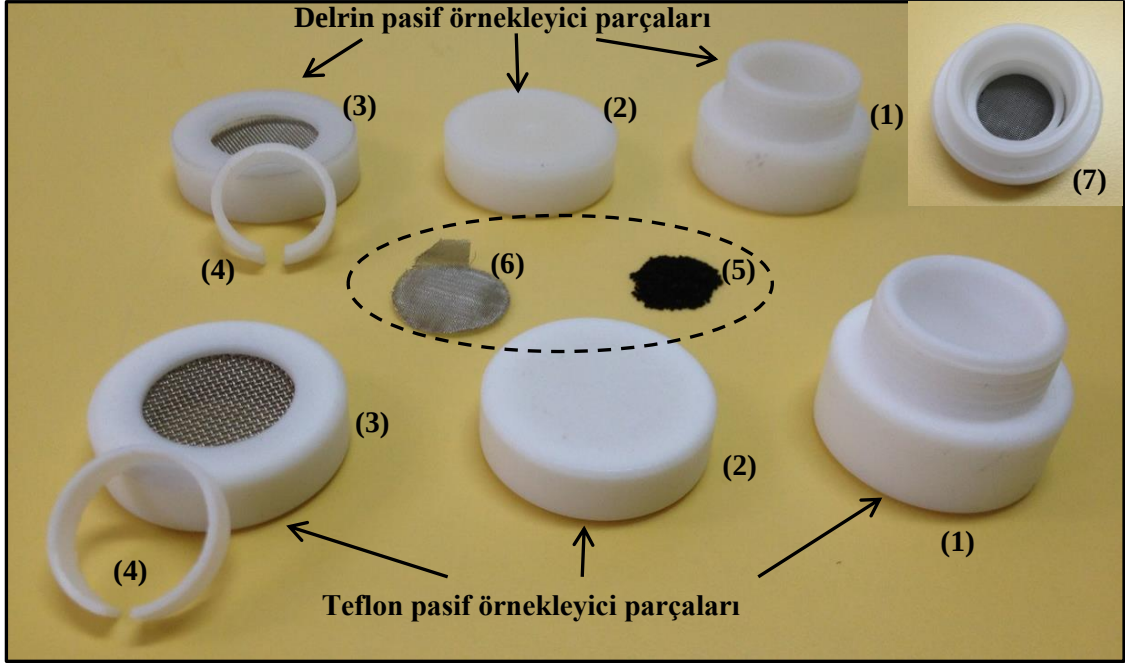
Şekil 4.5. “Granül aktif karbon+tel kafes+sabitleyici yüzük” kombinasyonları ile birlikte kullanılan teflon ve delrin malzemeye sahip pasif örnekleyiciler
