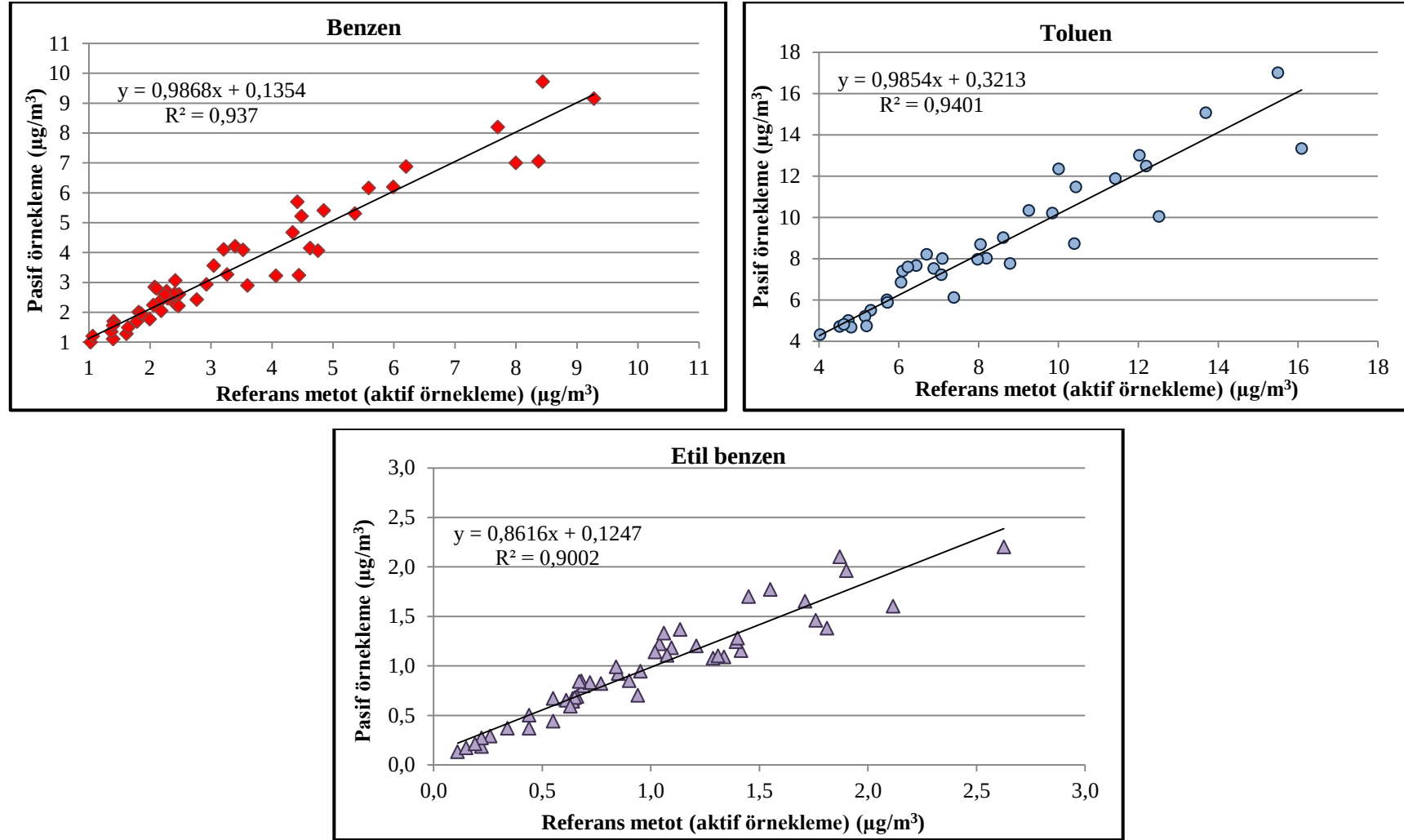
Şekil 5.5. BTEK'ler için pasif ve aktif örnekleme sonuçları arasındaki korelasyon (Anadolu pasif örnekleme)
