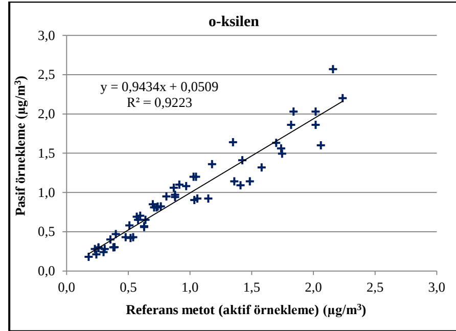
Şekil 5.5. (Devam) BTEK'ler için pasif ve aktif örnekleme sonuçları arasındaki korelasyon (Anadolu pasif örnekleycisi)
