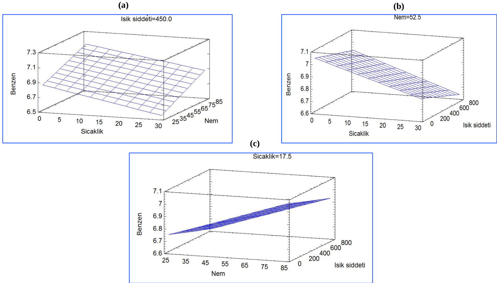
Şekil 5.18. Benzen için (a) örnekleme hızı-sıcaklık ve nem, (b) örnekleme hızı-sıcaklık ve güneş ışığı şiddeti, (c) örnekleme hızı-nem ve güneş ışığı şiddeti cevap yüzey eğrileri
