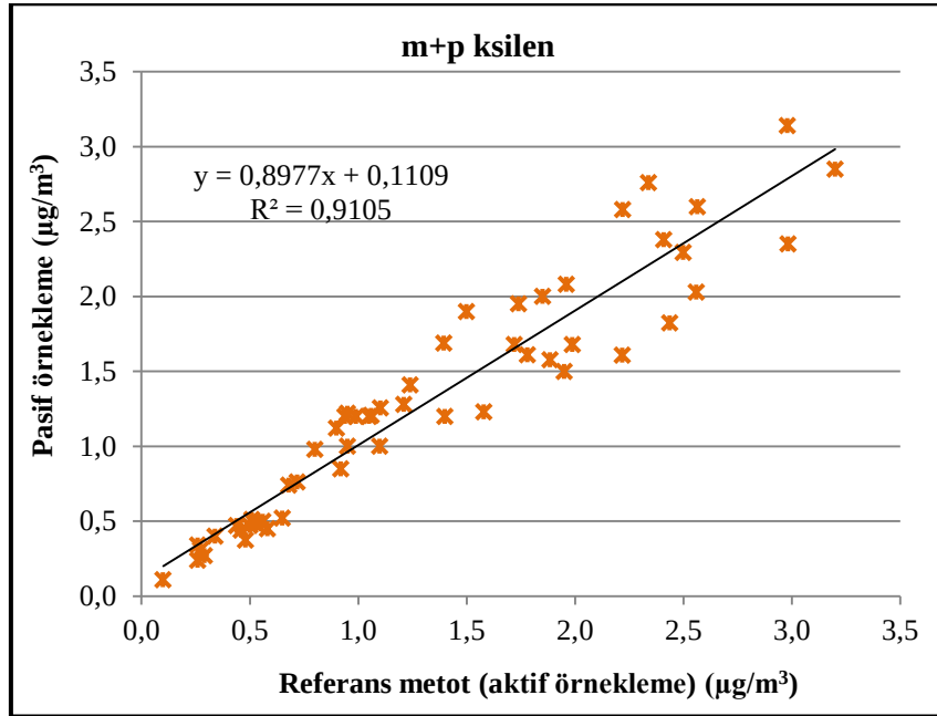
Şekil 5.5. (Devam) BTEK'ler için pasif ve aktif örnekleme sonuçları arasındaki korelasyon (Anadolu pasif örnekleycisi)
