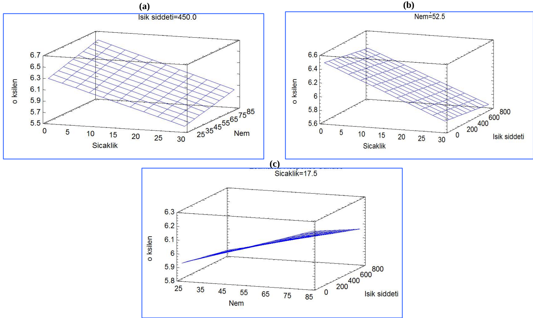
Şekil 5.26. o-ksilen için (a) örnekleme hızı-sıcaklık ve nem, (b) örnekleme hızı-sıcaklık ve güneş ışığı şiddeti, (c) örnekleme hızı-nem ve güneş ışığı şiddeti cevap yüzey eğrileri
