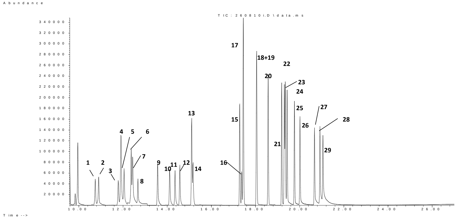
Şekil 4.23. Ozon öncül UOB kalibrasyon standardına ait kromatogram örneği
