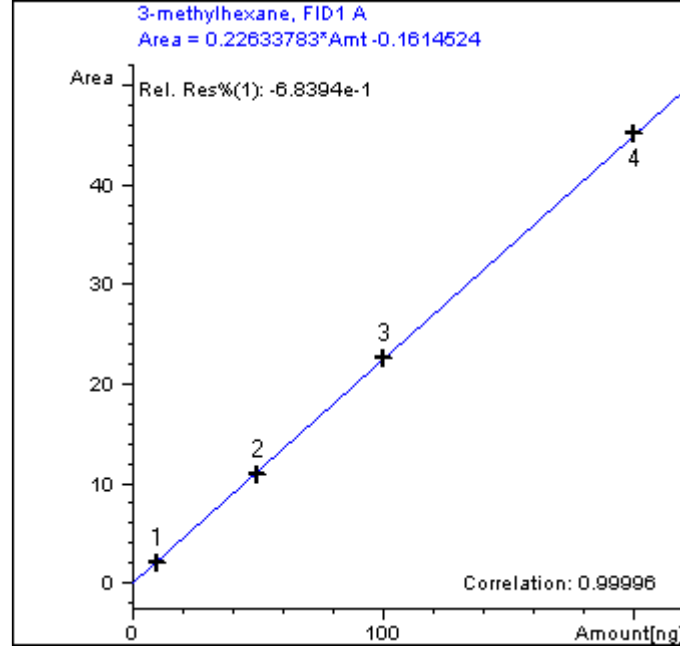
Şekil 4.25. GC-TD-FID sisteminde elde edilen kalibrasyon eğrisi örneği
