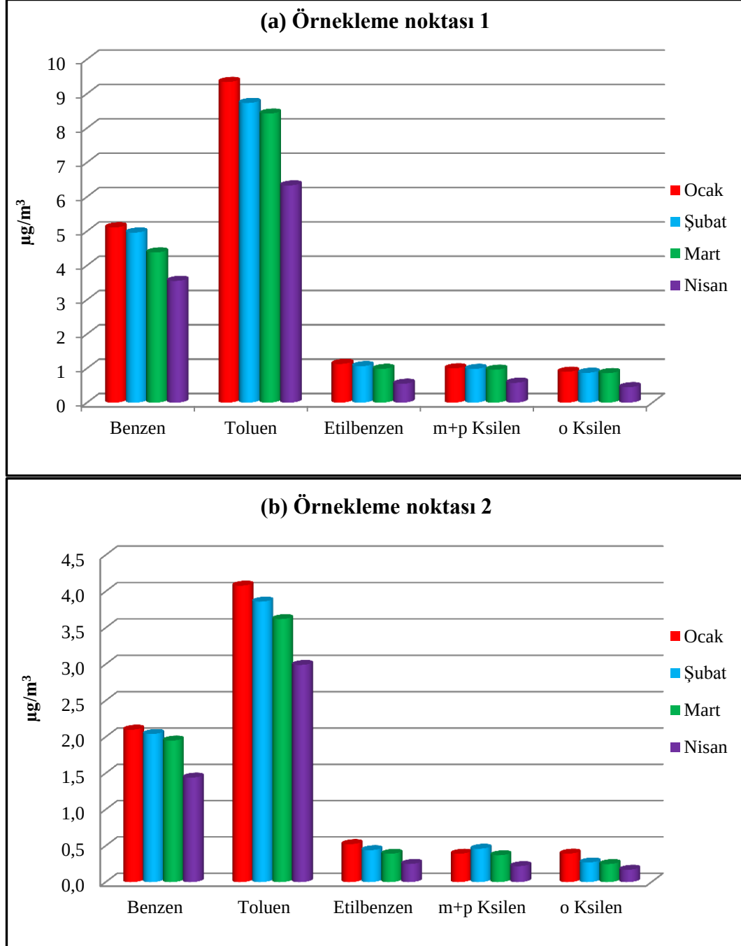
Şekil 5.32. (a) Örnekleme noktası 1 ve (b) Örnekleme noktası 2’den elde edilen aylık ortalama UOB derişim değeri
