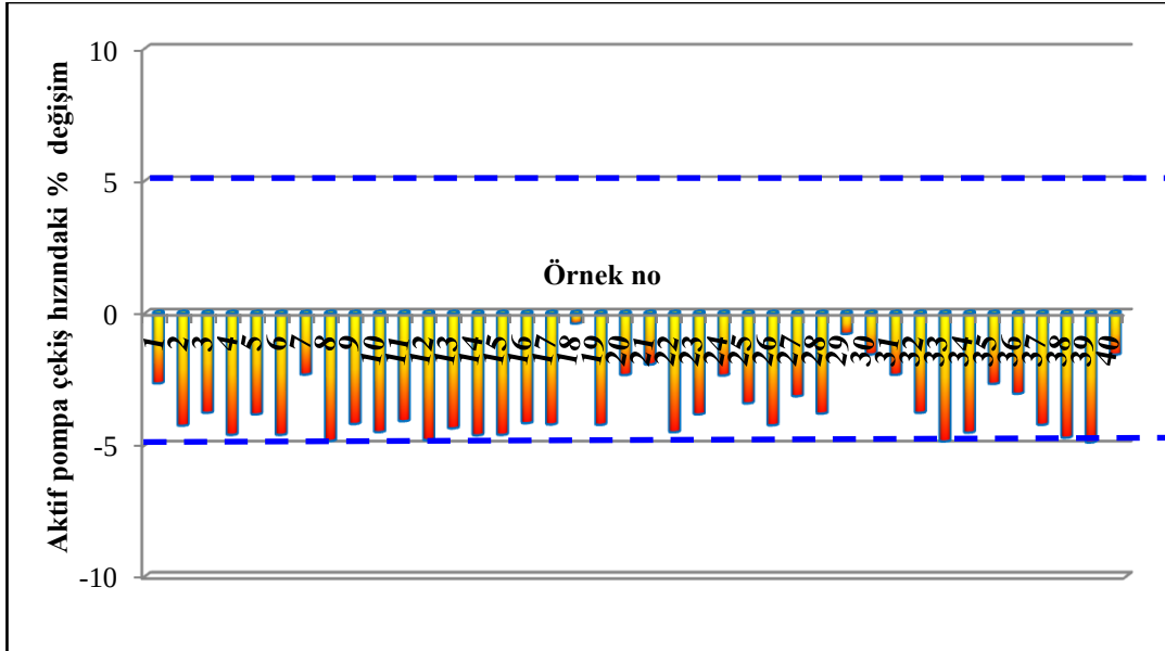
Şekil 4.18. Aktif örnekleme pompası çekiş hızı değişim yüzdesi
