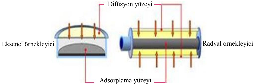
Şekil 2.5. Eksenel ve radyal pasif örnekleyci diyagramları (http-8)
