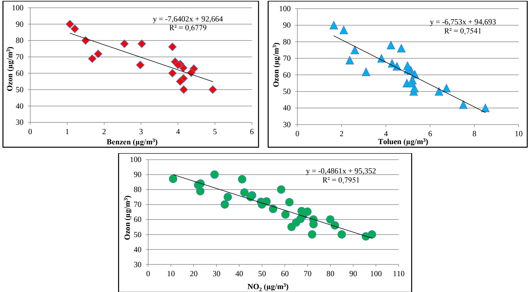
Şekil 5.34. Benzen, toluen ve NO 2 ile ozon arasındaki korelasyon grafikleri
