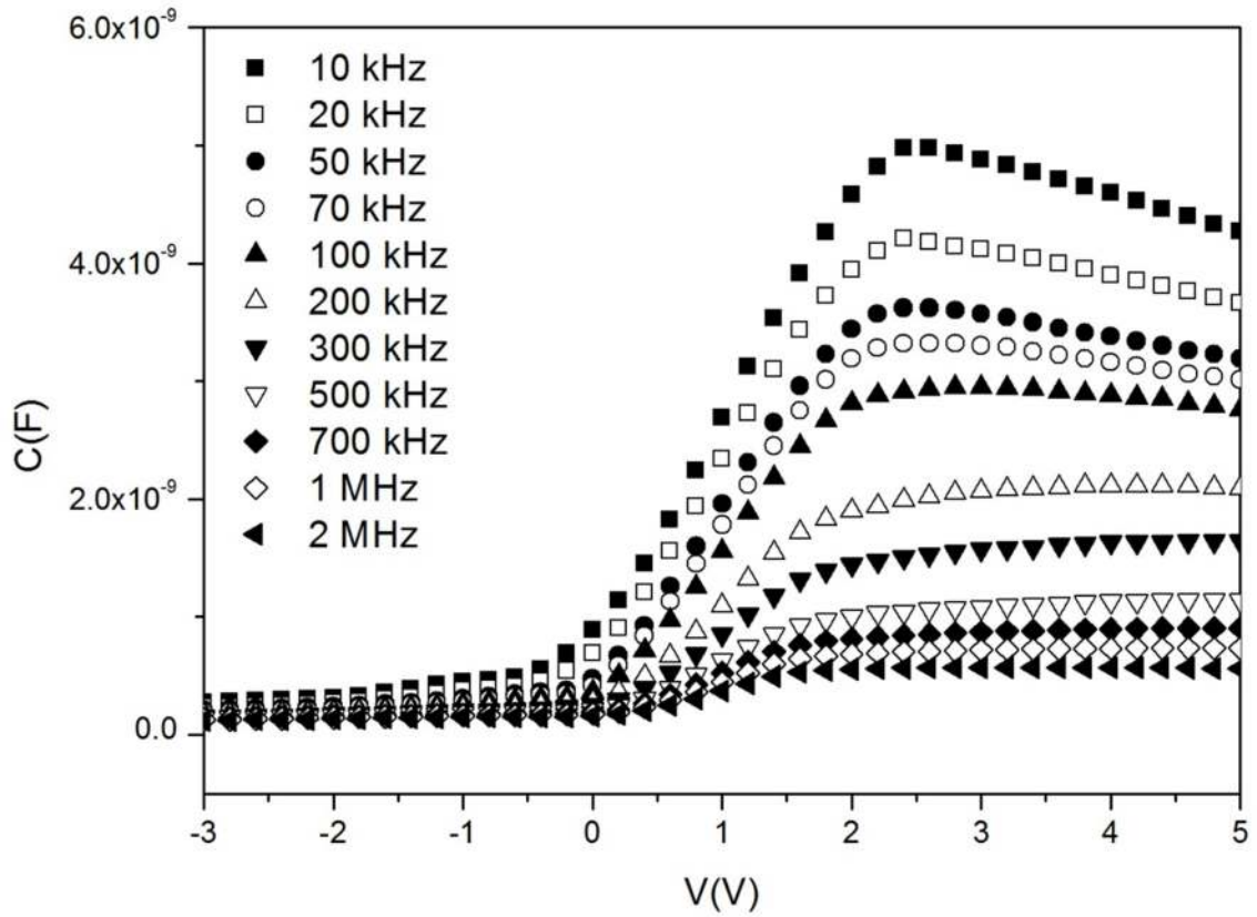
Şekil 4.1. 4:1 P3HT:PCBM katkı oranına sahip SBD'nin C - V karakteristiği.
