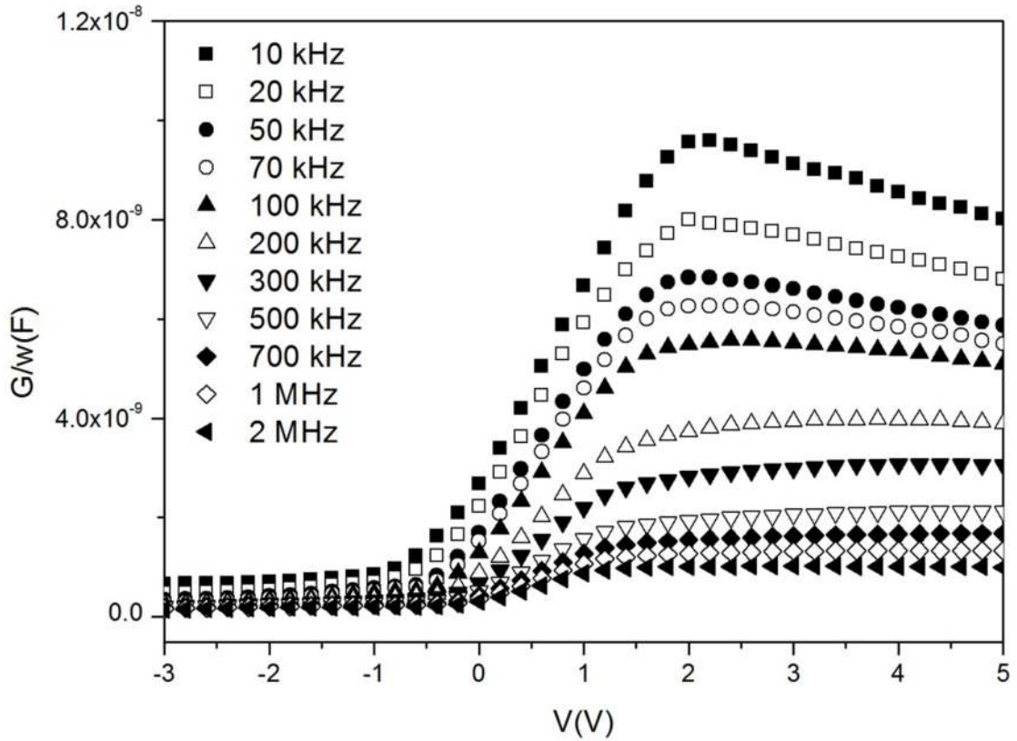
Şekil 4.2. 4:1 P3HT:PCBM katkı oranına sahip SBD'nin G/w - V karakteristiği.
