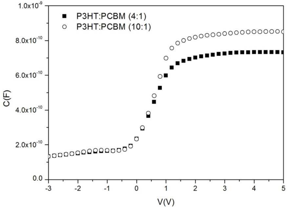
Şekil 4.5. 4:1 ve 10:1 P3HT:PCBM katkı oranları kullanılarak üretilen Au/P3HT:PCBM/n-Si MPY SBD'lerin 1 MHz frekans değerindeki kapasitans-voltaj ( C-V ) karakteristikleri.
