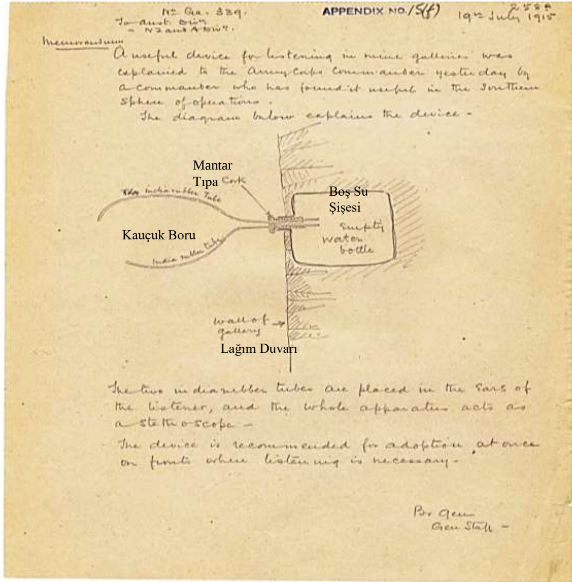
Şekil 15: Karşı Lağımları Dinlemeye Yarayan Tertibat
