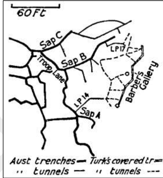
Şekil 23: ANZAK Bölgesinde Bazı Lağımları Gösterir Kroki
