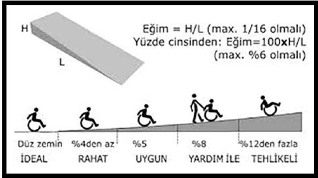
Şekil 2.5: Rampalarda güvenli eğim aralıkları
