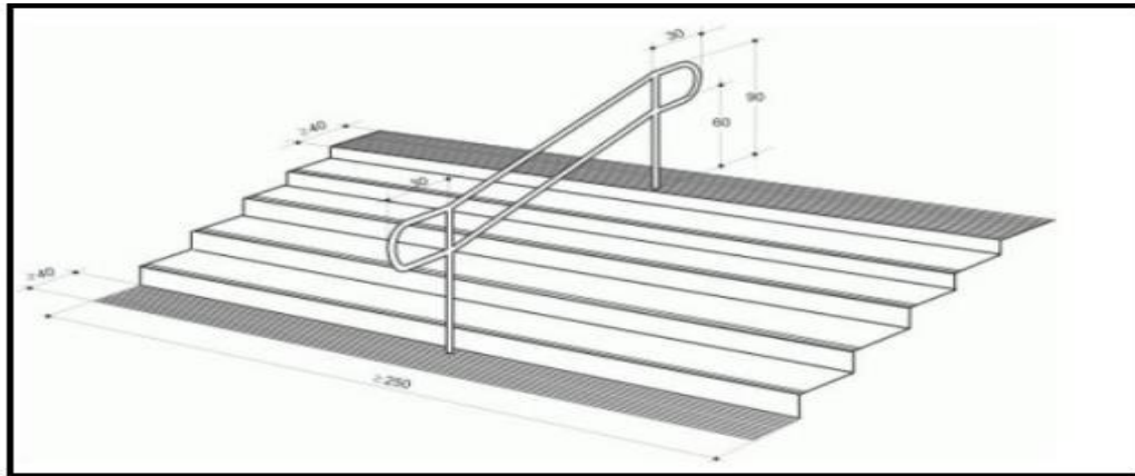
Şekil 2.8: Merdivenlerde hissedilebilir yüzeyler
