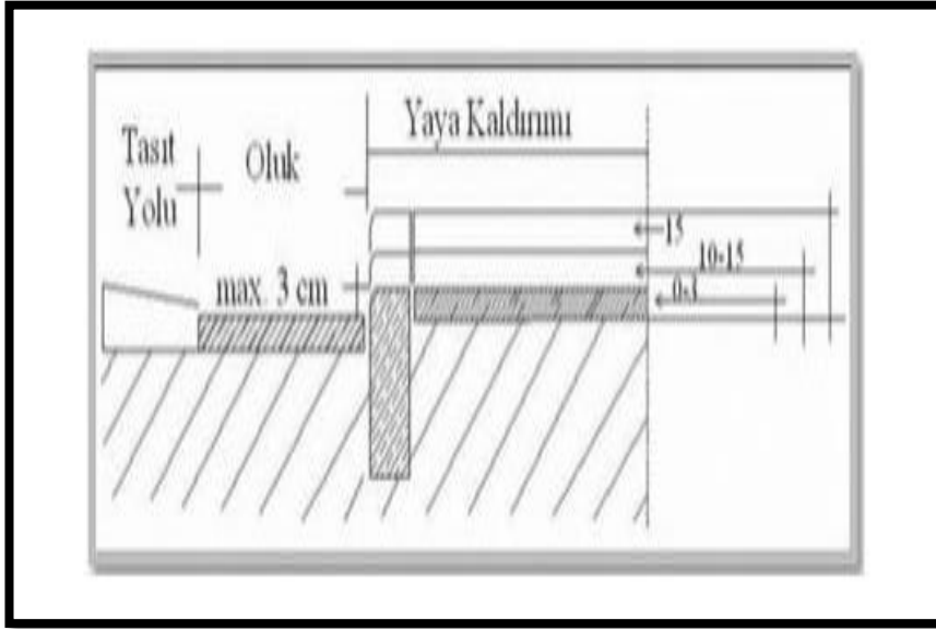
Şekil 2.4: Bordür taşının otoyola olan yükseltisi
