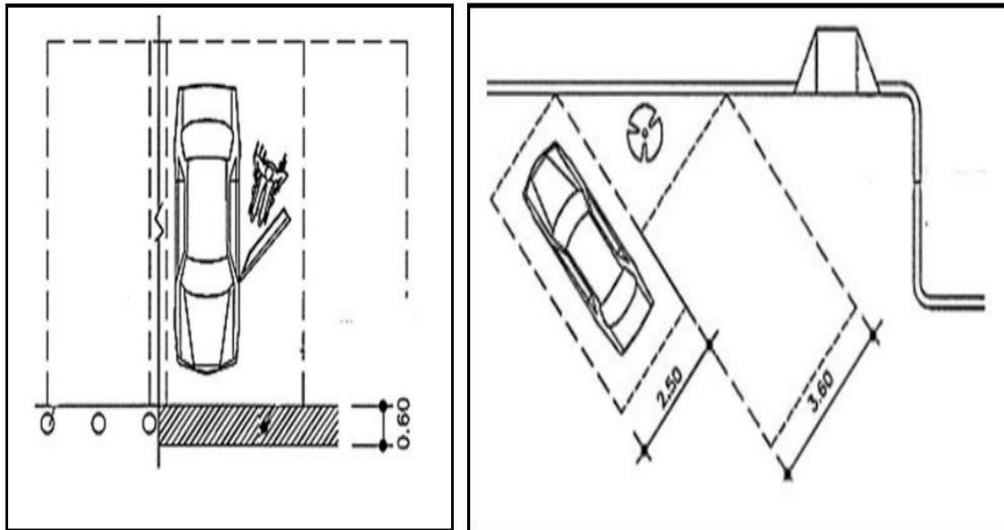
Şekil 2.9: Engelli otoparkı düzeni
