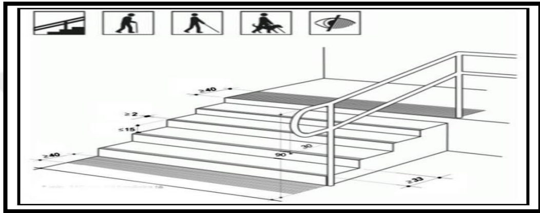
Şekil 2.7: Uyarıcı hissedilebilir yüzey
