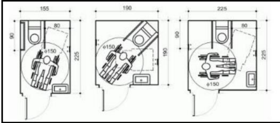
Şekil 2.12: Engelli bireyler için tuvalet boyutları
