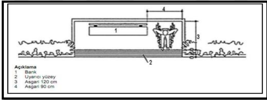
Şekil 2.14: Oturma banklarına tekerlekli sandalyenin yanaşması
