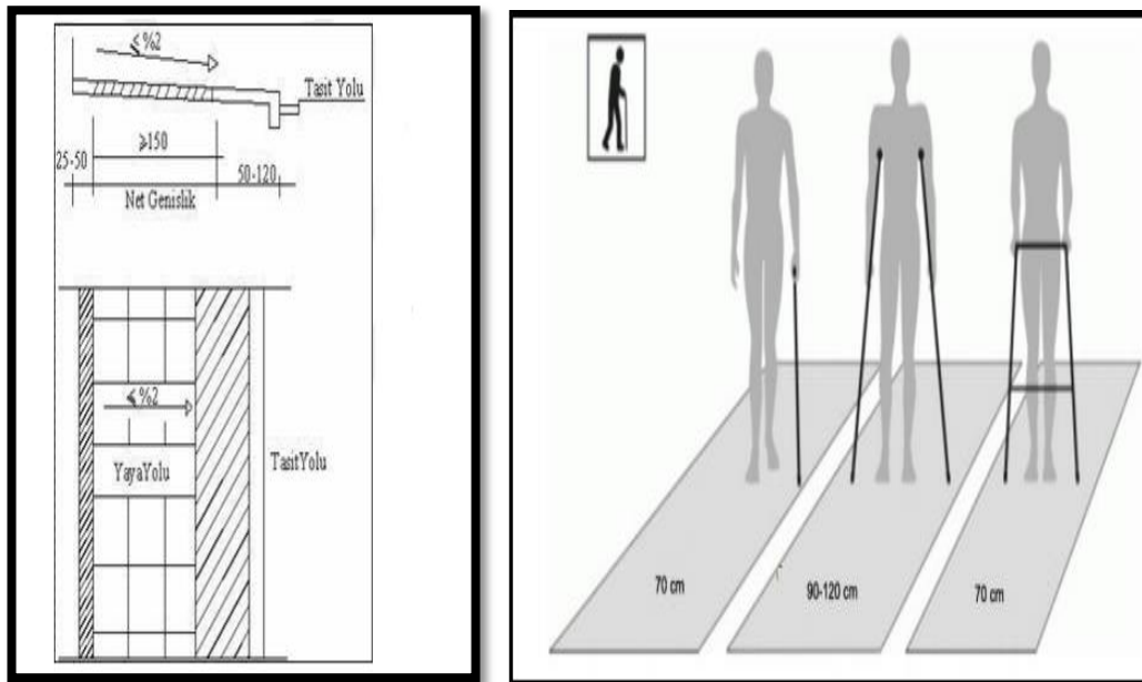
Şekil 2.1: Engelli bireyler için yaya kaldırım genişliği
