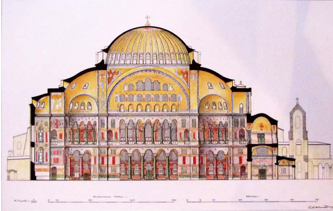
Şekil 2.5. Ayasofya Katedrali Doğu-Batı Yönlü Kesiti 14. Yüzyıl
