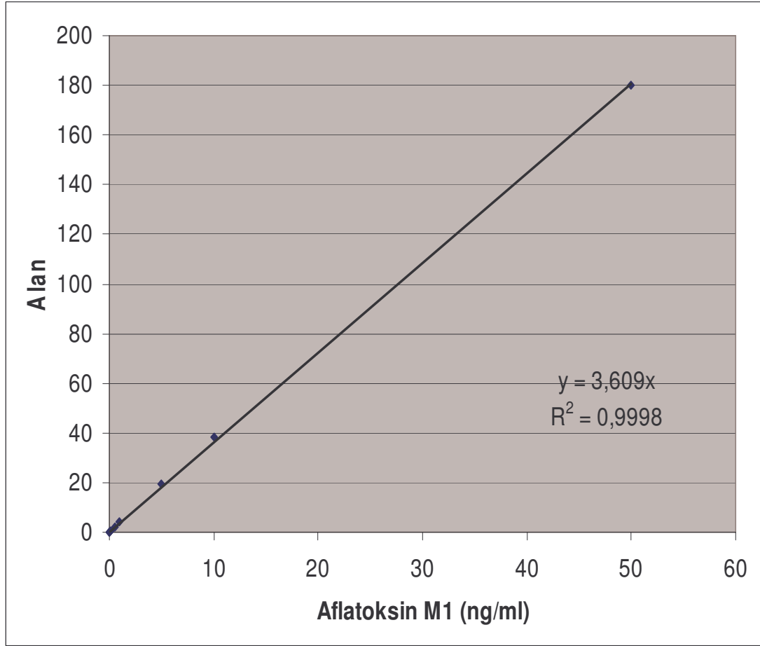
Şekil 10. Aflatoksin M 1 standardı kalibrasyon eğrisi.
