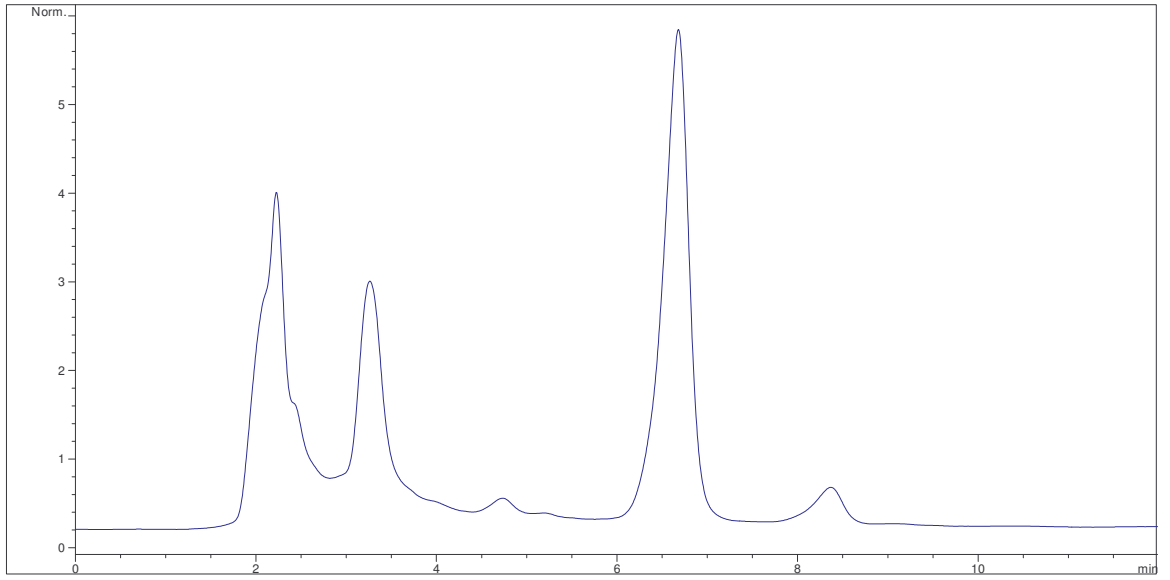
Şekil 7: Aflatoksin M 1 ilave edilen (10 ppb) yoğurt kromatogramı örneği.
