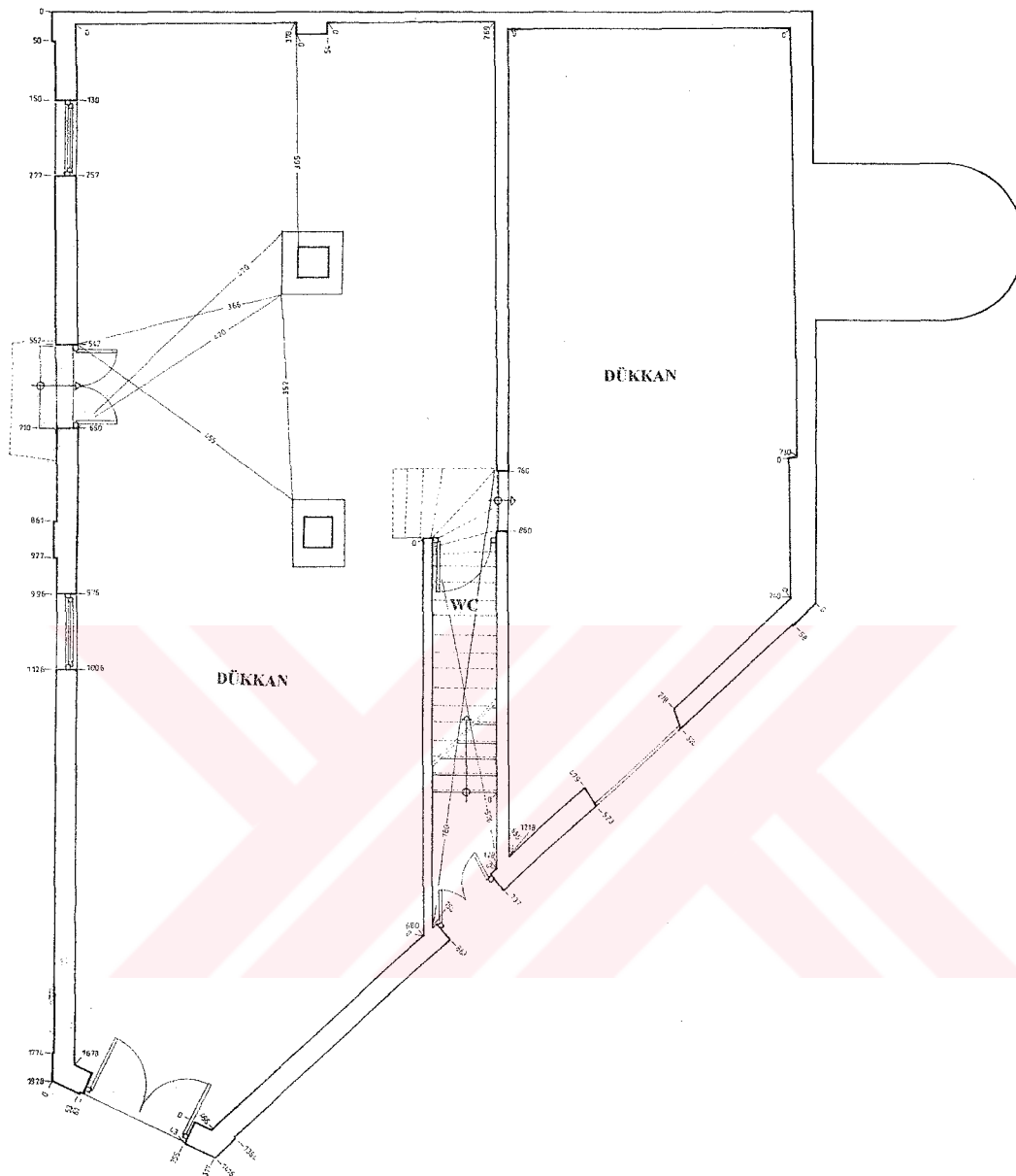
Çizim 4.14. Şehir Klübü Binası Zemin Kat Rölöve Planı Ö:1/100
