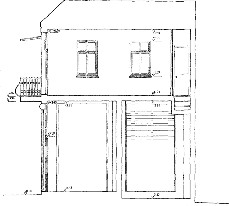
Kesit 1/100
