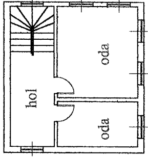
1. KAT PLANI
