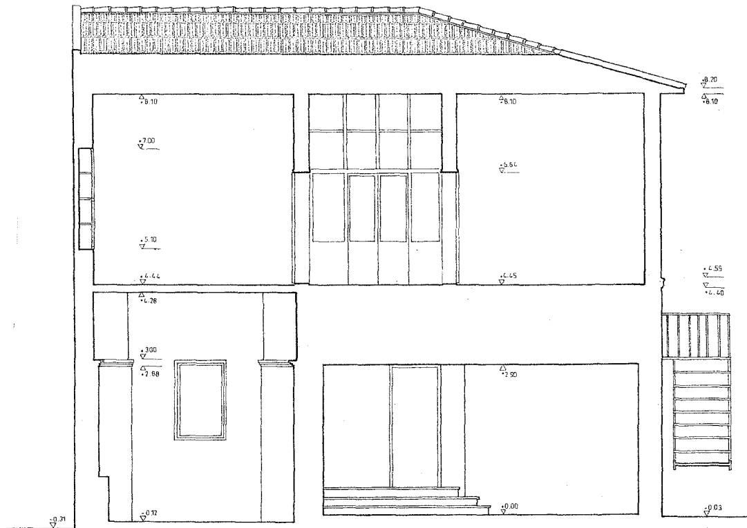
Kesit Ö:1/100
