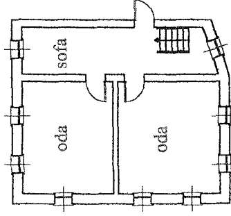
1. KAT PLANI
