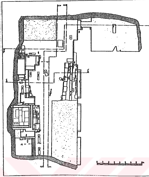
Çizim 4.1. Tralleis-Büyük Hamam Salon Taban Planı
