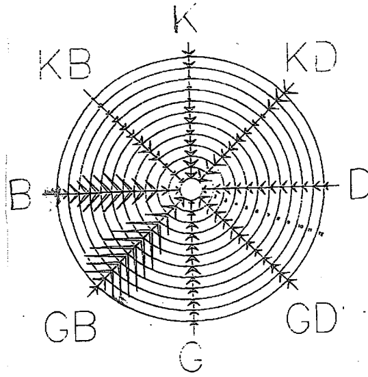
Şekil 2.2 Aydın İli Rüzgar Gücü
