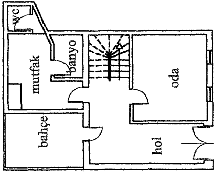
ZEMİN KAT PLANI
