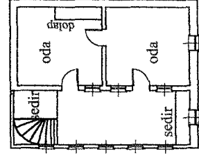
1. KAT PLANI
