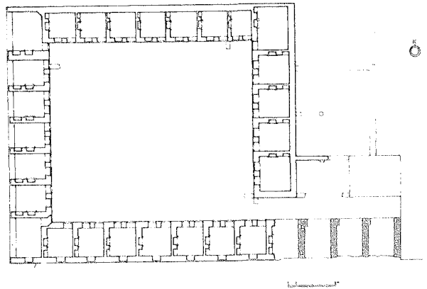
Çizim 5.10. Zincirli Han Birinci Kat Planı
