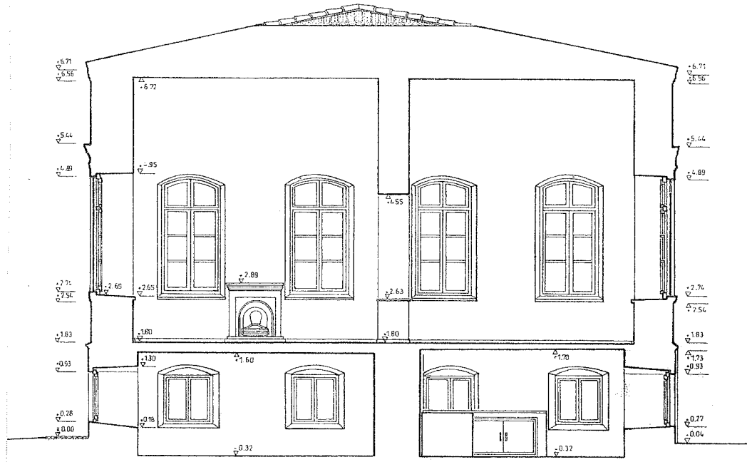
Orhan Çiftçi Evi Kesiti 1/100
