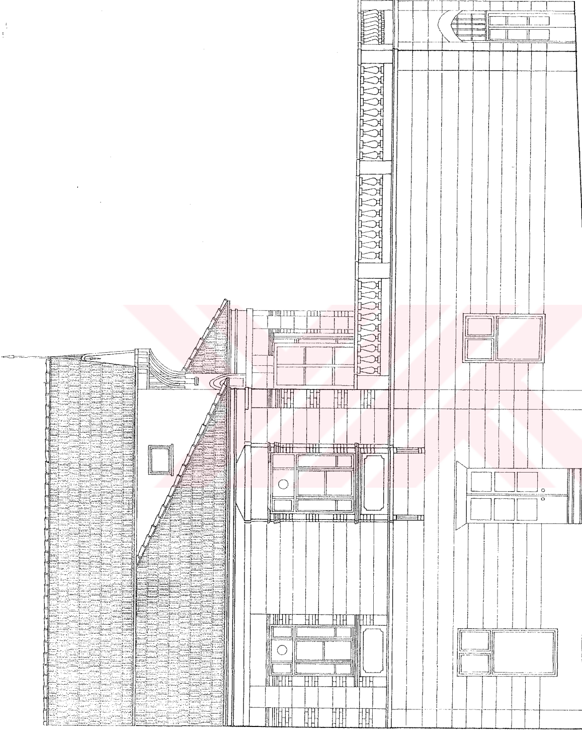
Çizim 4.19. Şehir Klübü Binası Rölöve Giriş Cephesi Ö: 1/100
