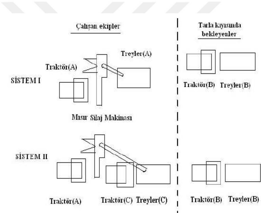
Şekil 9. Mısır silajı yapımında uygulanan mekanizasyon sistemleri ve akış şeması. (Topuz, 2005)
