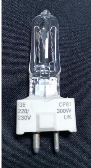
Resim 4.2. GE marka 300 W tungsten halojen lamba.
