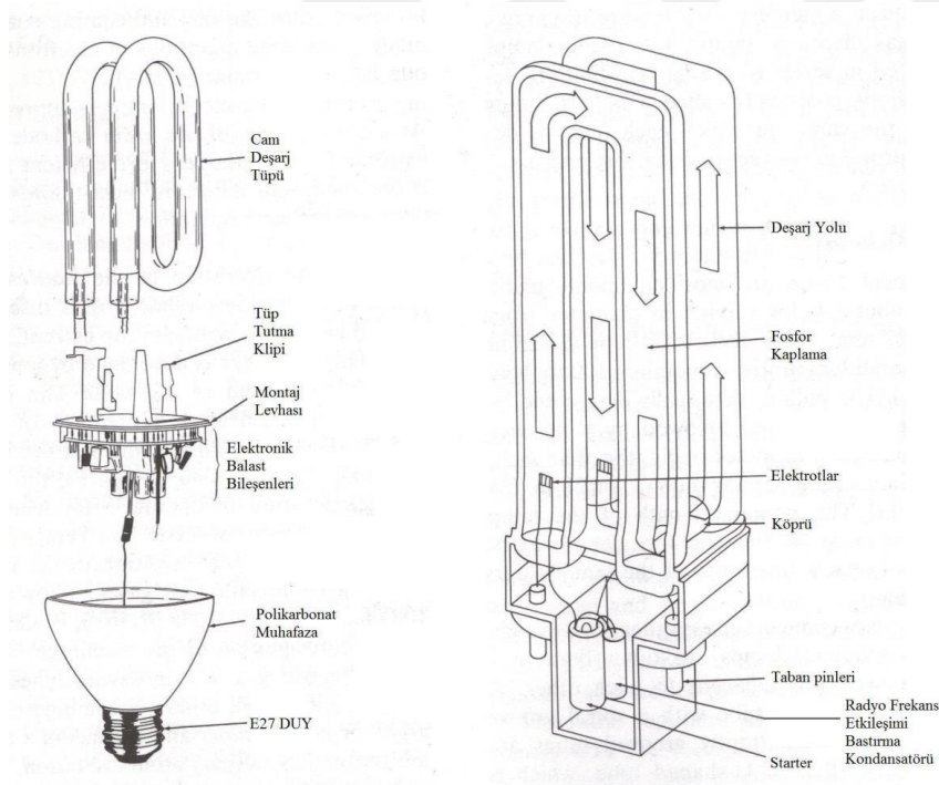
Şekil 2.38. Kendinden balastlı ve starterli kompakt flüoresan bölümleri [85].
