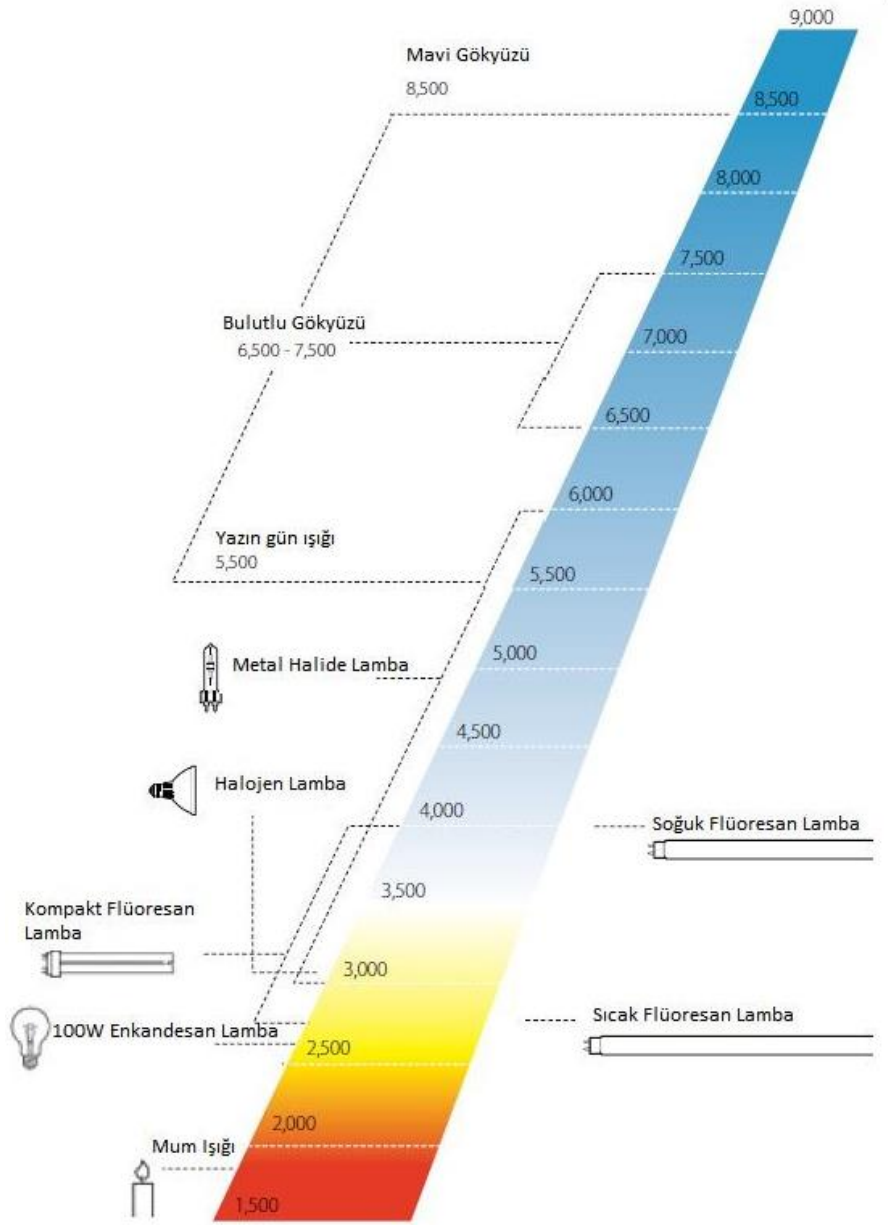
Şekil 2.18. Çeşitli ışık kaynaklarının renk sıcaklığı değerleri [28].
