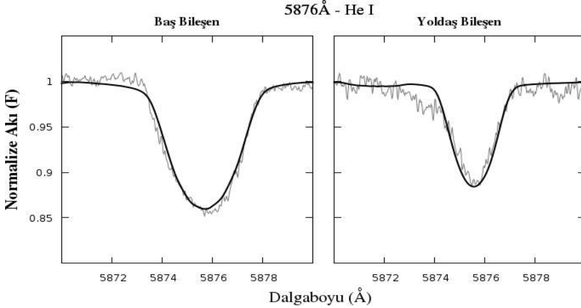
Şekil 3.11. MQ Cen sisteminin ayıklanmış Helyum (5876Å) çizgileri (gri) ve bu çizgiler ile en iyi uyum içerisinde olan model atmosfer uygulaması ile elde edilmiş sentetik tayflar (siyah)
