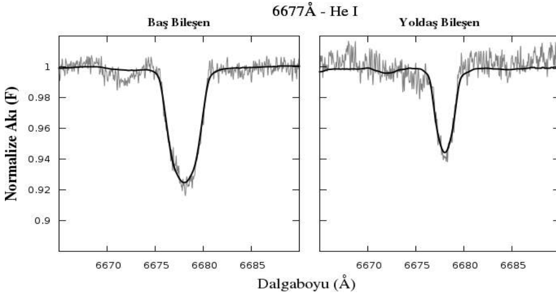
Şekil 3.12. MQ Cen sisteminin ayıklanmış Helyum (6677Å) çizgileri (gri) ve bu çizgiler ile en iyi uyum içerisinde olan model atmosfer uygulaması ile elde edilmiş sentetik tayflar (siyah)
