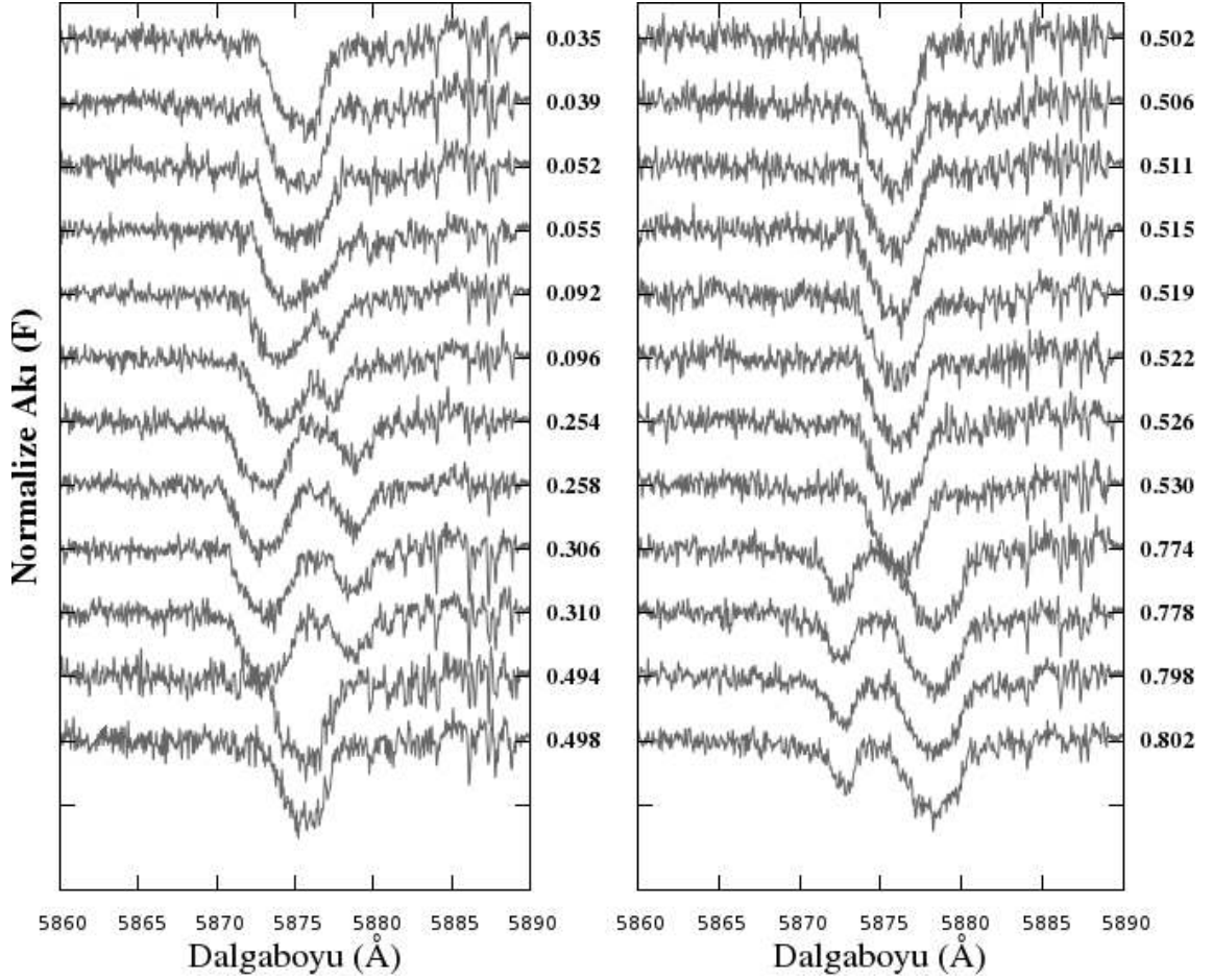
Şekil 3.4. MQ Cen sisteminin 5876Å (He I) çizgisine ait 0 ile 0.5 arasında evreye göre sıralı tayfları (solda), 0.5 ile 1.0 arasında evreye göre sıralı tayfları (sağda), tayfların gözlendiği evreler panellerin sağ kenarlarına yerleştirilmiştir
