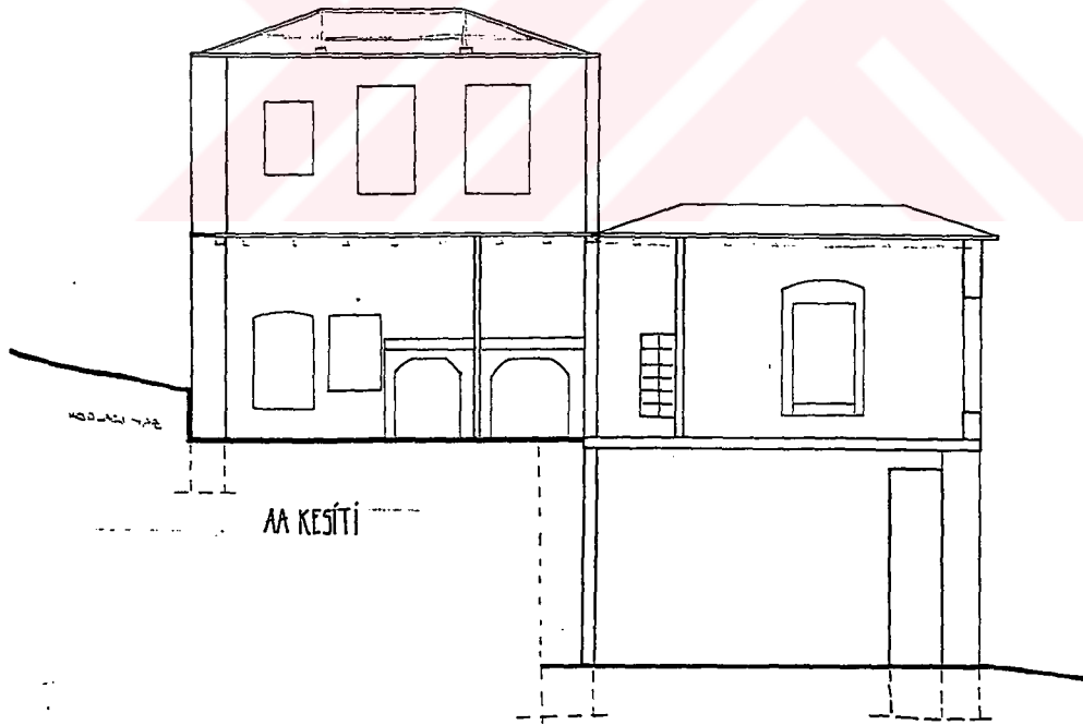
ŞEKİL 4.45 Girişin hemen solundaki ve onun önündeki yapının kesiti
