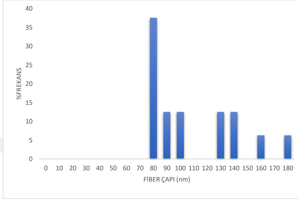
Şekil 4.6. PCL-Gel nanolişinin lif çapı grafiği
