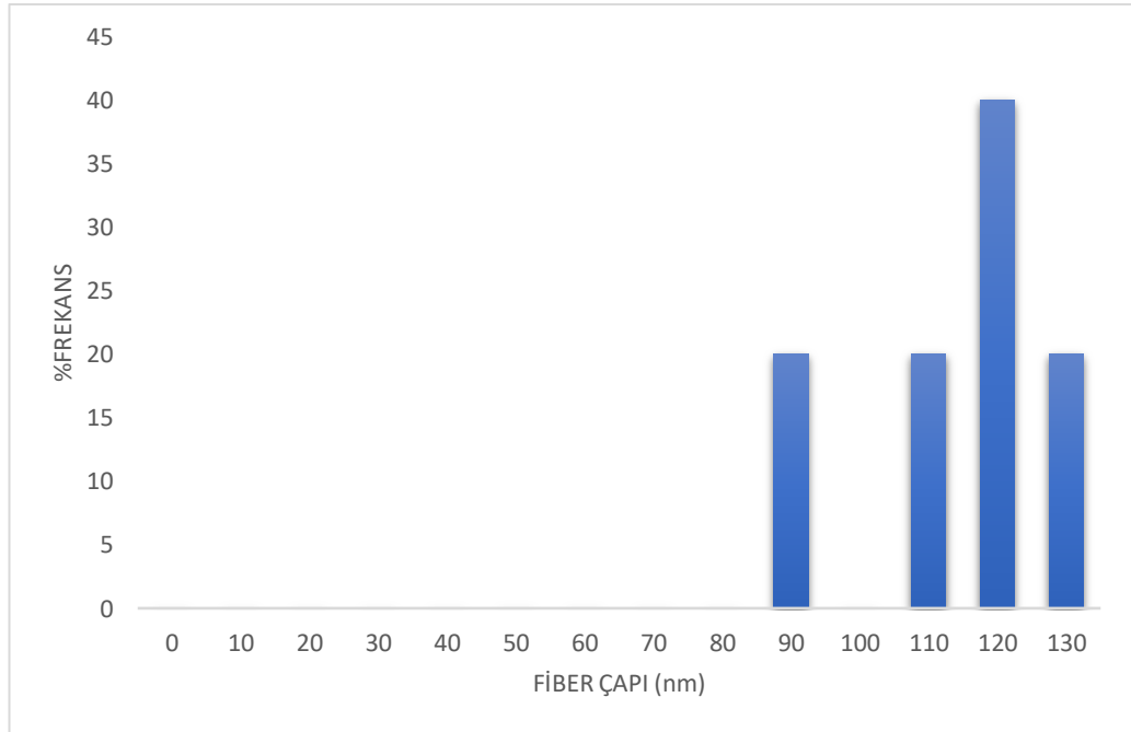
Şekil 4.7. PCL-Gel-B12 nanolişinin lif çapı grafiği
