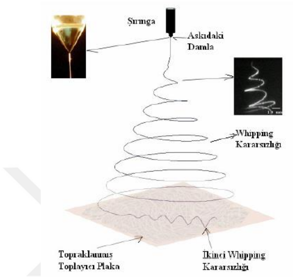
Şekil 2.7. Elektroçekim yönteminde Whipping kararsızlığı
