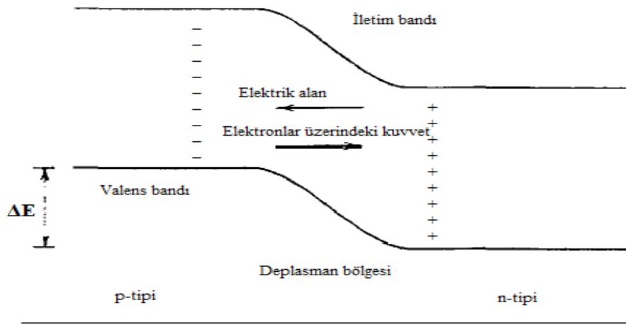
Şekil 4.5 : p-n eklemine ait şematik görünümü (Krane, 1988).
