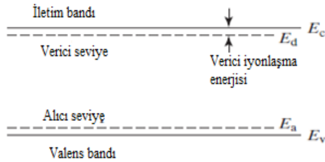
Şekil 4.4 : Yarı iletkenlerde verici ve alıcı seviyeler (Url-5).
