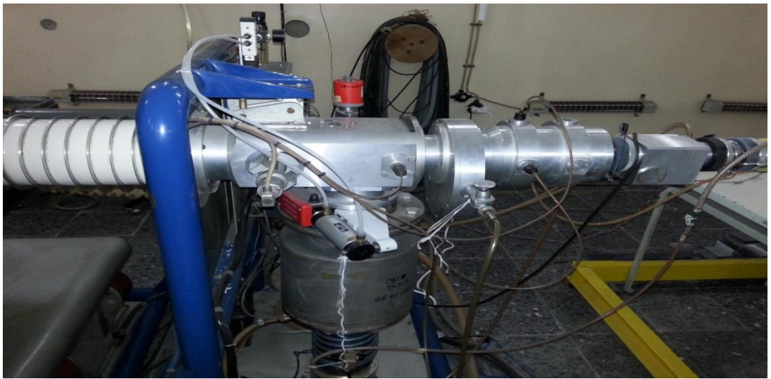
Şekil 5.1 : Sames J-15 hızlandırıcısının ana hızlandırma ünitesi.
