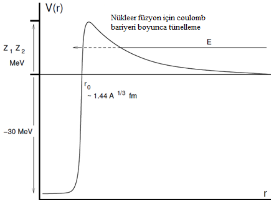
řekil 3.7 : Birbirlerine yaklařmakta olan iki \u00e7ekirdek arasındaki potansiyel enerji eđrisinin \u00e7ekirdekler arasındaki uzaklıđa bađlı olarak deđiřimi (Url-4).
