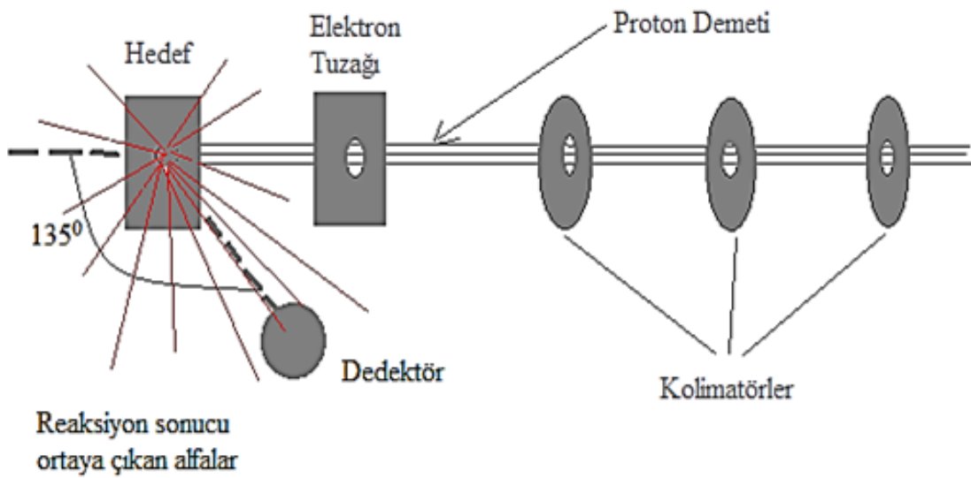
Şekil 5.4 : Dedektör geometrisi.
