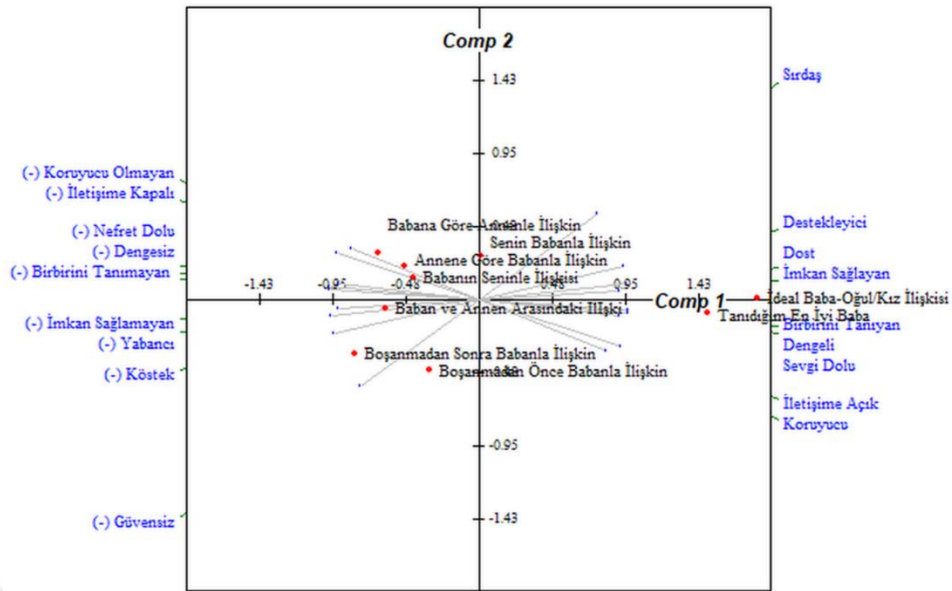
Şekil 3 Temel bileşenler analizi grafiksel gösterimi (Olgu 2)
