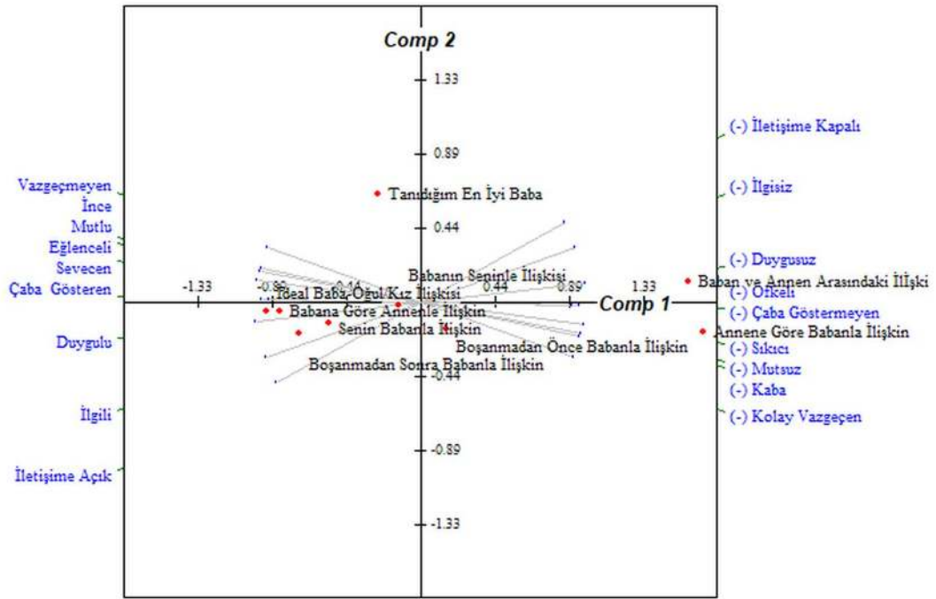
Şekil 17: Temel bileşenler analizi grafiksel gösterimi (Olgu 9)
