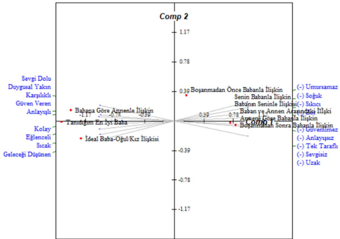
Şekil 1: Temel bileşenler analizi grafiksel gösterimi (Olgu 1)
