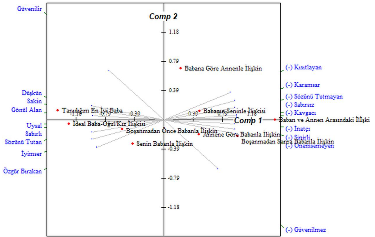
Şekil 9: Temel bileşenler analizi grafiksel gösterimi (Olgu 5)
