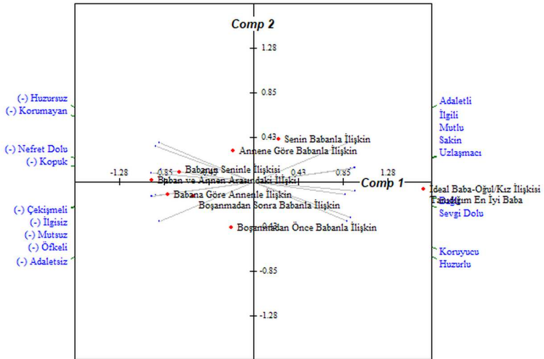
Şekil 5. Temel bileşenler analizi grafiksel gösterimi (Olgu 3)
