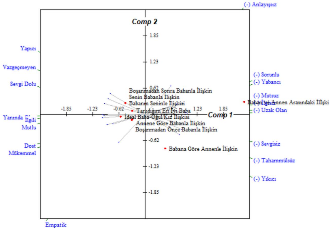
Şekil 11: Temel bileşenler analizi grafiksel gösterimi (Olgu 6)
