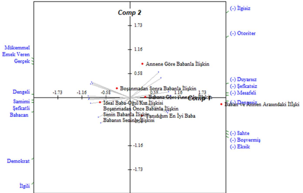
Şekil 15: Temel bileşenler analizi grafiksel gösterimi (Olgu 8)
