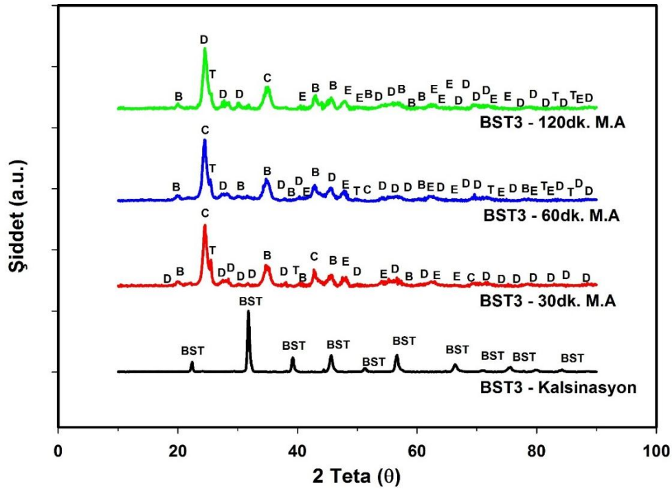
Şekil 5.2. BST3 tozlarının XRD analizi (BST: Baryum stronsiyum titanat, B: \text{BaCO}_3 , C: Baryum stronsiyum karbonat, D: \text{BaTi}_4\text{O}_9 -Baryum tetra titanat, E: Baryum titanyum oksit, T: \text{TiO}_2 ).
