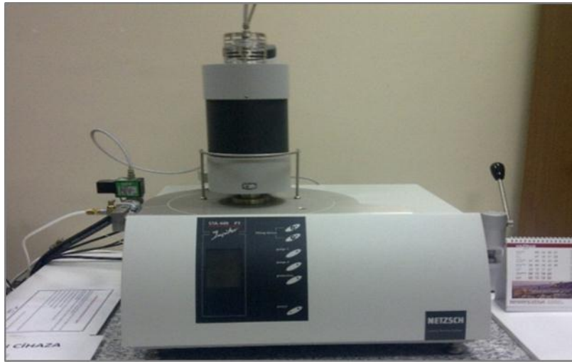
Şekil 4.11. Deneysel çalışmalarda kullanılan Netzsch marka DTA/TG analiz cihazı
