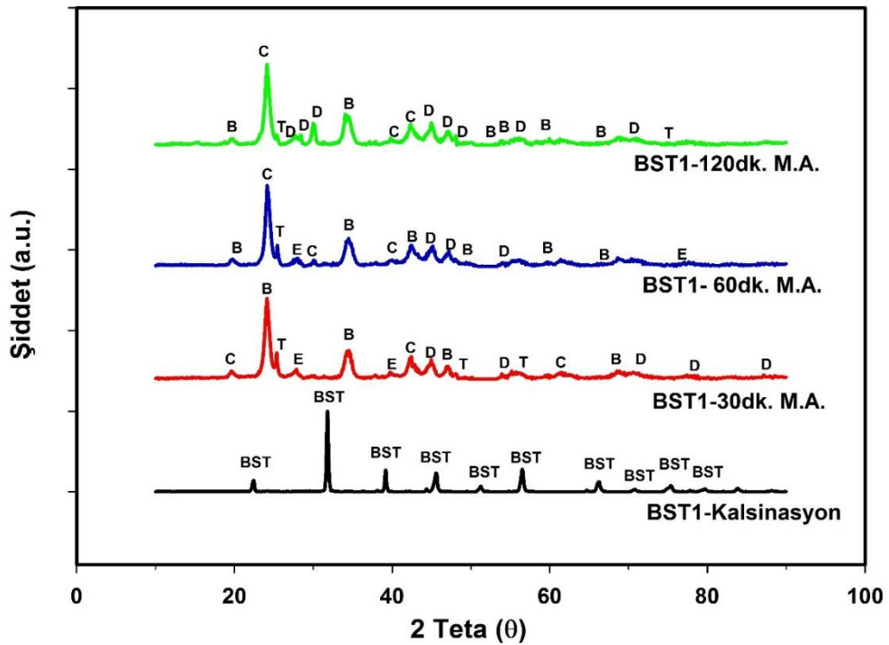
Şekil 5.1. BST1 tozlarının XRD analizi (BST: Baryum stronsiyum titanat, B: BaCO_3 , C: Baryum stronsiyum karbonat, D: BaTi_4O_9 -Baryum tetra titanat, E: Baryum titanyum oksit, T: TiO_2 ).
