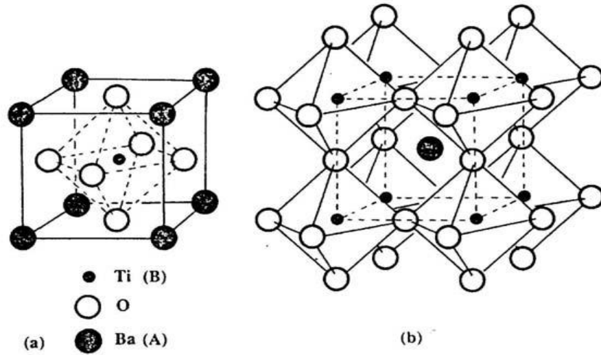
Şekil 2.4. (a) \text{ABO}_3 tipi perovskit kübik birim hücresi ve (b) \text{BO}_6 oktahedra'nın üç boyutlu ağ örgüsü [12].
