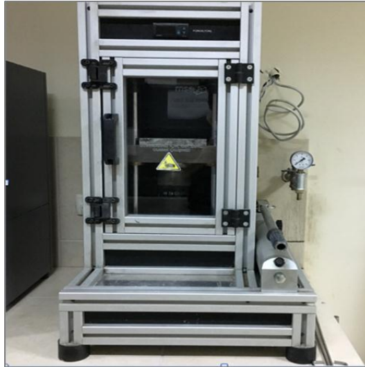
Şekil 4.7. Deneyisel çalışmalarda kullanılan MSE marka manuel pres
