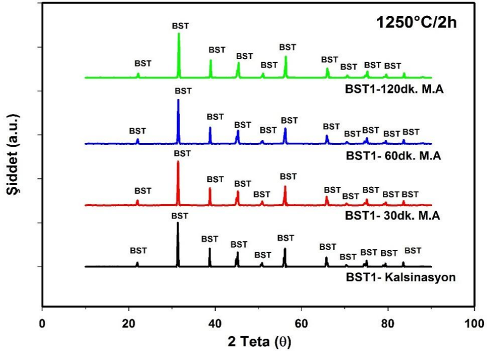
Şekil 5.12. BST1 numunelerinin 1250°C’de 2 saat sinterlenme sonrası XRD analizi (BST: Baryum stronsiyum titanat).
