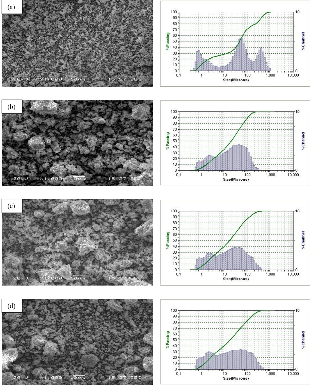
Şekil 5.6. BST5 tozlarının 1000 büyütmedeki SEM görüntüleri ve tane boyut dağılım analizi, (a) 1000°C/3saat'te kalsinasyon işlemi olmuş, (b) 30dk. mekanik aktive edilmiş, (c) 60dk. mekanik aktive edilmiş ve (d) 120dk. mekanik aktive edilmiş tozlar
