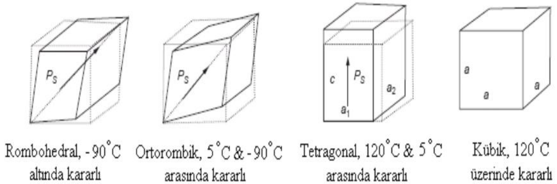
Şekil 2.14. BaTiO 3 kristalinin sıcaklığa bağlı olarak kristal yapı değişimi [15].
