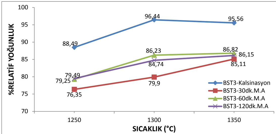
Şekil 5.10. BST3 numunelerine ait yoğunluk grafikleri
