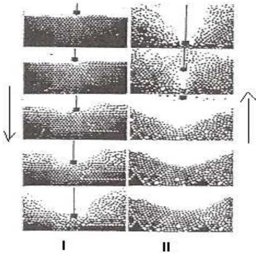
Şekil 3.2. Küresel modelle şematik olarak gerçekleştirilmiş darbe geriliminin farklı kademeleri (↓-katının latisine penetrasyon, ↑-latis distorsiyonu oluşarak fazın bozulması) [25].
