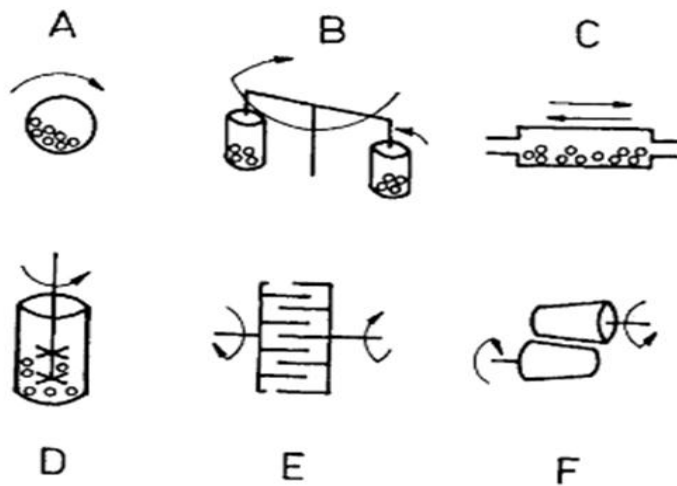
Şekil 3.5. Mekanik aktivasyon için kullanılan değirmen tipleri ve gerilim tipleri, A- Bilyalı değirmen (R1-R4), B- Gezegenel değirmen (R1-R4), C- Titreşimli değirmen (R1-R4), D- Karıştırıcı bilyalı değirmen-atritör (R1-R4), E- Mil değirmeni (R4) ve F- Haddeli Değirmen (R1-R2) [25].
