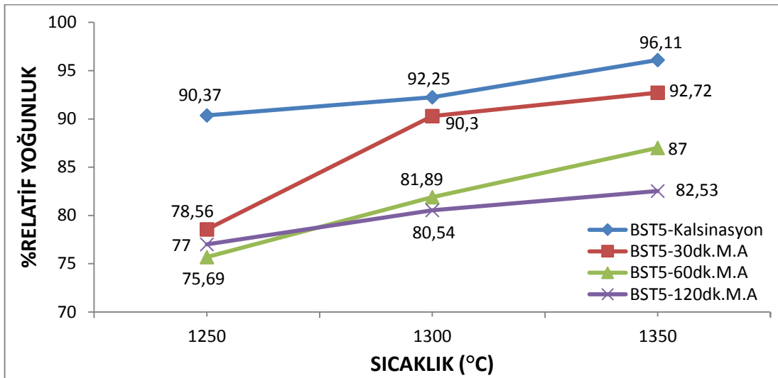
Şekil 5.11. BST5 numunelerine ait yoğunluk grafikleri
