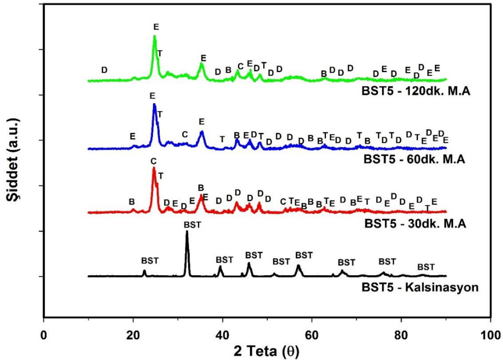
Şekil 5.3. BST5 tozlarının XRD analizi (BST: Baryum stronsiyum titanat, B: \text{BaCO}_3 , C: Baryum stronsiyum karbonat, D: \text{BaTi}_4\text{O}_9 -Baryum tetra titanat, E: Baryum titanyum oksit, T: \text{TiO}_2 ).
