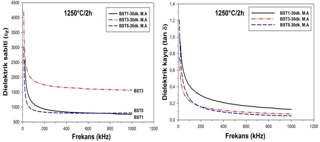
Şekil 5.30. 1250°C’de 2 saat sinterlenen 30dk. mekanik aktive edilmiş BST numunelerinin dielektrik sabiti ( \epsilon_r ) ve dielektrik kayıp ( \tan \delta ) ölçüm grafiği
