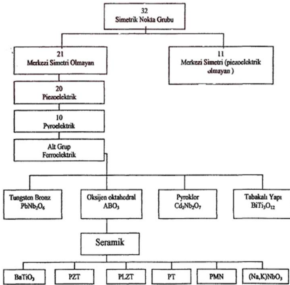
Şekil 2.15. Piezoelektrik ve alt gruplarının simetri üzerine ilişkileri [10].
