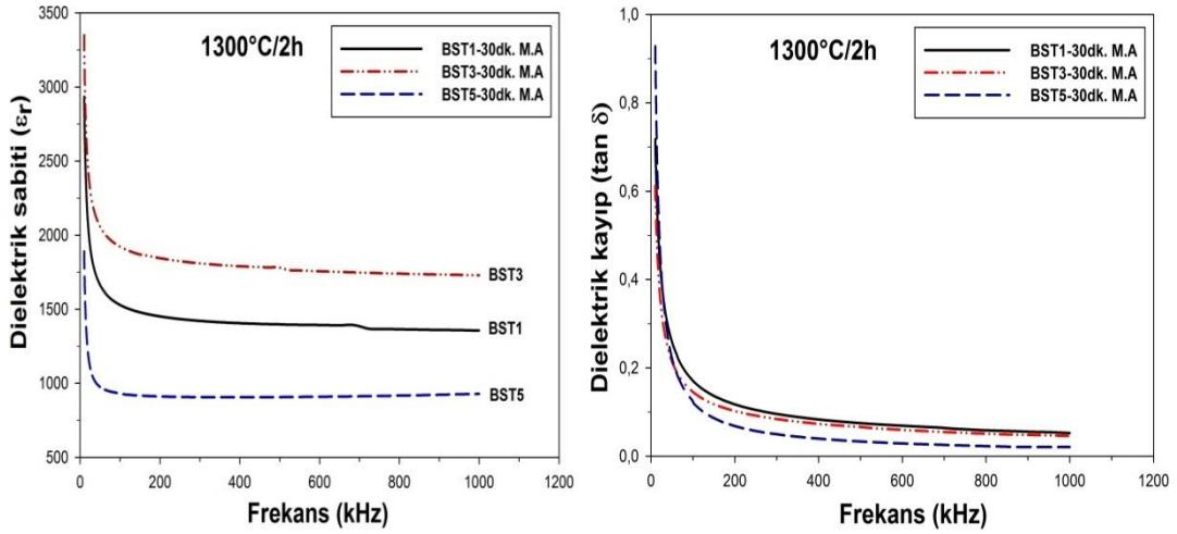
Şekil 5.31. 1300°C’de 2 saat sinterlenen 30dk. mekanik aktive edilmiş BST numunelerinin dielektrik sabiti ( \epsilon_r ) ve dielektrik kayıp ( \tan \delta ) ölçüm grafiği
