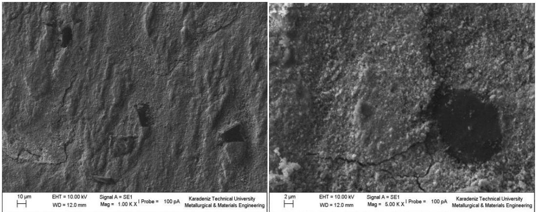
Şekil 3.26. % 10 B 4 C içeren numunenin aşınma yüzeyinin SEM de 1000x ve 5000x görüntüsü
