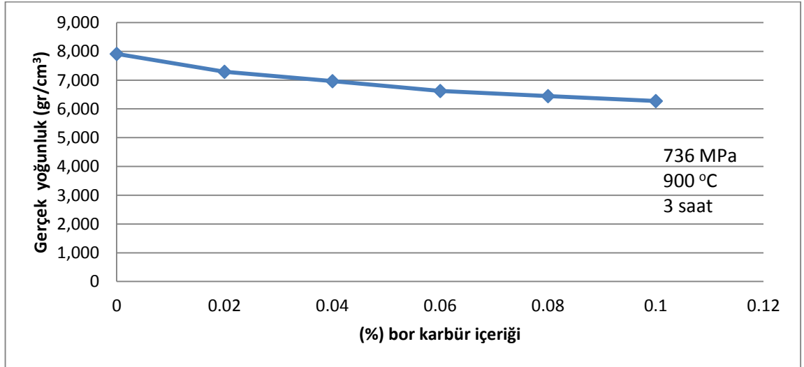
Şekil 3.10.Bor karbürün gerçek yoğunluğa etkisi
