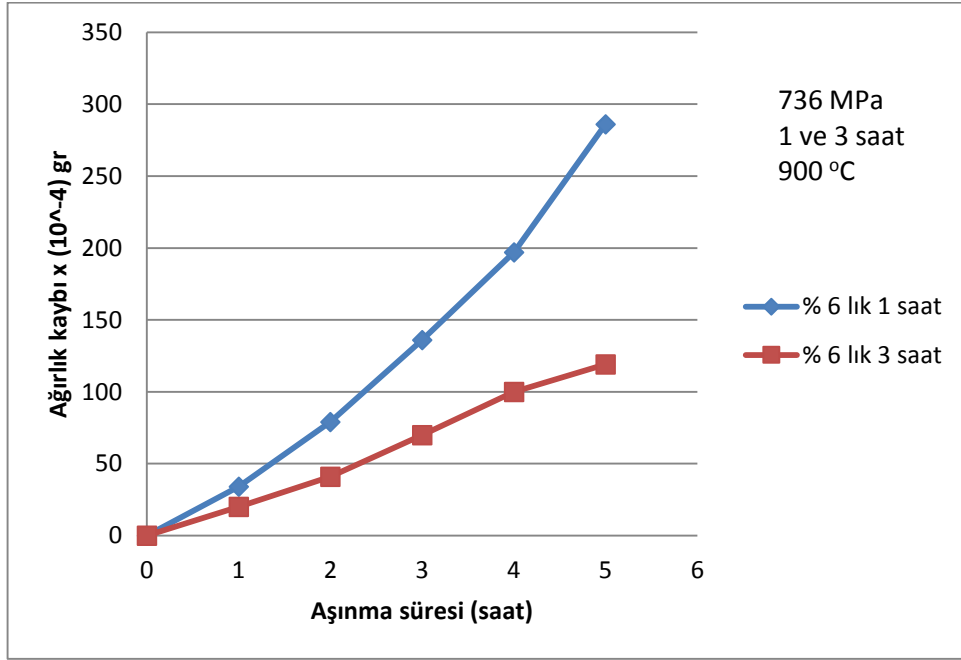
Şekil 3.17.% 6 B 4 C içeren numunelere ait sinterleme süresinin aşınma dayanımına etkisi
